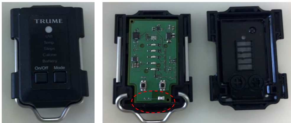
2.4G BLE Antenna
