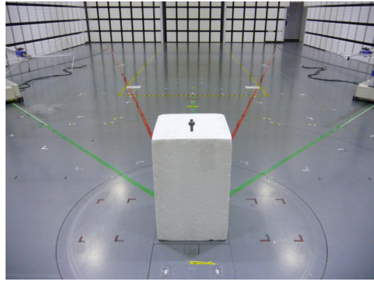
30 - 1000MHz
