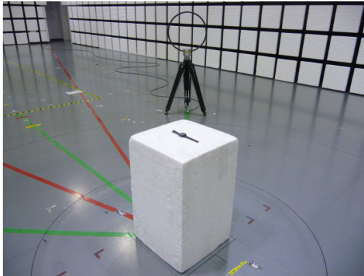
9kHz - 30MHz
