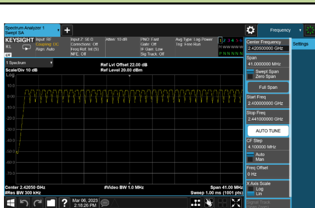
DH5(1Mbps)-2400~2441MHz
