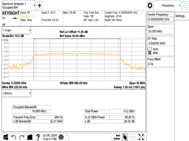
802.11ax_20MHz_Chain1_5320MHz_RU106_54
