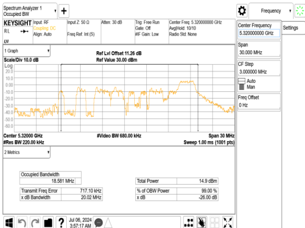
802.11ax_20MHz_Chain1_5320MHz_RU26_8
