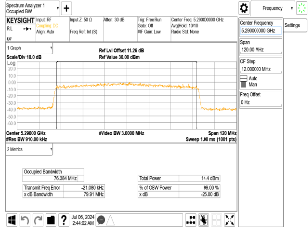
802.11ax_80MHz_Chain0_5290MHz_RU484_66
