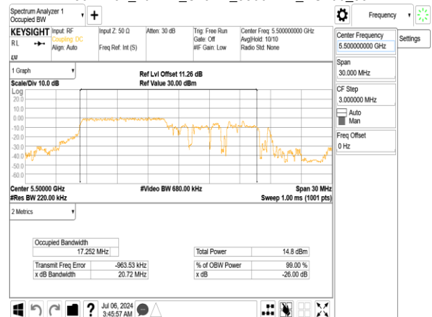
802.11ax_20MHz_Chain1_5500MHz_RU106_53
