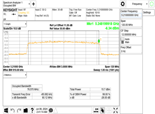
802.11ax_80MHz_Chain1_5210MHz_RU484_65
