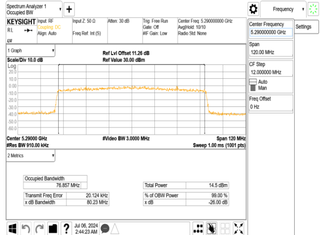
802.11ax_80MHz_Chain1_5290MHz
