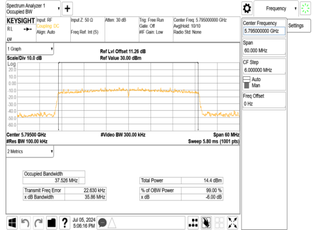
802.11ax_40MHz_Chain1_5795MHz_RU242_62
