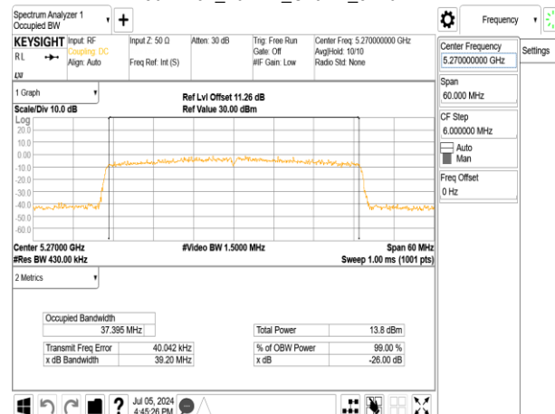
802.11ax_40MHz_Chain1_5270MHz
