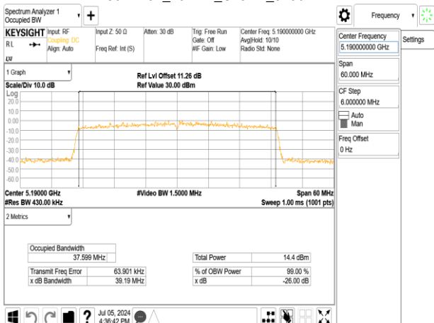
802.11ax_40MHz_Chain1_5190MHz
