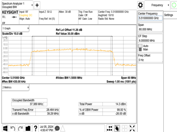
802.11ax_40MHz_Chain0_5510MHz
