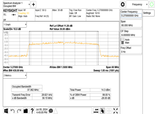
802.11ax_40MHz_Chain0_5270MHz
