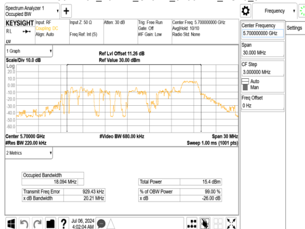
802.11ax_20MHz_Chain1_5700MHz_RU26_8
