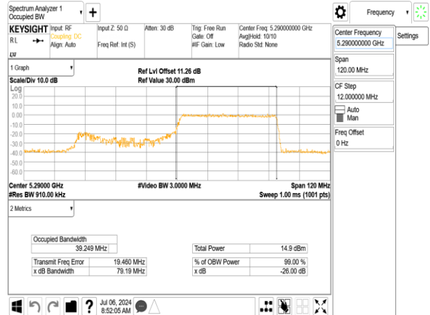
802.11ax_80MHz_Chain0_5290MHz_RU484_66
