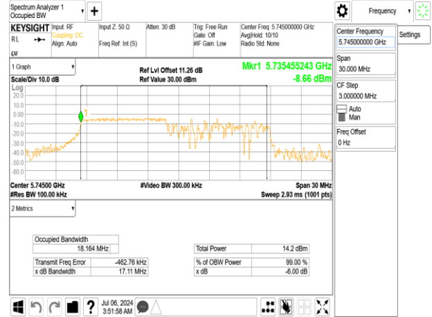
802.11ax_20MHz_Chain1_5745MHz_RU26_0
