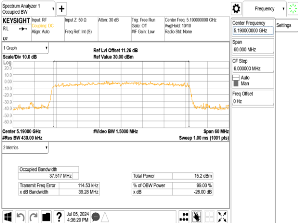
802.11ax_40MHz_Chain0_5190MHz
