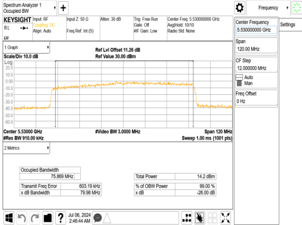
802.11ax_80MHz_Chain0_5530MHz_RU484_65
