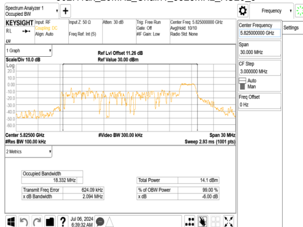
802.11ax_20MHz_Chain1_5825MHz_RU52_40
