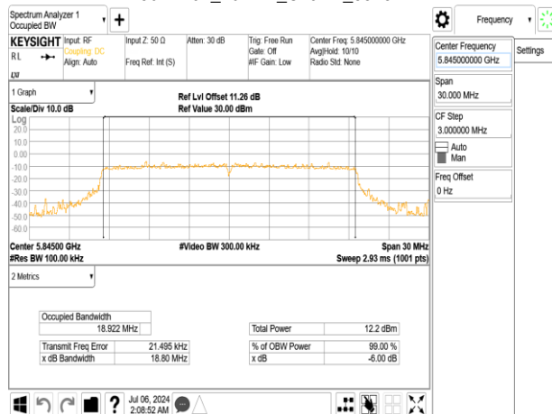
802.11ax_20MHz_Chain1_5845MHz
