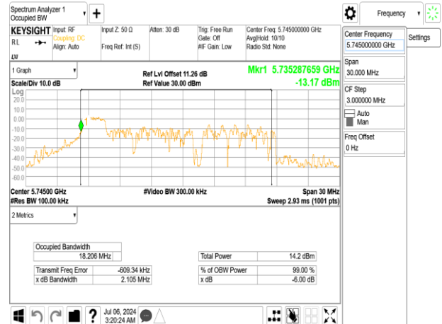
802.11ax_20MHz_Chain1_5745MHz_RU52_37
