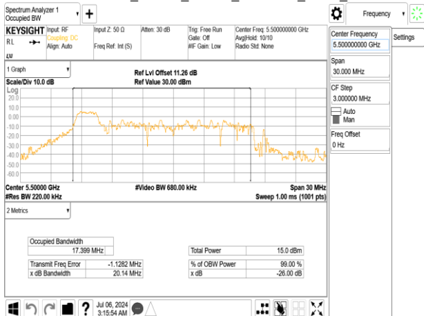
802.11ax_20MHz_Chain1_5500MHz_RU52_37
