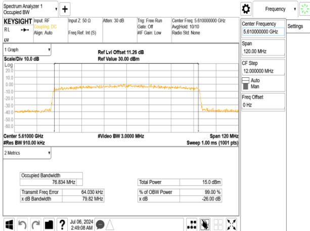
802.11ax_80MHz_Chain0_5610MHz
