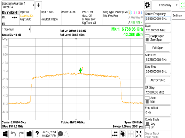
802.11ax_80MHz_Chain1_6785MHz_RU484_66
