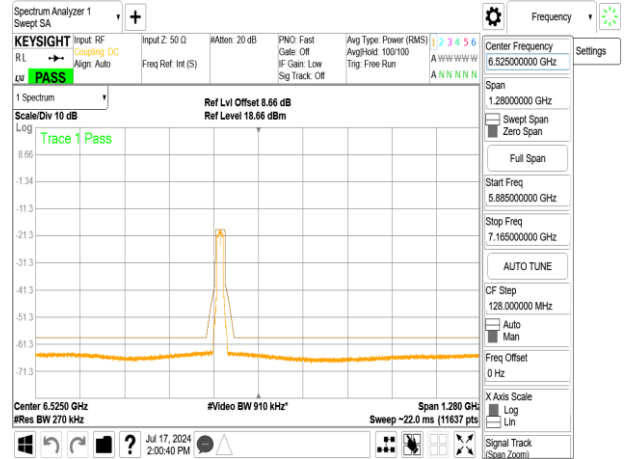
802.11n_20MHz_Chain0_6435MHz
