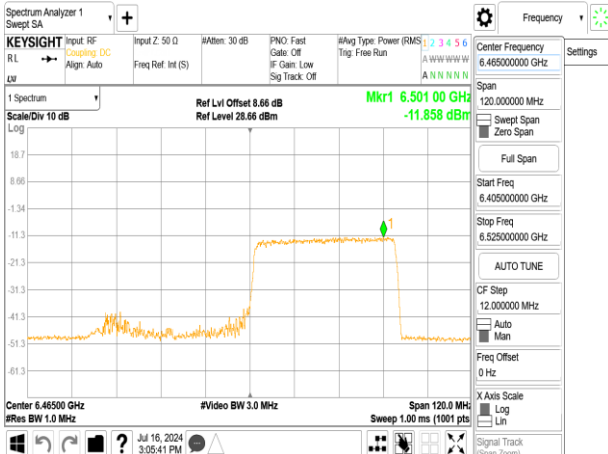
802.11ax_80MHz_Chain1_6465MHz_RU484_66
