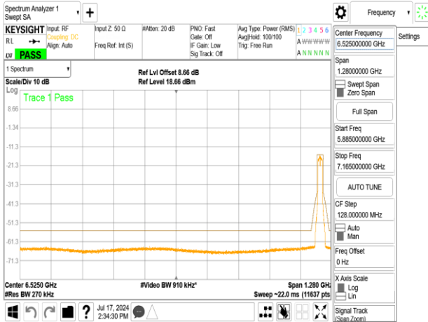
802.11n_20MHz_Chain0_7115MHz
