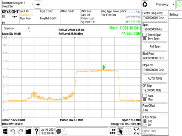
802.11ax_80MHz_Chain1_7025MHz_RU484_66
