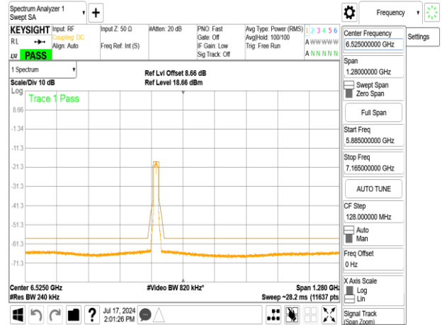
802.11n_20MHz_Chain1_6415MHz
