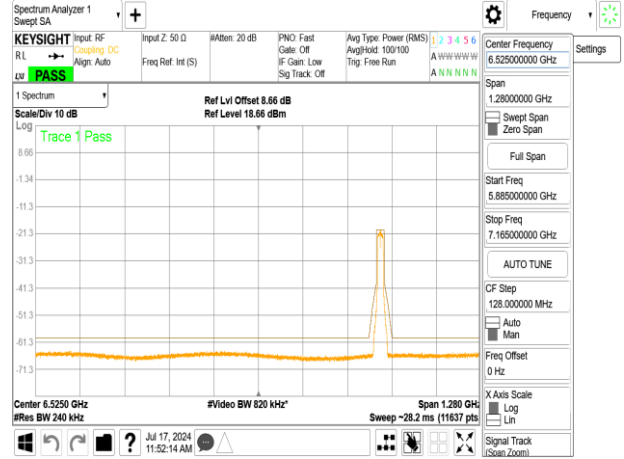
802.11a_20MHz_Chain1_6895MHz
