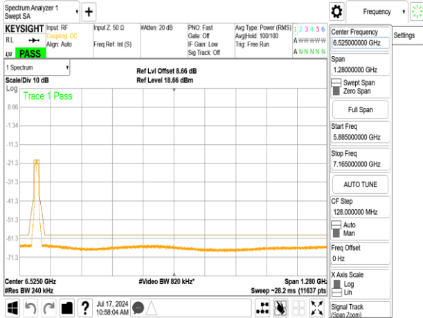
802.11a_20MHz_Chain1_6175MHz
