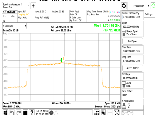
802.11ax_80MHz_Chain0_6705MHz
