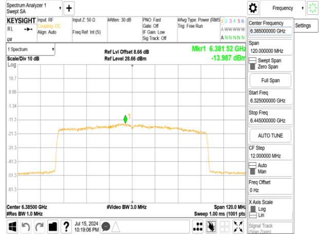
802.11ax_80MHz_Chain0_6385MHz_RU484_66
