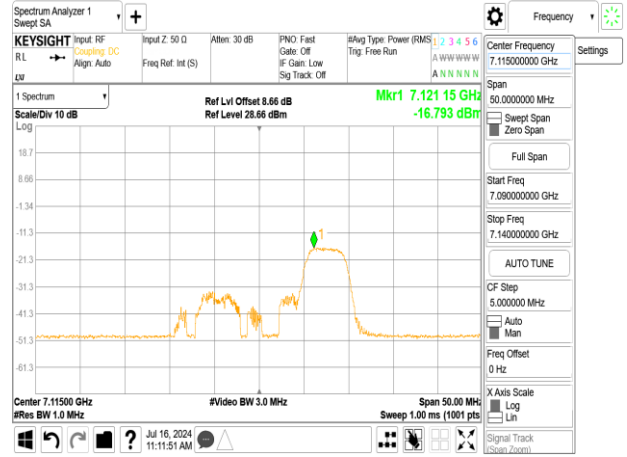
802.11ax_20MHz_Chain1_7115MHz_RU52_40
