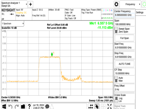
802.11ax_40MHz_Chain1_6565MHz_RU242_61
