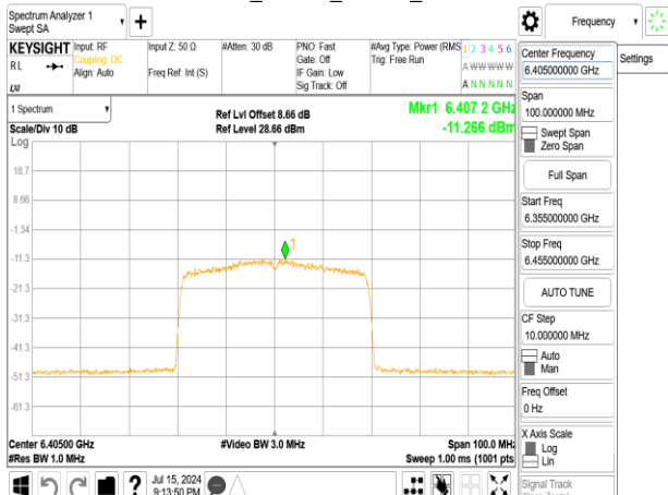
802.11ax_40MHz_Chain1_6405MHz_RU242_62
