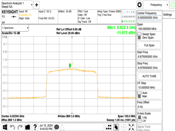
802.11ax_40MHz_Chain1_6925MHz_RU242_61
