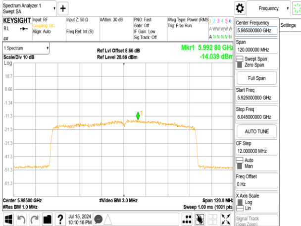
802.11ax_80MHz_Chain1_5985MHz_RU484_65
