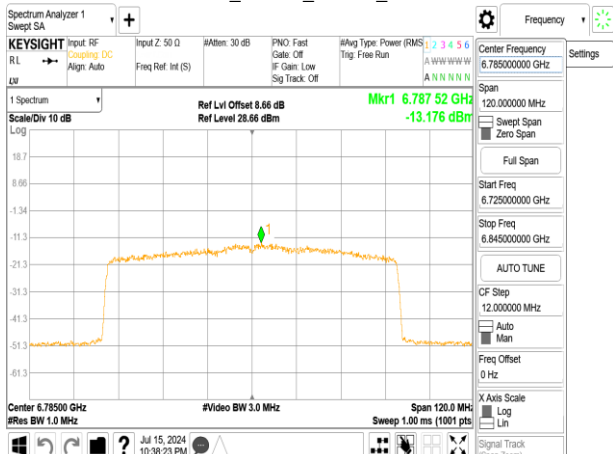
802.11ax_80MHz_Chain0_6785MHz_RU484_66
