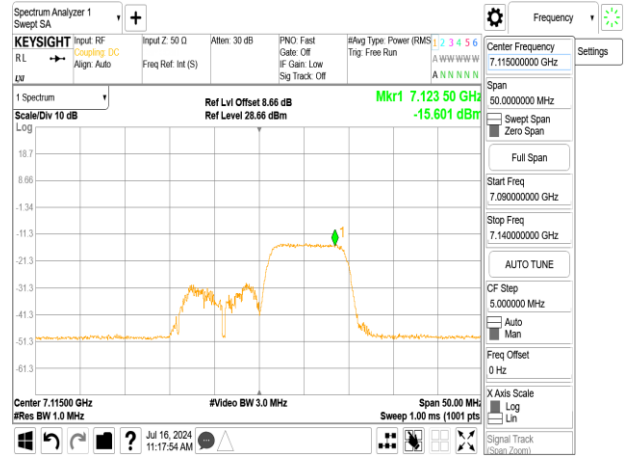
802.11ax_20MHz_Chain1_7115MHz_RU26_8
