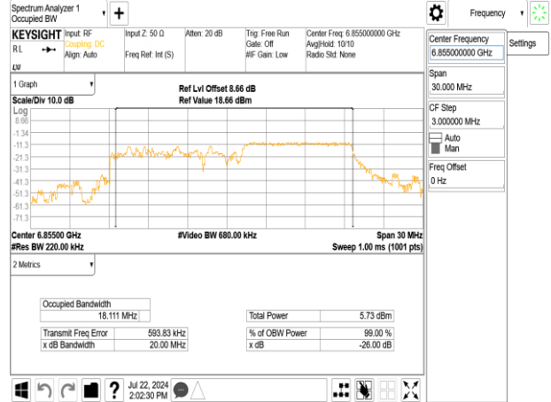
802.11ax_20MHz_Chain0_6855MHz_RU26_8
