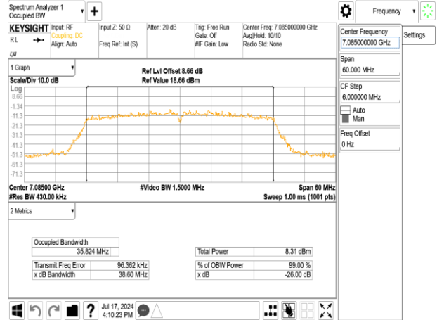
802.11n_40MHz_Chain1_7085MHz
