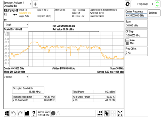
802.11ax_20MHz_Chain0_6435MHz_RU52_37
