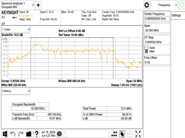
802.11ax_20MHz_Chain1_5955MHz_RU52_37
