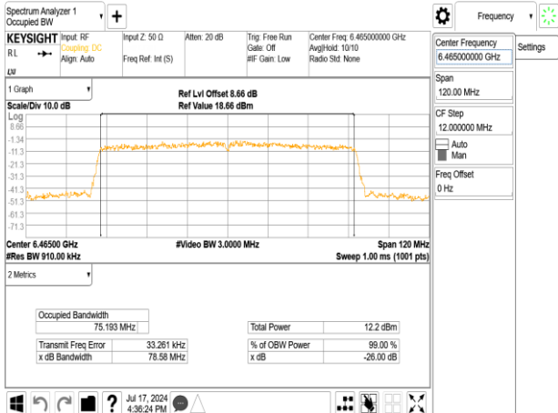
802.11ac_80MHz_Chain1_6465MHz
