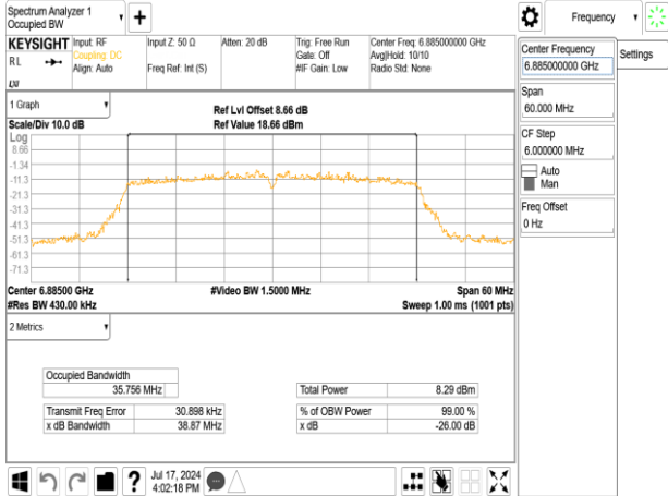
802.11n_40MHz_Chain1_6885MHz
