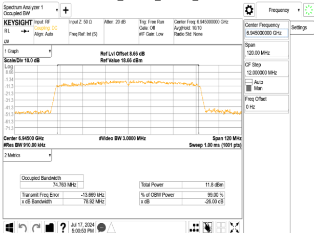
802.11ac_80MHz_Chain1_6945MHz
