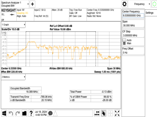
802.11ax_20MHz_Chain0_6535MHz_RU52_37
