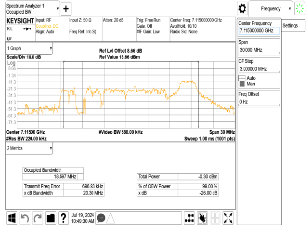
802.11ax_20MHz_Chain0_7115MHz_RU52_40
