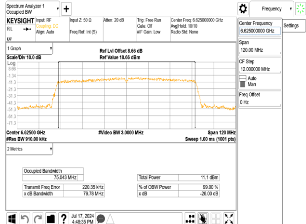
802.11ac_80MHz_Chain0_6625MHz
