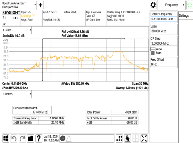
802.11ax_20MHz_Chain1_6415MHz_RU52_40
