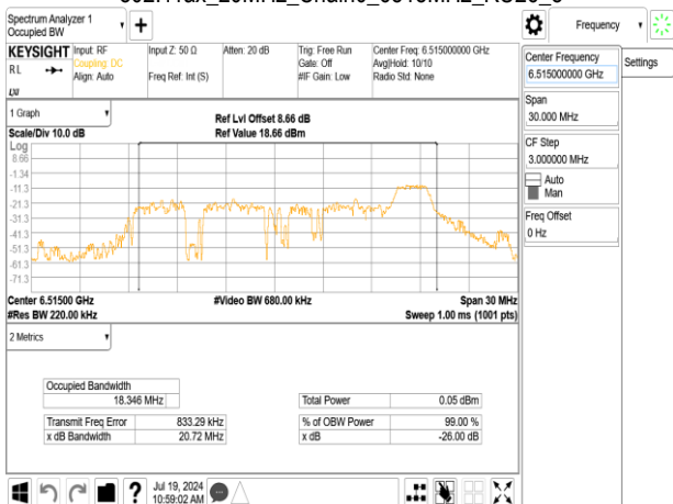
802.11ax_20MHz_Chain0_6515MHz_RU26_8
