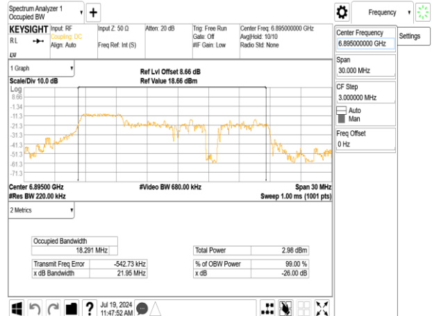
802.11ax_20MHz_Chain0_6895MHz_RU52_37
