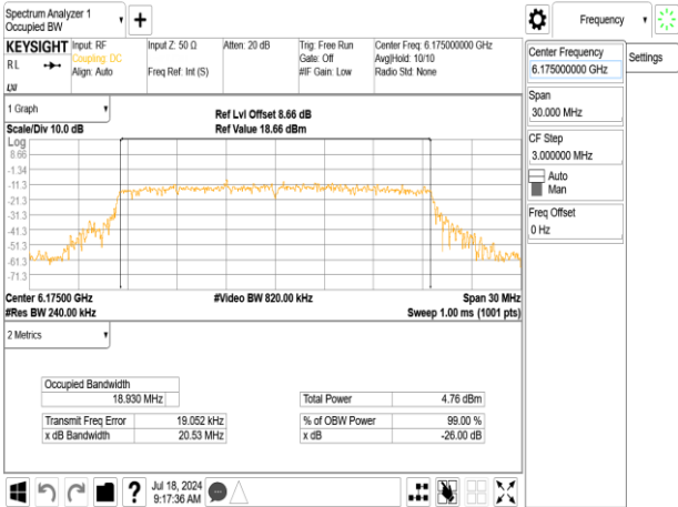
802.11ax_20MHz_Chain0_6175MHz
