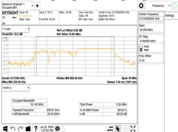
802.11ax_20MHz_Chain0_6515MHz_RU26_8
