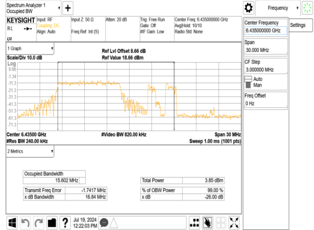
802.11ax_20MHz_Chain1_6435MHz_RU26_0
