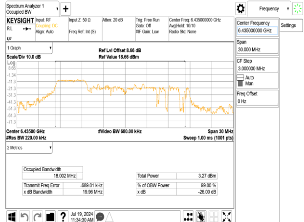
802.11ax_20MHz_Chain1_6435MHz_RU52_37
