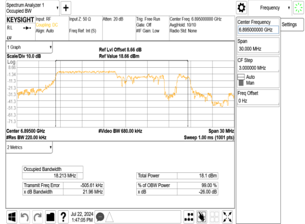
802.11ax_20MHz_Chain0_6895MHz_RU26_0
