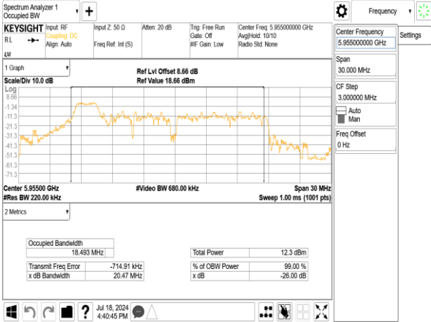
802.11ax_20MHz_Chain0_5955MHz_RU52_37
