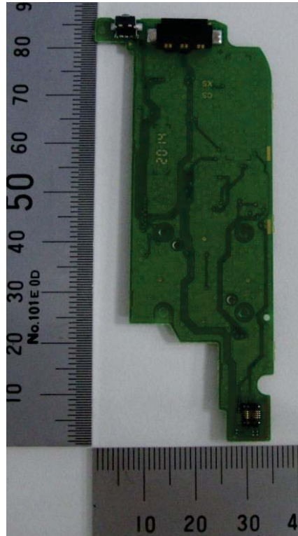
AYS-RED-PCB/ABXY/0X-C0
