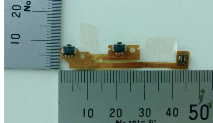
AYS-KTR-FPC/RKEY/*/OX-C0
