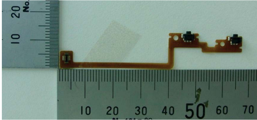
AYS-KTR-FPC/LKEY/*/OX-C0
