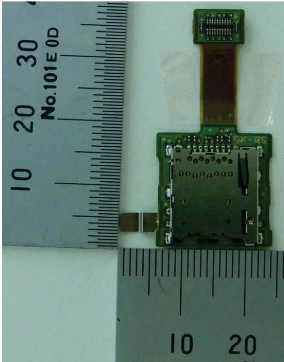
AYS-KTR-RFPCB/SD/0X-C0
