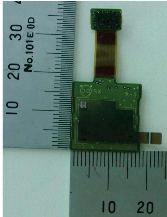
AYS-KTR-RFPCB/SD/0X-C0
