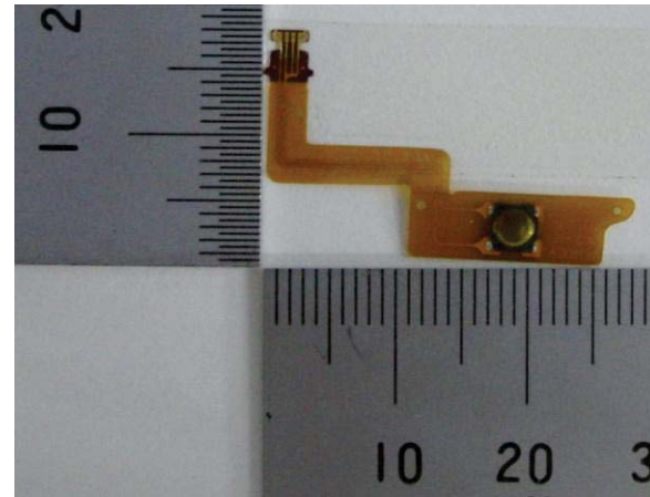
AYS-RED-FPC/HOME/0X-C0
