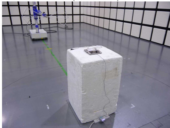
Rear (30-1000MHz)
