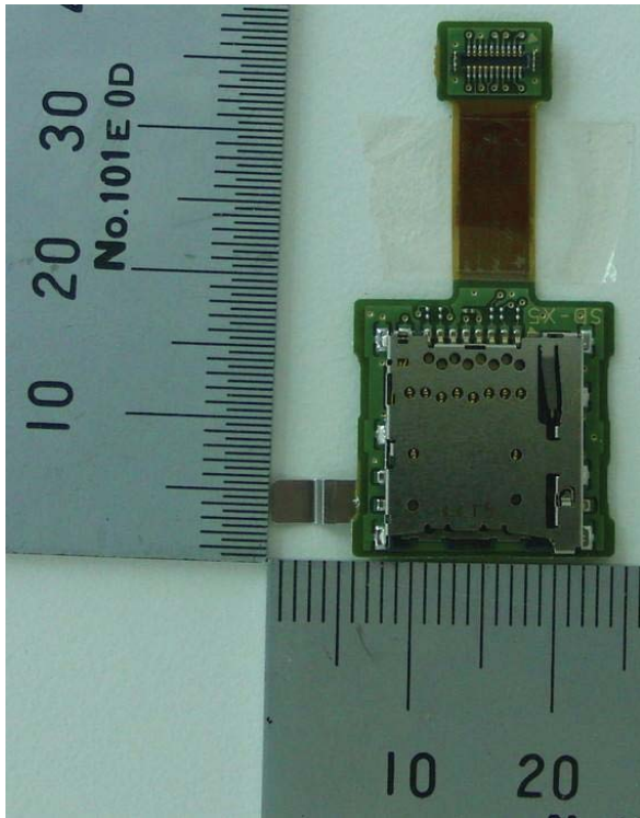
AYS-KTR-RFPCB/SD/0X-C0
