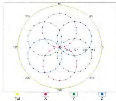
f=1800 MHz,R22
