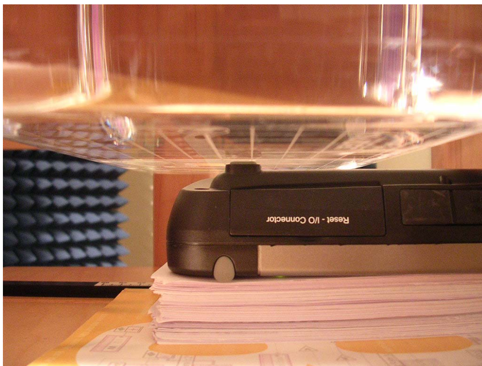
EUT Back
