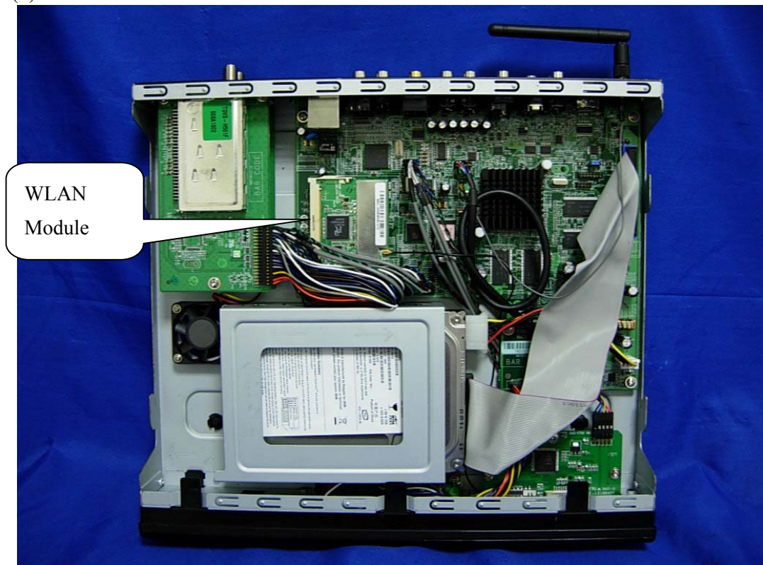
(6) EUT Photo
