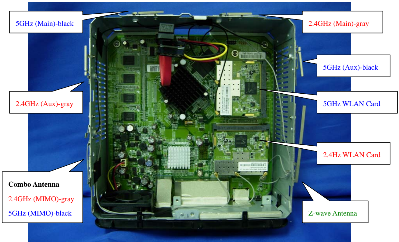
(8) EUT Photo
