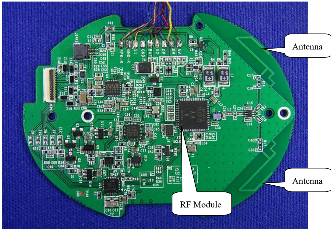
(18) EUT Photo
