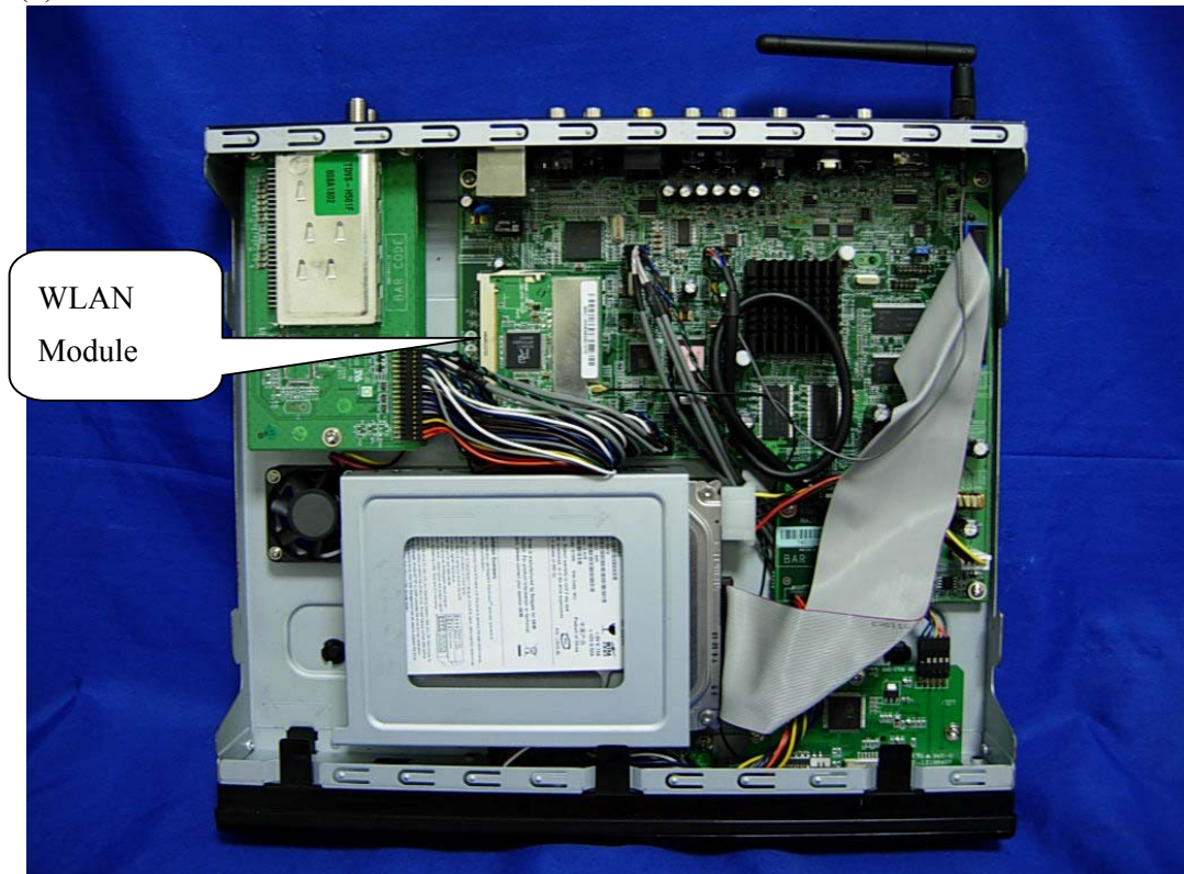
(6) EUT Photo
