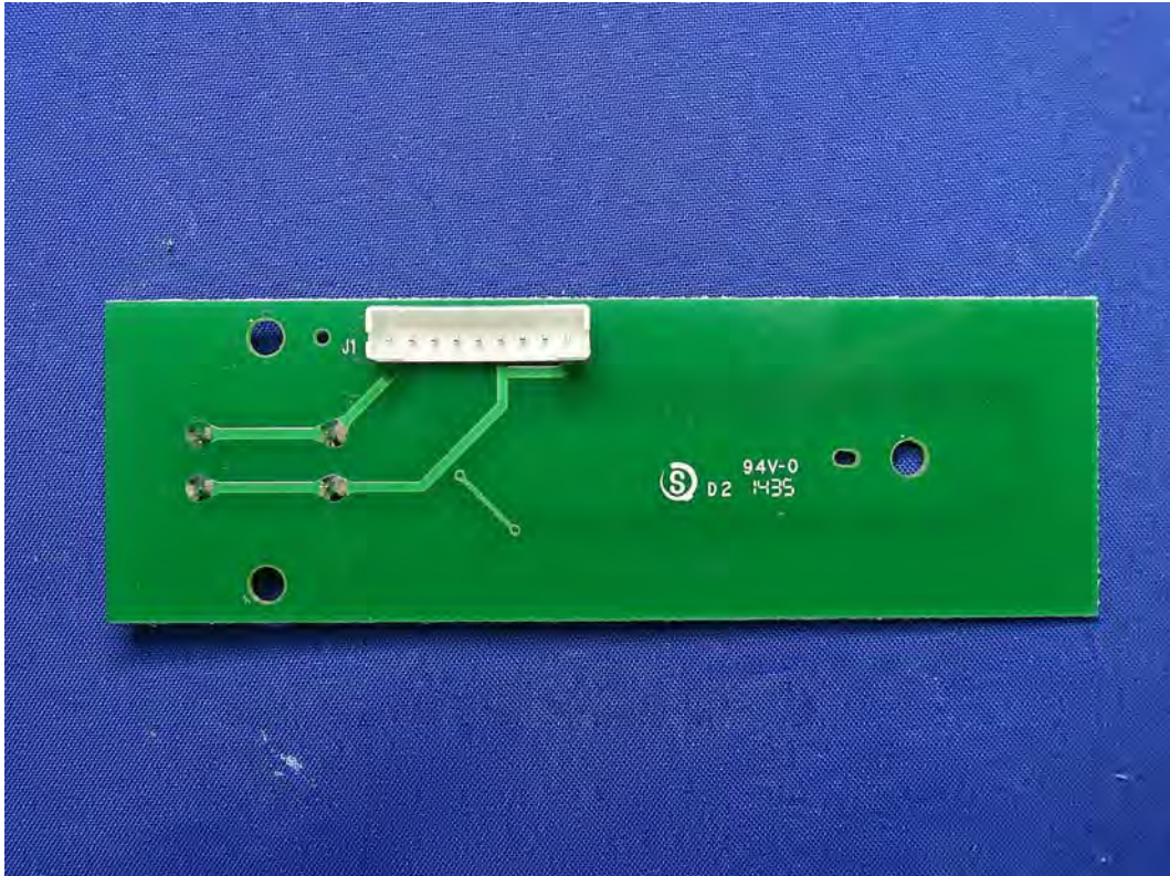
(36) EUT Photo
