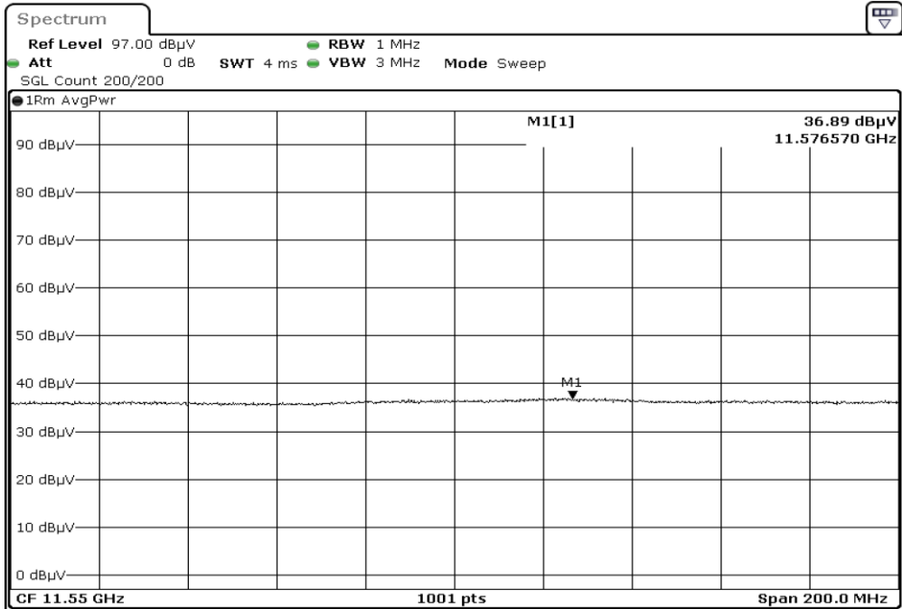
F1 X2 11550.0 Harmonic Vertical AVG
