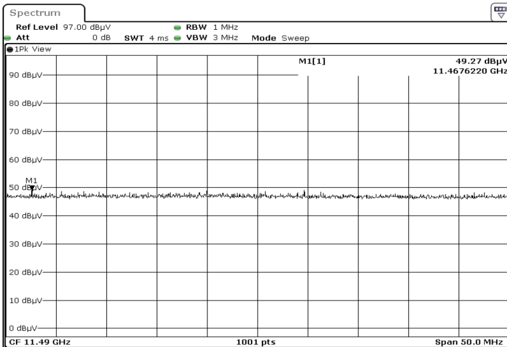
F1 X2 11490.0 Harmonic Horizontal PEAK
