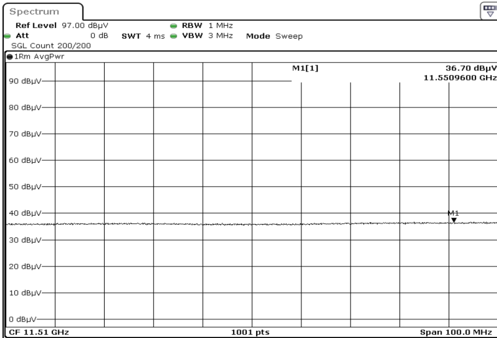
F1 X2 11510.0 Harmonic Horizontal AVG
