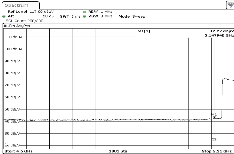
5210.0 F1 RestrictedBand Vertical AVG
