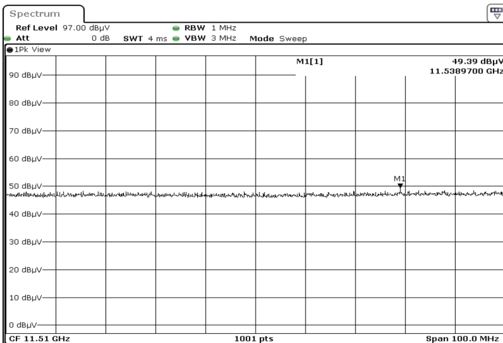
F1 X2 11510.0 Harmonic Vertical PEAK
