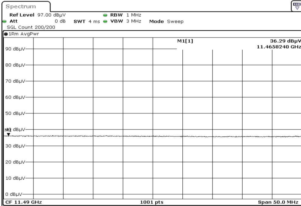
F1 X2 11490.0 Harmonic Horizontal AVG
