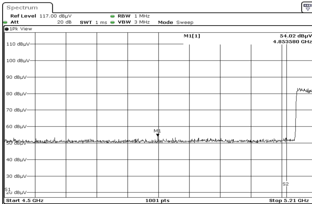
5210.0 F1 RestrictedBand Vertical PEAK
