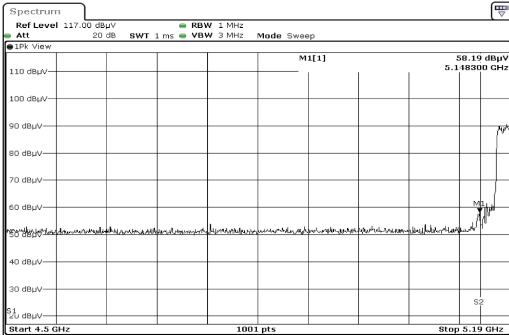
5190.0 F1 RestrictedBand Vertical PEAK
