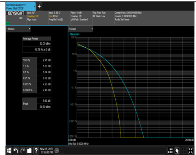
256QAM
