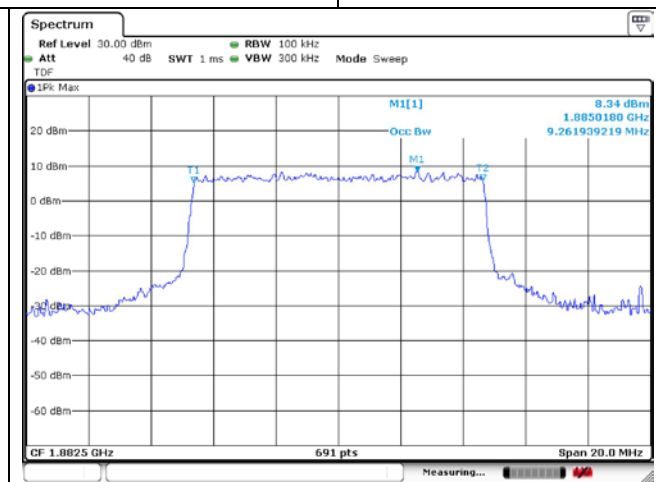
10 MHz CP-OFDM 16QAM
