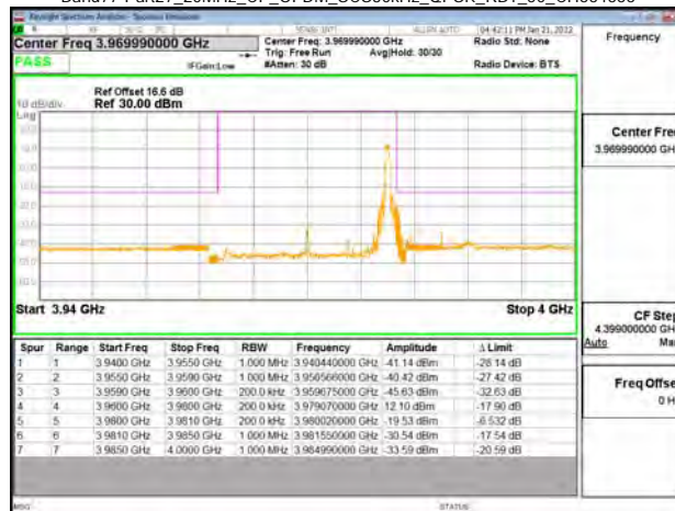
Band77-Part27_20MHz_CP_OFDM_SCS30kHz_QPSK_RB1_50_CH664666
