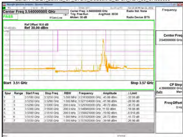
Band77-Part27_20MHz_CP_OFDM_SCS30kHz_QPSK_RB1_50_CH636000
