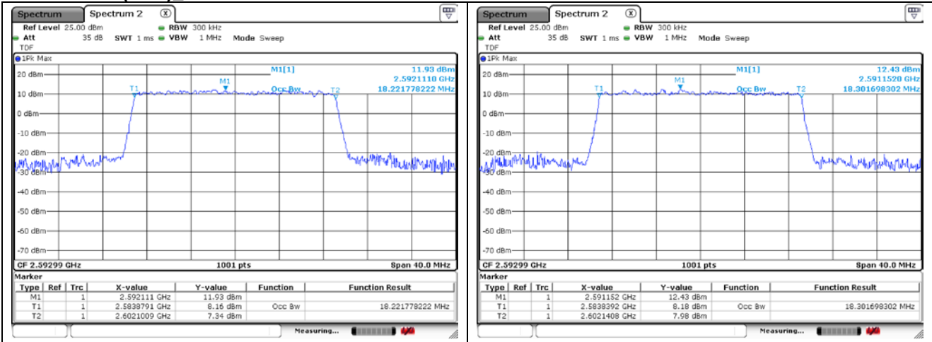
20 MHz CP-OFDM QPSK
