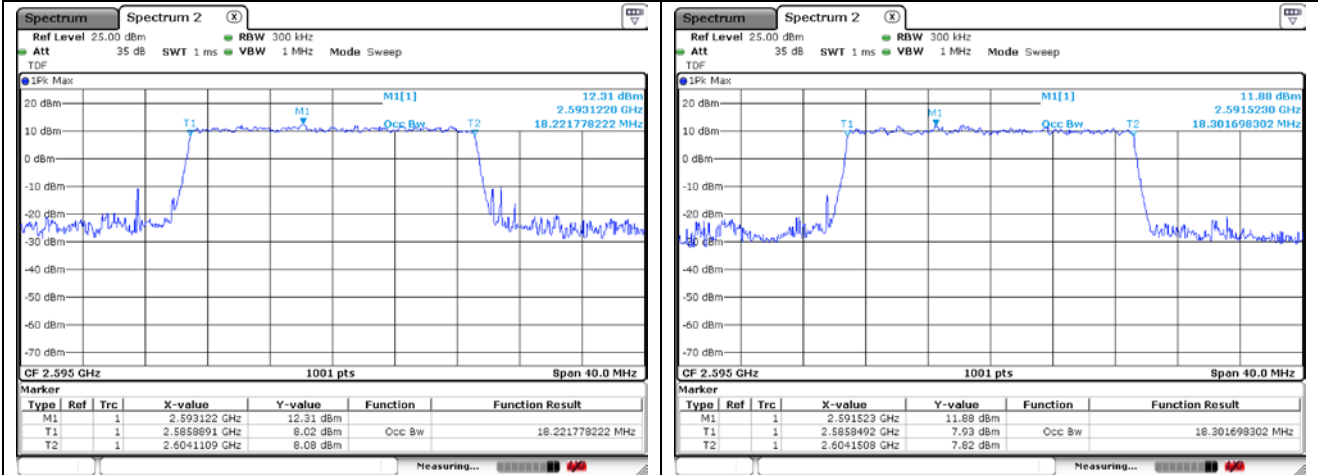
20 MHz CP-OFDM QPSK
