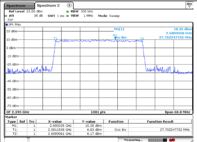
30 MHz CP-OFDM 16QAM
