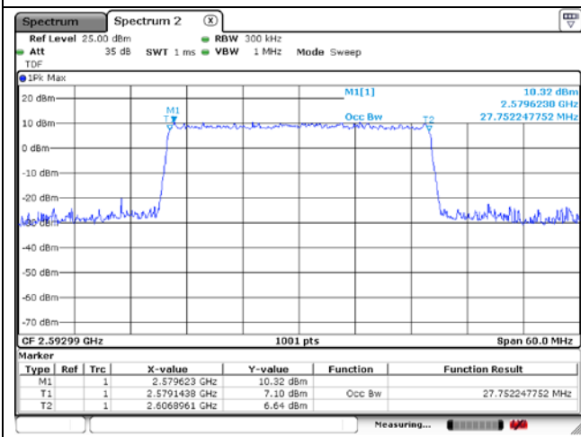
30 MHz CP-OFDM QPSK
