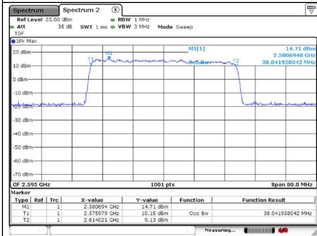
40 MHz CP-OFDM QPSK
