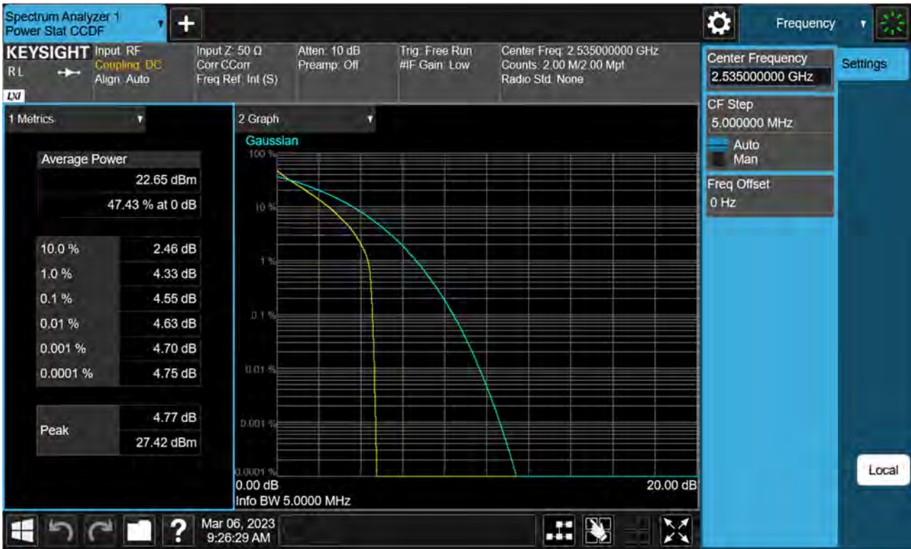
Sub6 n7. PAR Plot (5 M BW_Ch.507000_QPSK)
