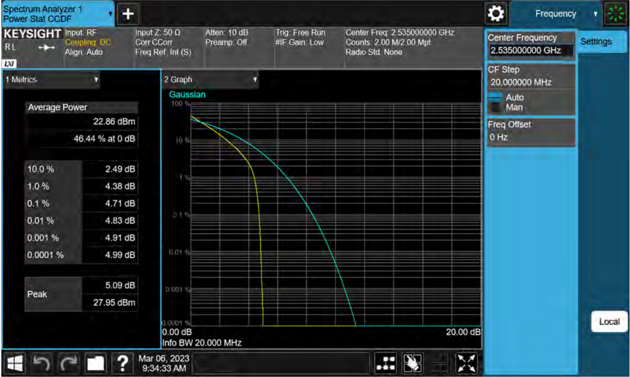
Sub6 n7. PAR Plot (20 M BW_Ch.507000_QPSK)
