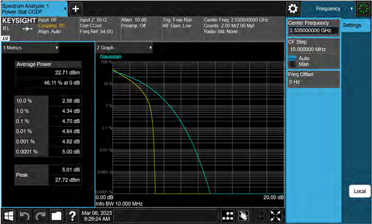
Sub6 n7. PAR Plot (10 M BW_Ch.507000_QPSK)
