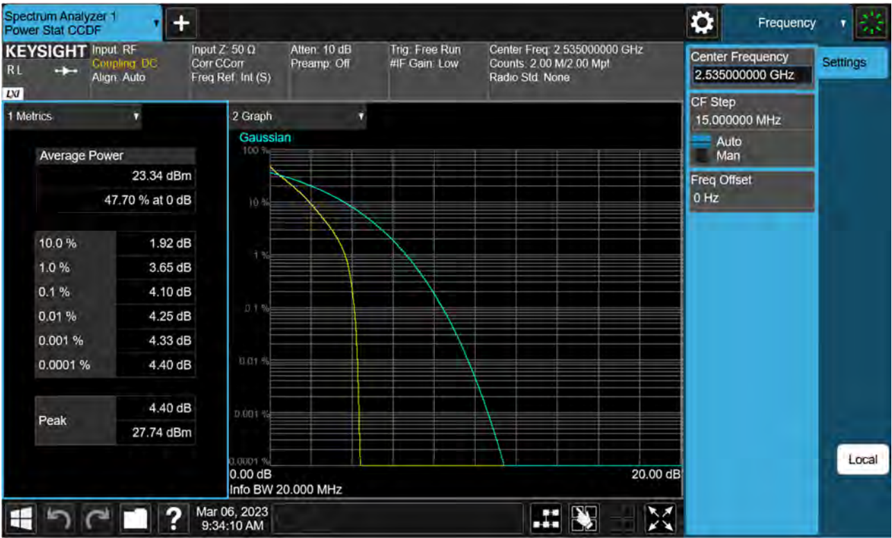
Sub6 n7. PAR Plot (20 M BW_Ch.507000_ BPSK)
