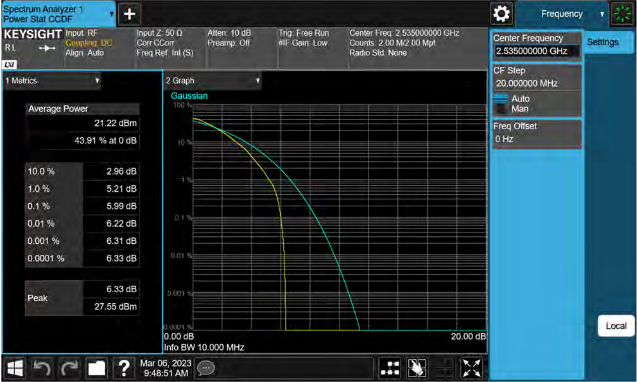
Sub6 n7. PAR Plot (10 M BW_Ch.507000_64QAM)
