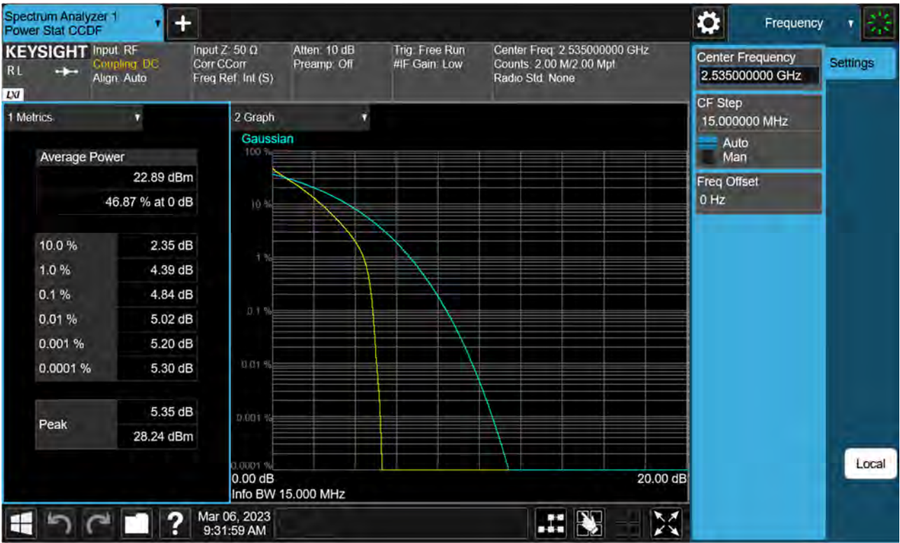
Sub6 n7. PAR Plot (15 M BW_Ch.507000_QPSK)
