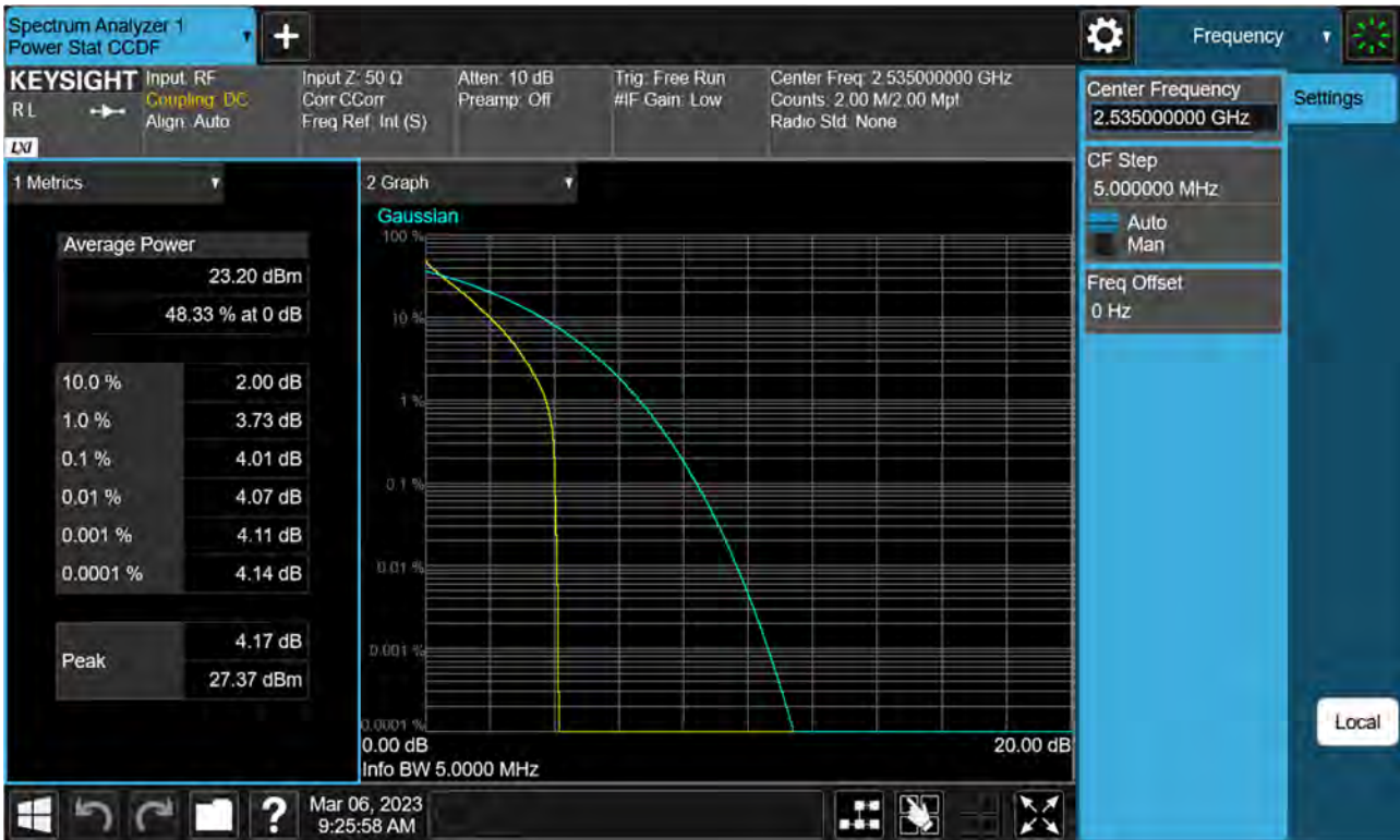
Sub6 n7. PAR Plot (5 M BW_Ch.507000_ BPSK)
