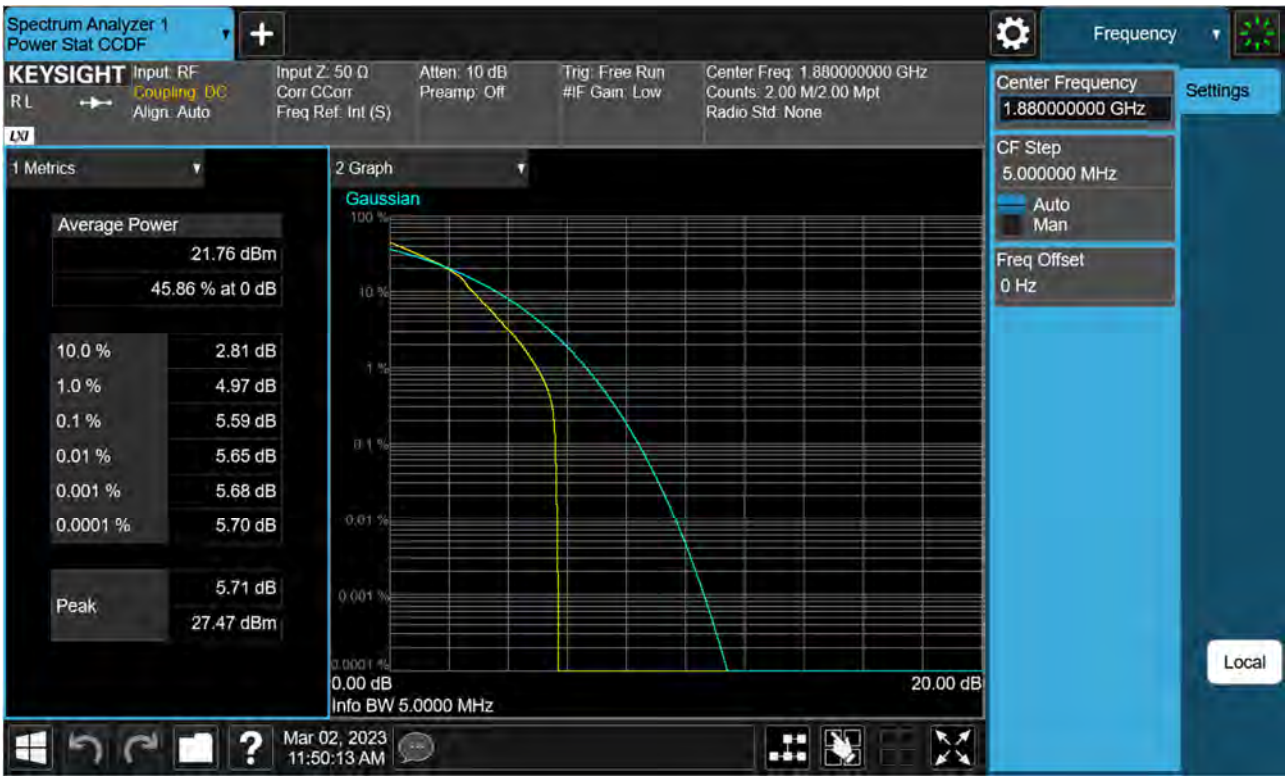
Sub6 n2. PAR Plot (5 M BW Ch.376000 16QAM RB 25_0)
