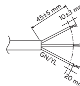
<Guide de retrait de la gaine>
