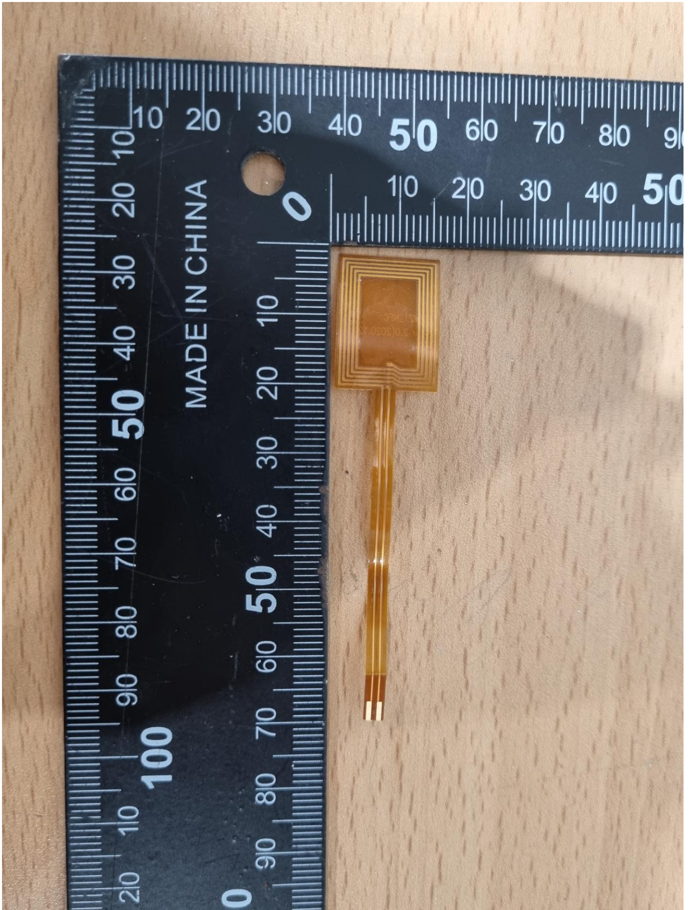
Rear NFC Antenna
