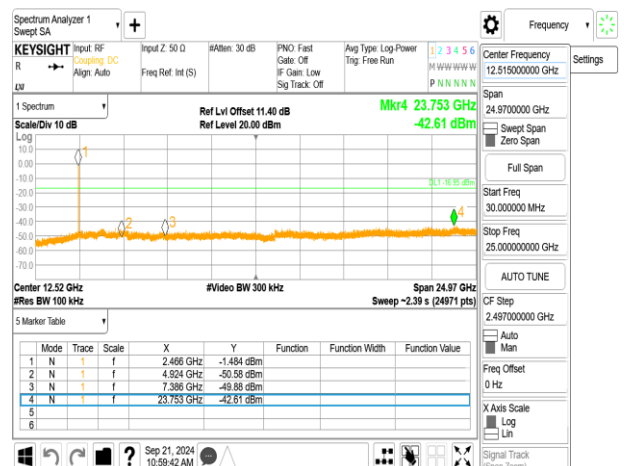
802.11be_20MHz_ChainA_2462MHz
