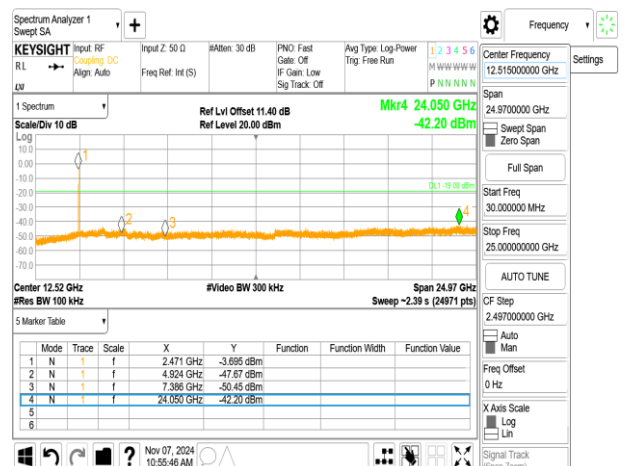
802.11ax_20MHz_ChainB_2462MHz_RU26_8
