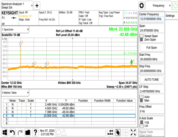
802.11be_20MHz_ChainA_2462MHz_52+26_MRU3
