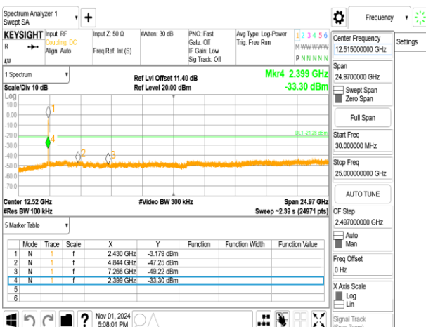
802.11ax_40MHz_ChainB_2422MHz
