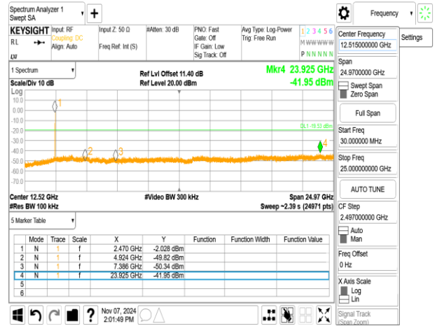
802.11be_20MHz_ChainA_2462MHz_RU52_40
