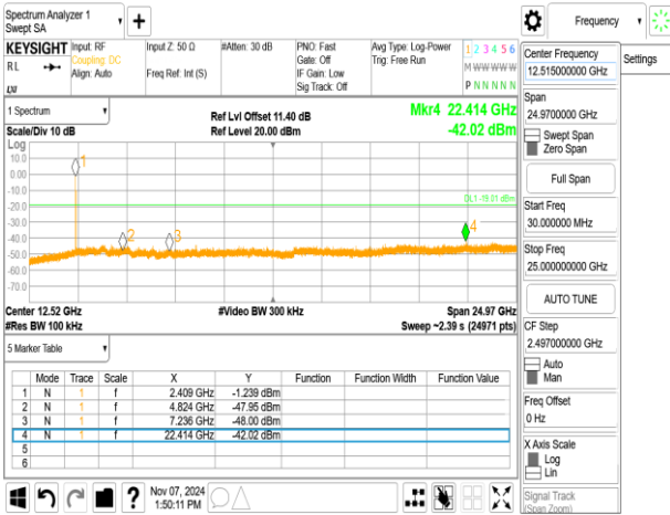
802.11be_20MHz_ChainA_2412MHz_RU106_53
