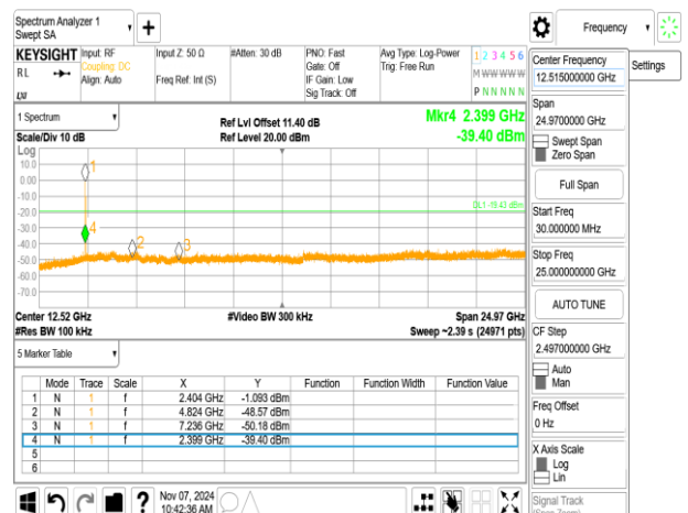
802.11ax_20MHz_ChainA_2412MHz_RU52_37
