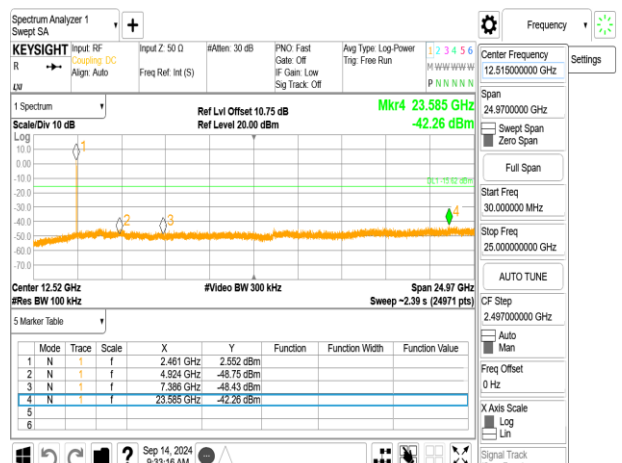
802.11b_20MHz_ChainA_2462MHz
