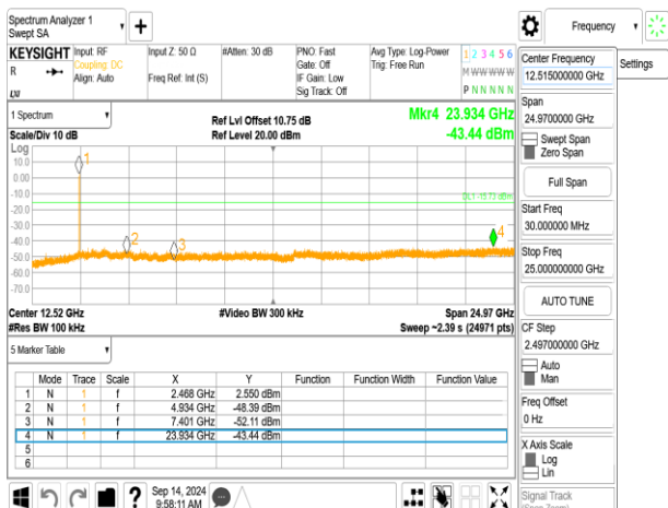
802.11b_20MHz_ChainB_2472MHz
