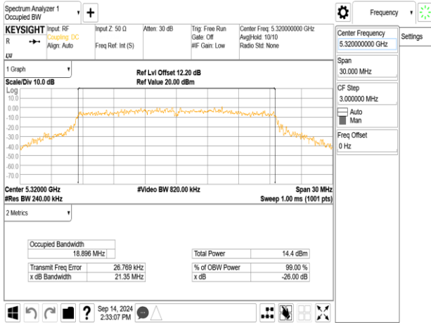
802.11be_20MHz_ChainA_5320MHz_106+26_MRU2
