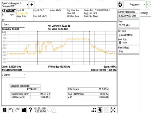
802.11be_20MHz_ChainA_5320MHz_52+26_MRU3
