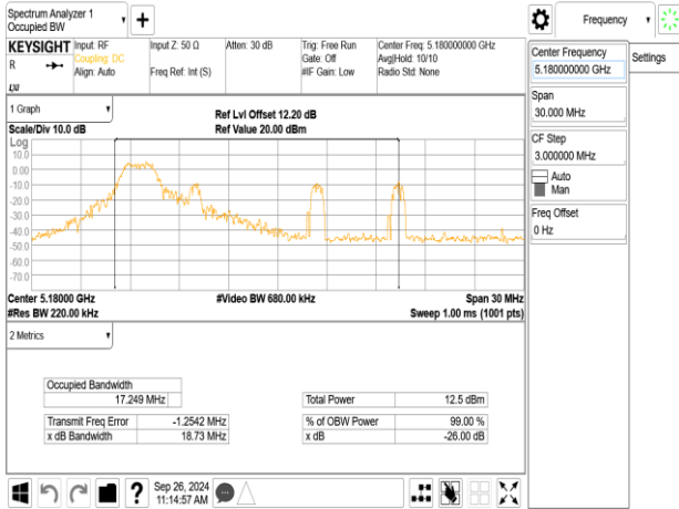
802.11be_20MHz_ChainA_5180MHz_RU52_37
