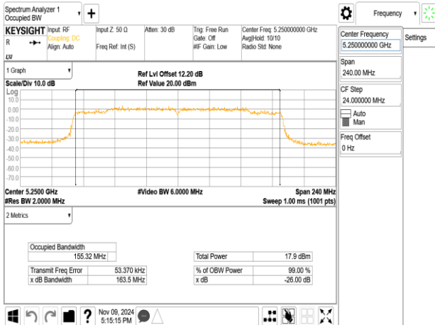
802.11ax_160MHz_ChainB_5250MHz_RU996_67
