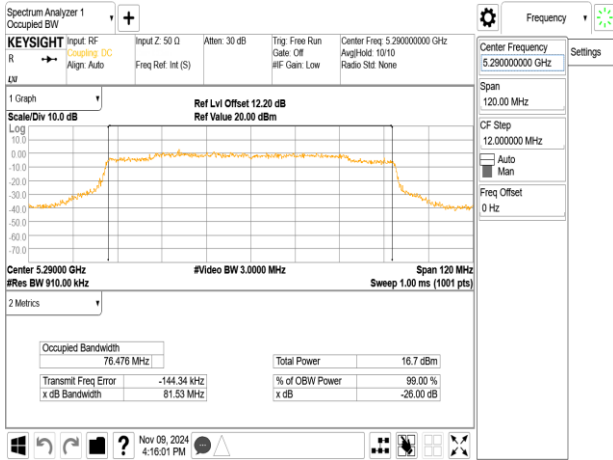
802.11ax_80MHz_ChainA_5290MHz_RU484_66
