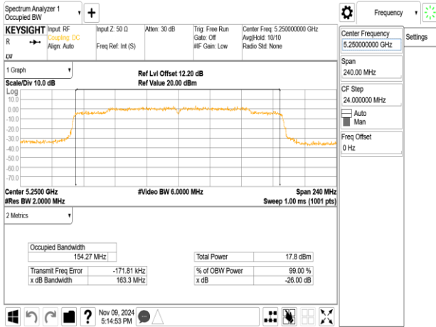
802.11ax_160MHz_ChainA_5250MHz_RU996_67
