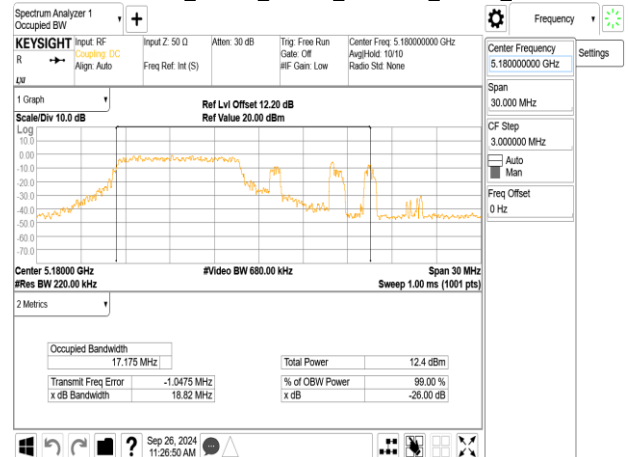
802.11be_20MHz_ChainA_5180MHz_RU106_53
