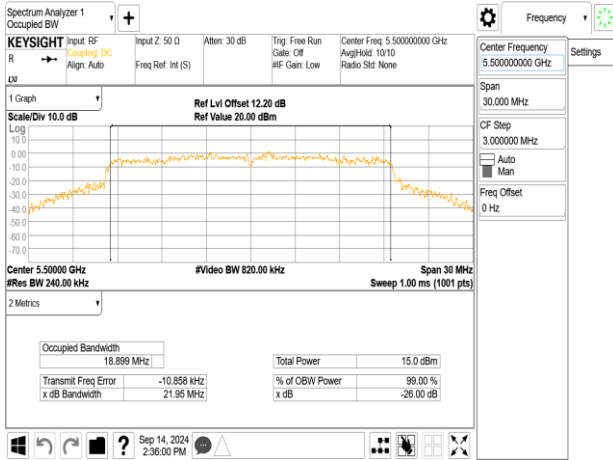
802.11be_20MHz_ChainA_5500MHz_106+26_MRUI
