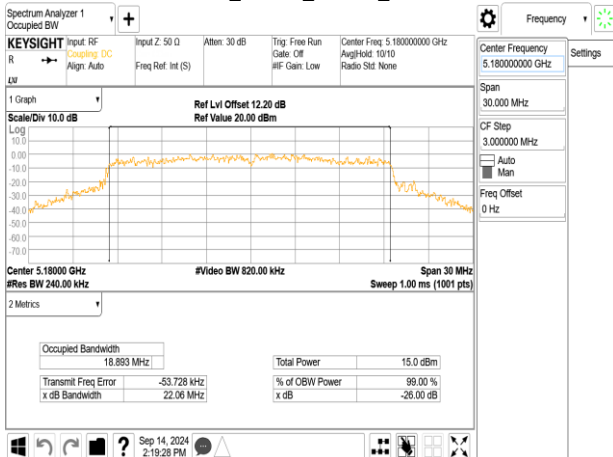
802.11be_20MHz_ChainA_5180MHz
