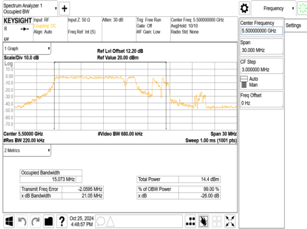
802.11be_20MHz_ChainA_5500MHz_52+26_MRUI
