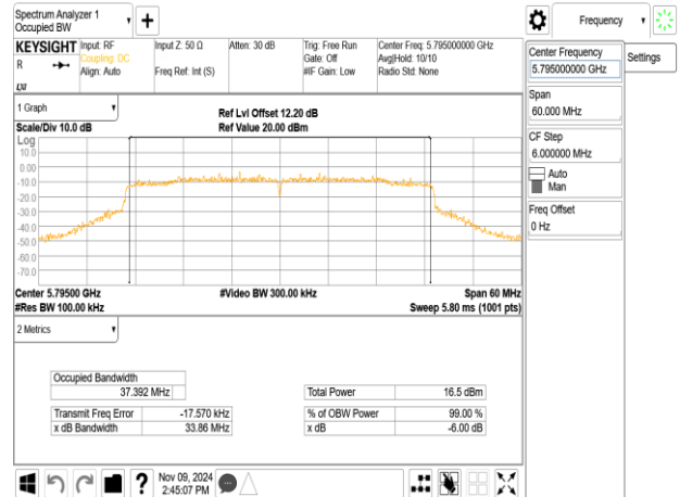
802.11ax_40MHz_ChainB_5795MHz_RU242_62
