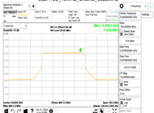
802.11be_40MHz_ChainB_6925MHz
