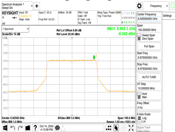
802.11be_40MHz_ChainA_6925MHz
