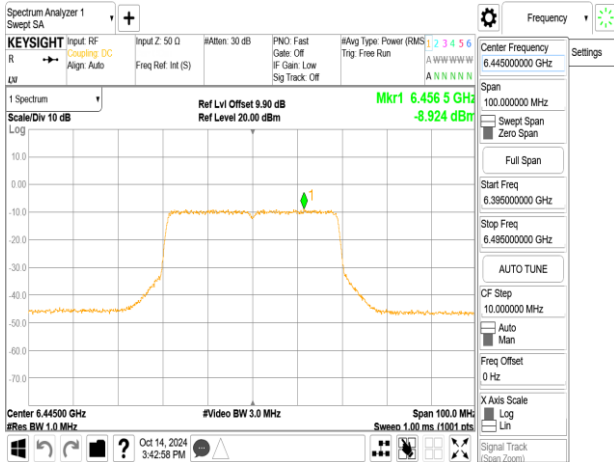
802.11be_40MHz_ChainB_6445MHz_RU242_61
