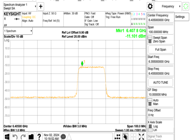
802.11be_40MHz_ChainB_6405MHz_RU242_62
