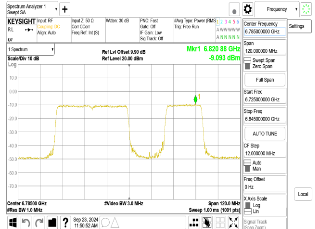
802.11be_80MHz_ChainA_6785MHz_RU484_66
