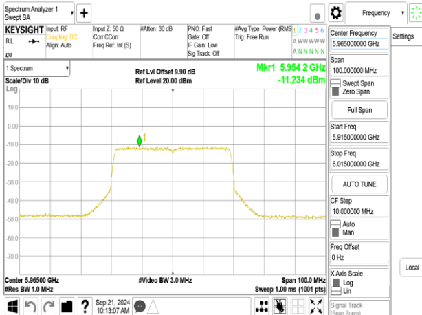
802.11be_40MHz_ChainB_5965MHz_RU242_61
