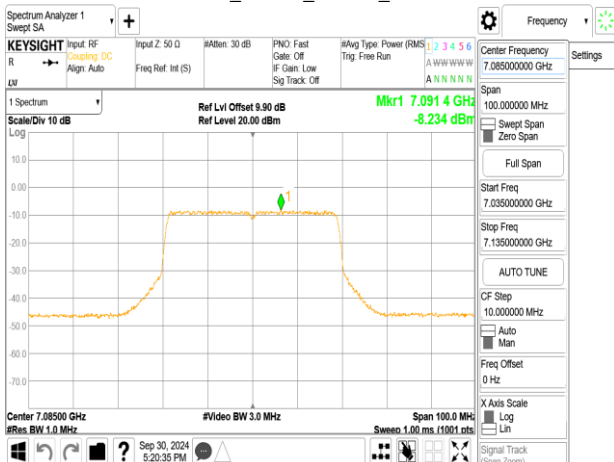
802.11be_40MHz_ChainB_7085MHz
