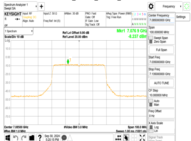
802.11be_40MHz_ChainA_7085MHz
