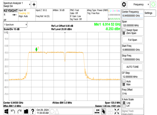
802.11be_80MHz_ChainA_6945MHz_RU484_65
