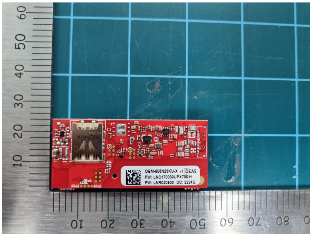
<RFID Module – Rear>
