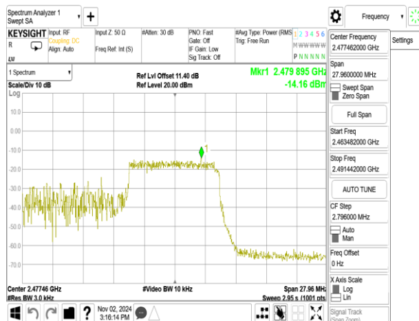
802.11ax_20MHz_ChainB_2472MHz_RU26_8
