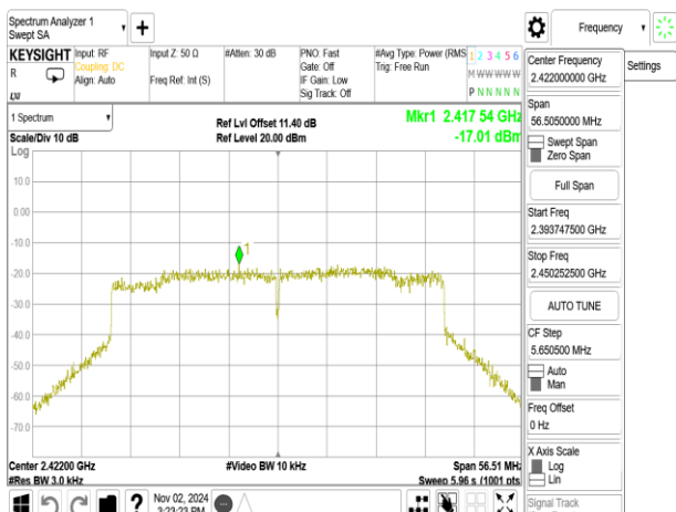
802.11ax_40MHz_ChainB_2422MHz
