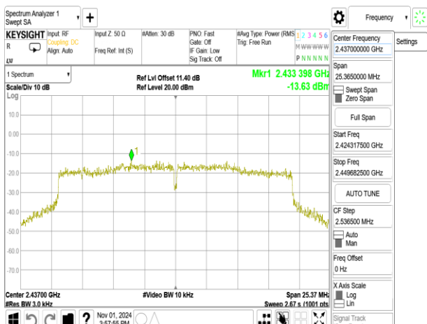
802.11ax_20MHz_ChainB_2437MHz
