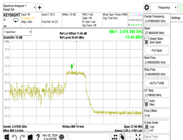
802.11ax_20MHz_ChainB_2472MHz_RU52_40
