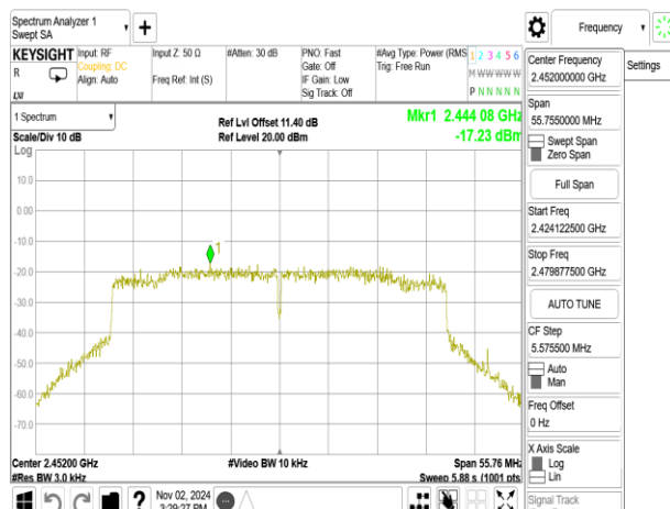
802.11ax_40MHz_ChainB_2452MHz
