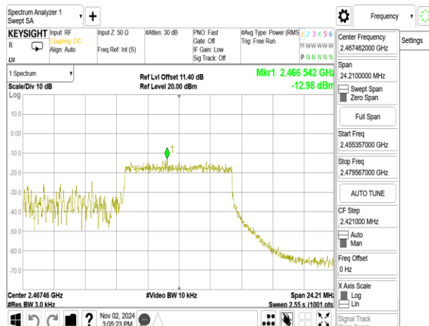
802.11ax_20MHz_ChainB_2462MHz_RU26_8
