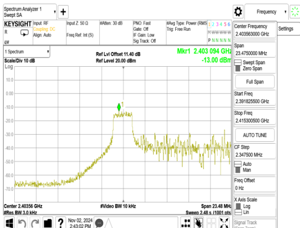
802.11ax_20MHz_ChainB_2412MHz_RU52_37
