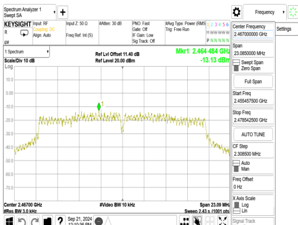
802.11n_20MHz_ChainB_2467MHz
