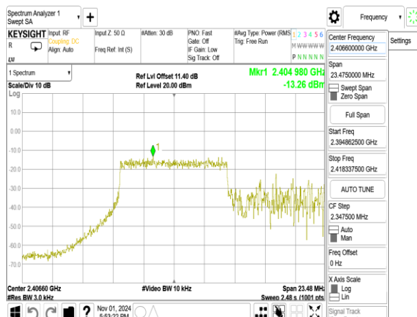
802.11ax_20MHz_ChainB_2412MHz_RU106_53
