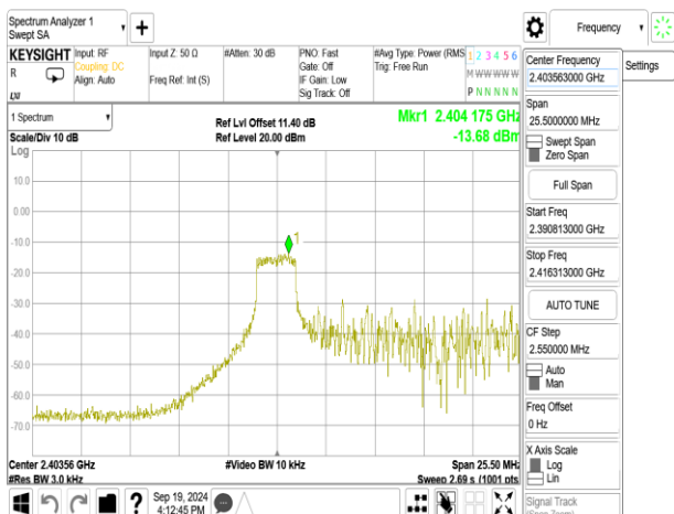
802.11be_20MHz_ChainA_2412MHz_RU26_0
