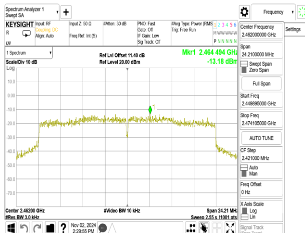
802.11ax_20MHz_ChainB_2462MHz_RU106_54
