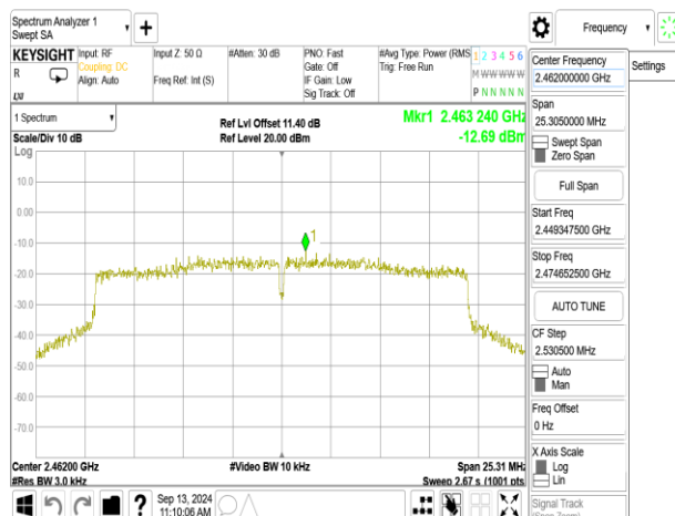
802.11be_20MHz_ChainA_2462MHz
