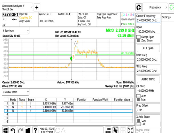
802.11be_20MHz_ChainB_2412MHz_RU52_37
