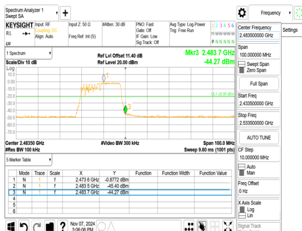
802.11be_20MHz_ChainA_2472MHz_52+26_MRU3
