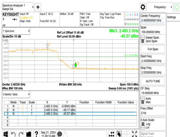
802.11be_40MHz_ChainA_2452MHz_RU242_62
