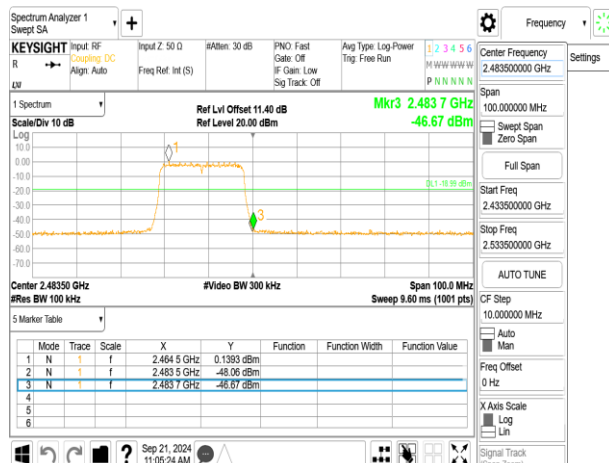
802.11be_20MHz_ChainB_2472MHz_106+26_MRU2
