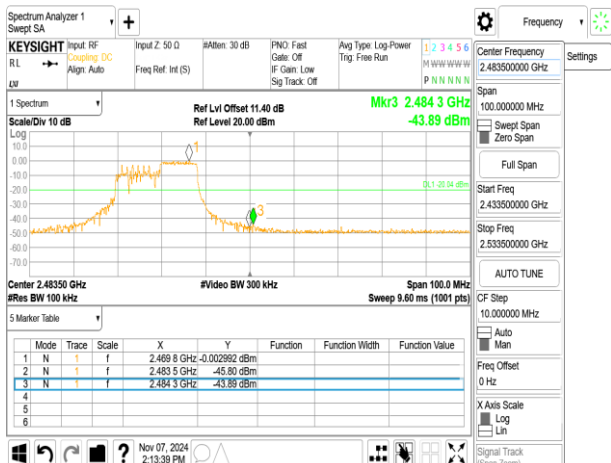
802.11be_20MHz_ChainB_2462MHz_RU26_8
