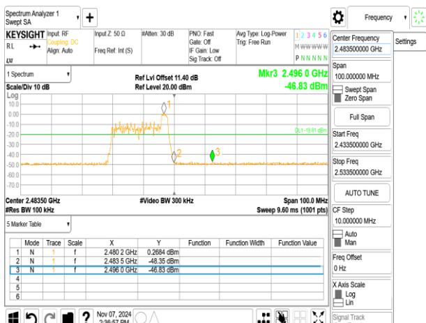
802.11be_20MHz_ChainB_2472MHz_RU26_8
