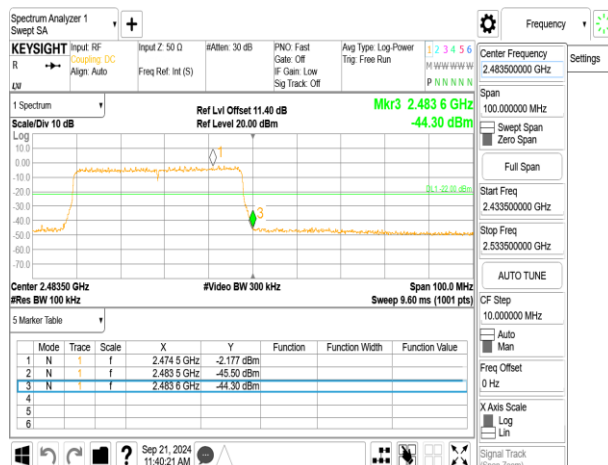
802.11be_40MHz_ChainA_2462MHz_RU242_62
