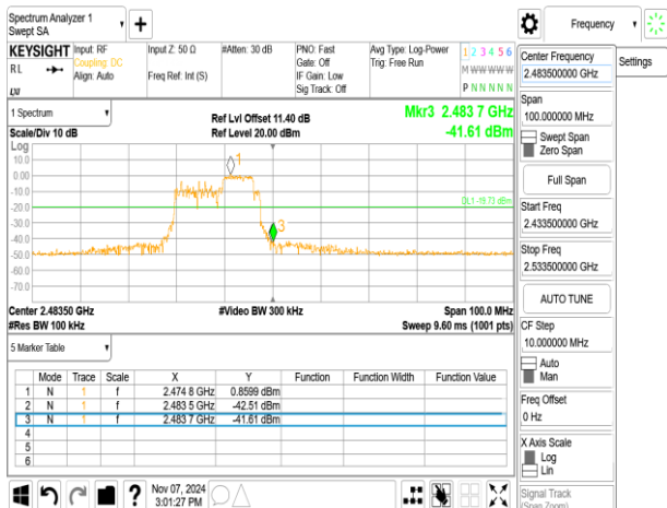
802.11be_20MHz_ChainB_2472MHz_RU106_54
