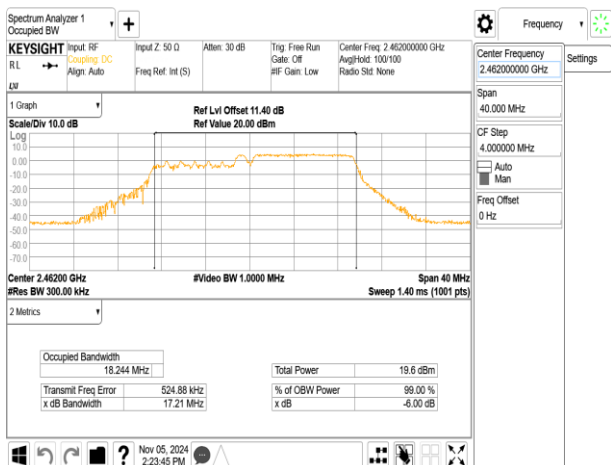
802.11be_20MHz_ChainA_2462MHz_52+26_MRU3
