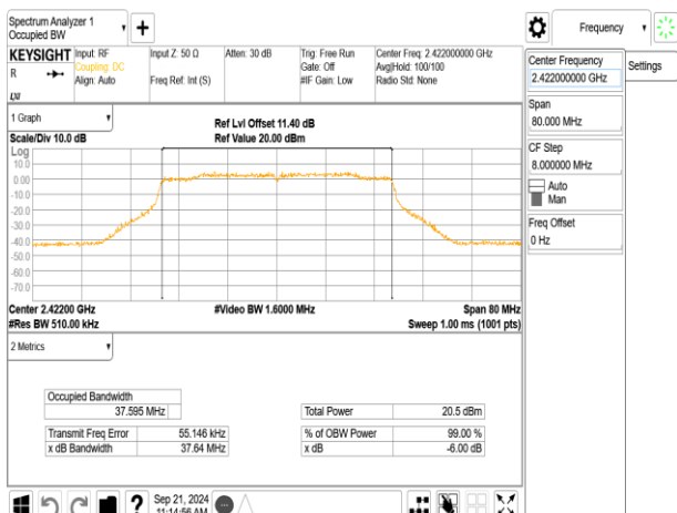
802.11be_40MHz_ChainA_2422MHz
