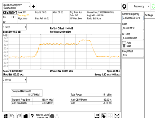
802.11ax_20MHz_ChainB_2472MHz_RU52_40
