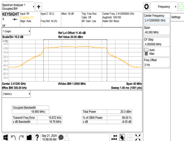
802.11be_20MHz_ChainB_2412MHz_106+26_MRU1
