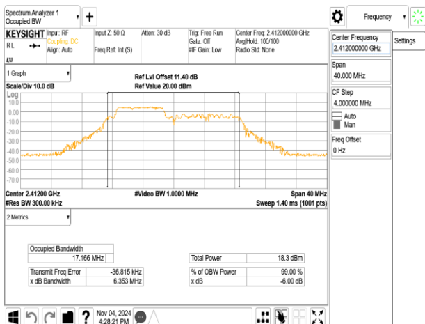
802.11be_20MHz_ChainA_2412MHz_RU106_53
