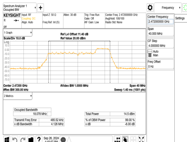
802.11be_20MHz_ChainA_2472MHz_RU52_40
