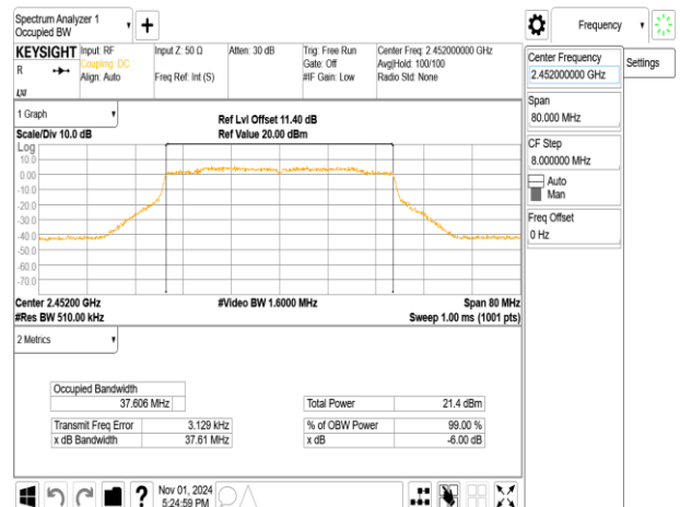
802.11ax_40MHz_ChainB_2452MHz
