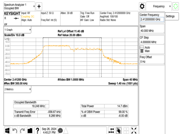
802.11be_20MHz_ChainB_2412MHz_RU26_0
