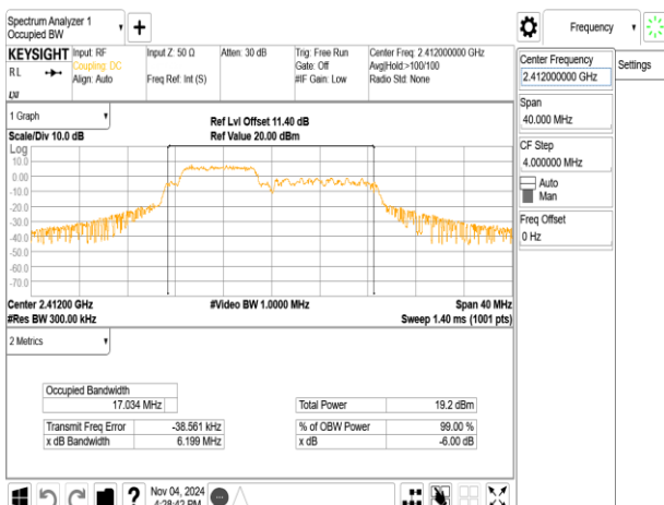
802.11be_20MHz_ChainB_2412MHz_52+26_MRU1
