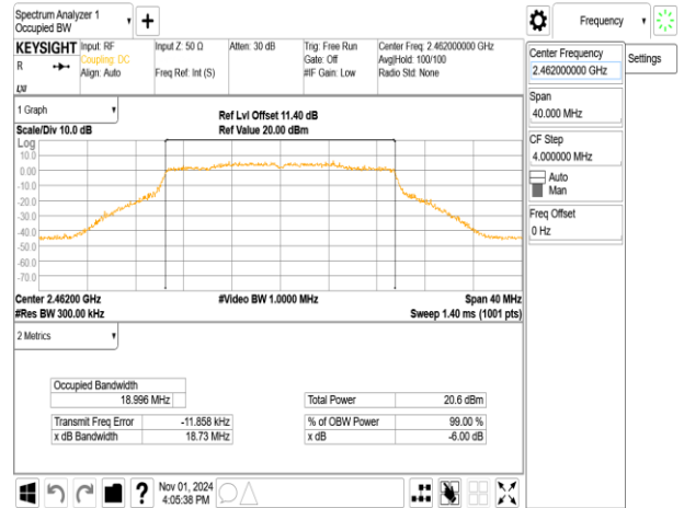
802.11ax_20MHz_ChainB_2462MHz_RU106_54
