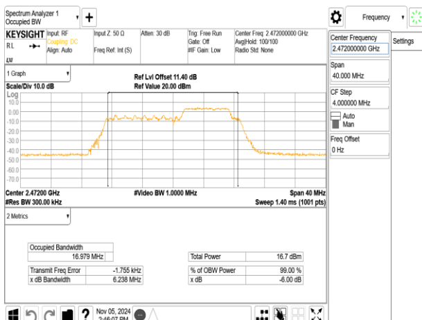
802.11be_20MHz_ChainA_2472MHz_52+26_MRUI3
