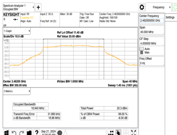
802.11be_20MHz_ChainA_2462MHz
