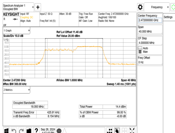
802.11be_20MHz_ChainB_2472MHz_RU106_54
