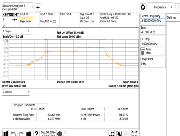
802.11be_20MHz_ChainA_2462MHz_RU106_54
