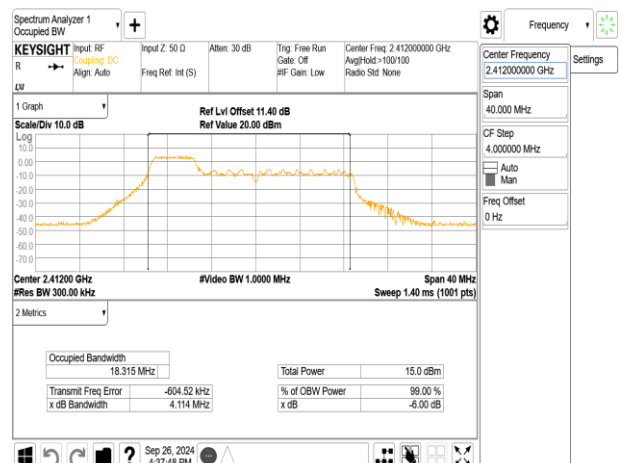
802.11be_20MHz_ChainB_2412MHz_RU52_37
