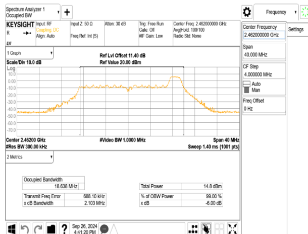
802.11be_20MHz_ChainA_2462MHz_RU52_40
