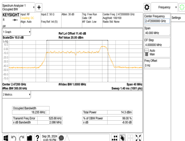
802.11be_20MHz_ChainB_2472MHz_RU52_40
