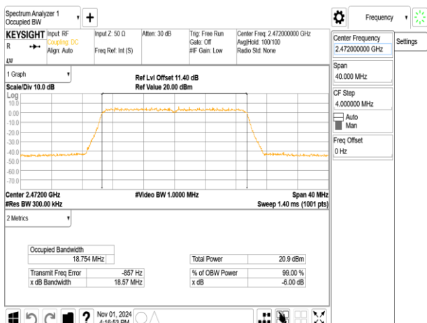
802.11ax_20MHz_ChainB_2472MHz
