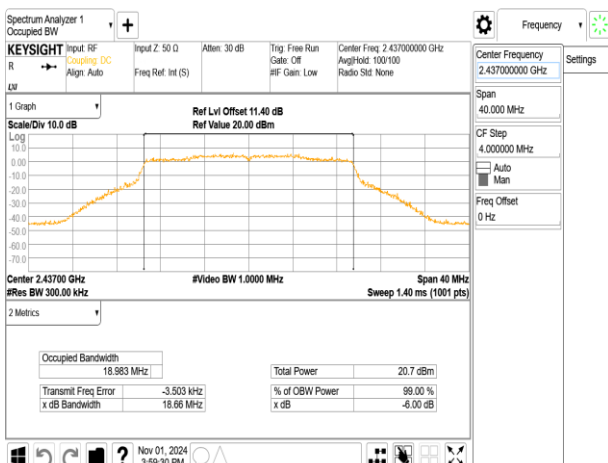
802.11ax_20MHz_ChainB_2437MHz
