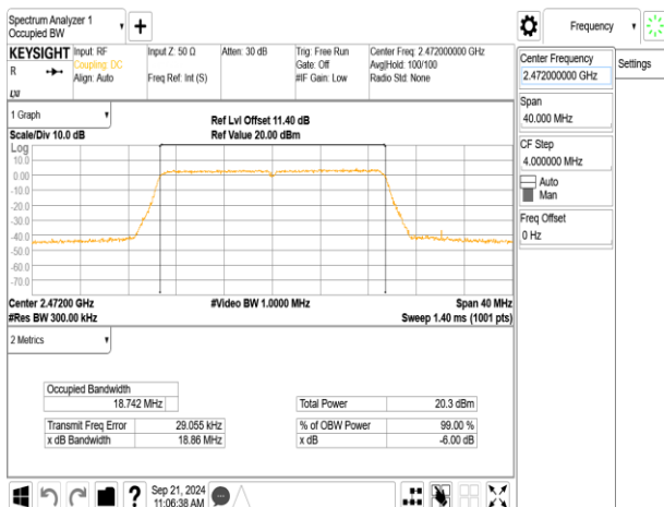
802.11be_20MHz_ChainA_2472MHz_106+26_MRUI2
