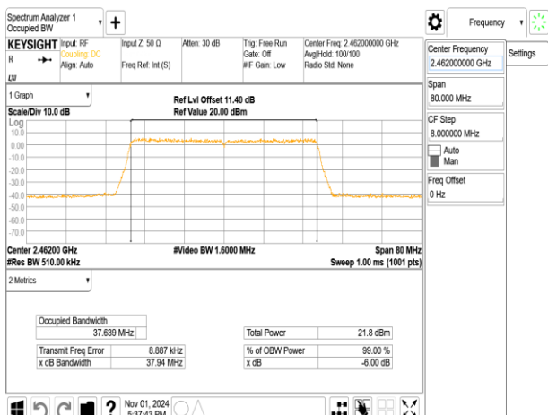
802.11ax_40MHz_ChainB_2462MHz
