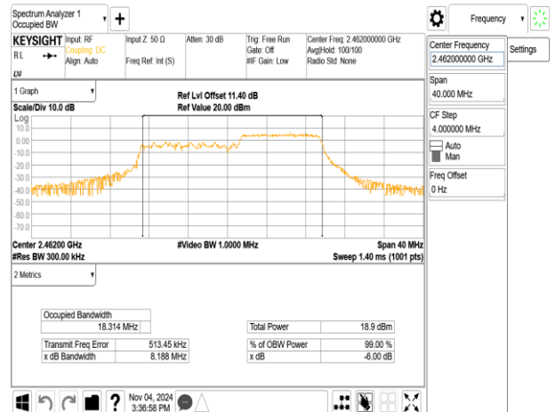
802.11ax_20MHz_ChainB_2462MHz_RU26_8
