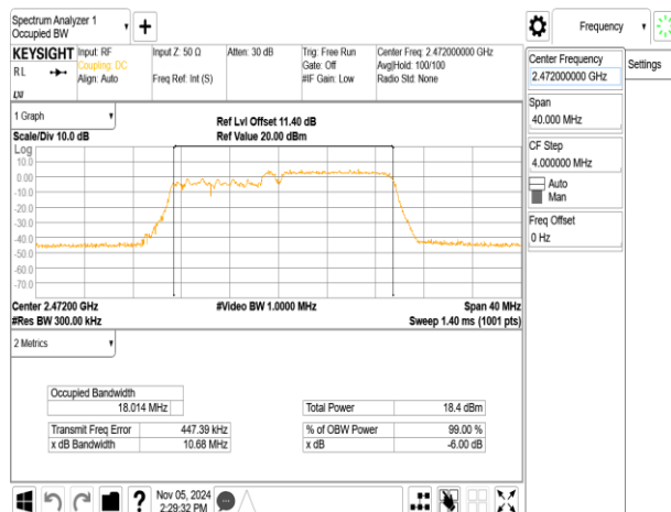
802.11be_20MHz_ChainB_2472MHz_52+26_MRU3
