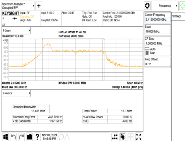
802.11ax_20MHz_ChainB_2412MHz_RU52_37
