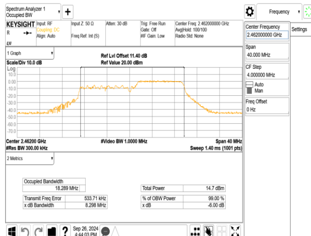
802.11be_20MHz_ChainB_2462MHz_RU26_8
