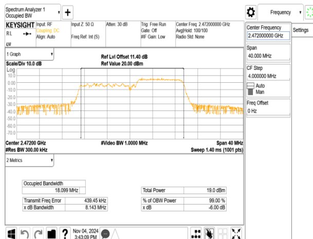
802.11ax_20MHz_ChainB_2472MHz_RU26_8
