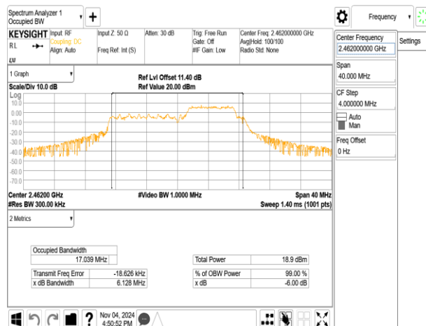
802.11be_20MHz_ChainB_2462MHz_RU106_54
