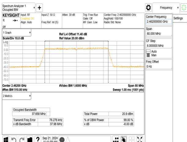
802.11be_40MHz_ChainA_2462MHz
