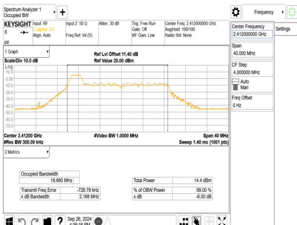
802.11be_20MHz_ChainA_2412MHz_RU26_0
