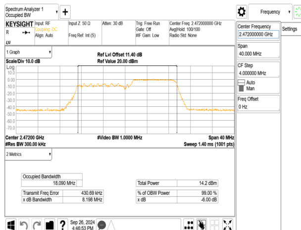
802.11be_20MHz_ChainA_2472MHz_RU26_8
