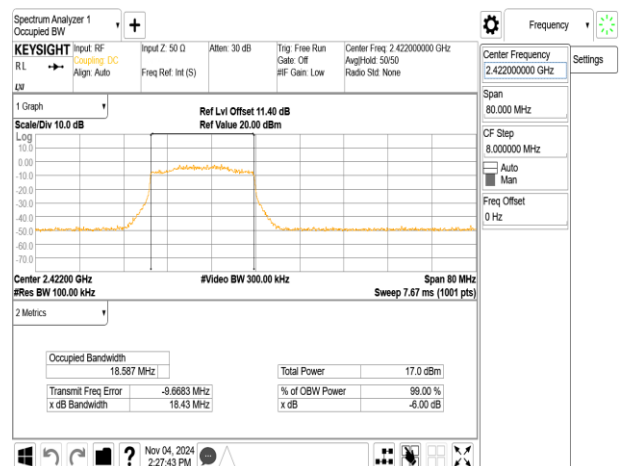
802.11be_40MHz_ChainB_2422MHz_RU242_61
