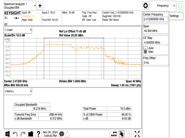
802.11ax_20MHz_ChainA_2412MHz_RU26_0
