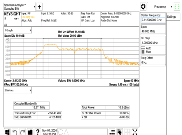
802.11ax_20MHz_ChainA_2412MHz_RU52_37
