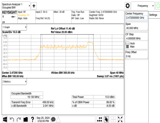
802.11be_20MHz_ChainB_2472MHz_RU52_40
