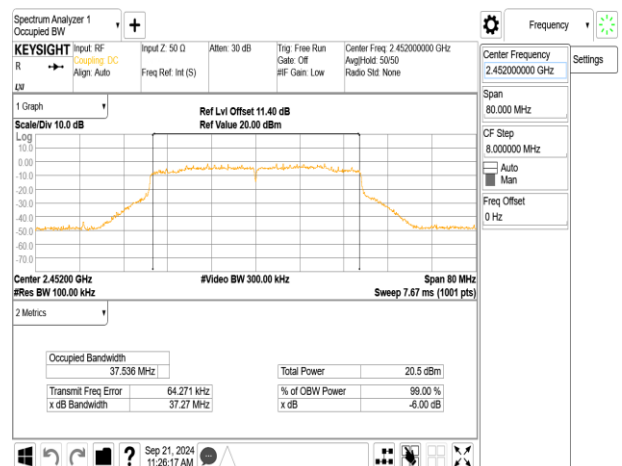
802.11be_40MHz_ChainA_2452MHz
