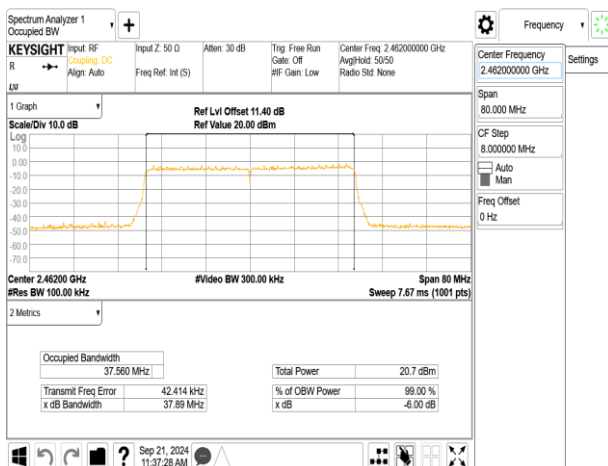
802.11be_40MHz_ChainA_2462MHz
