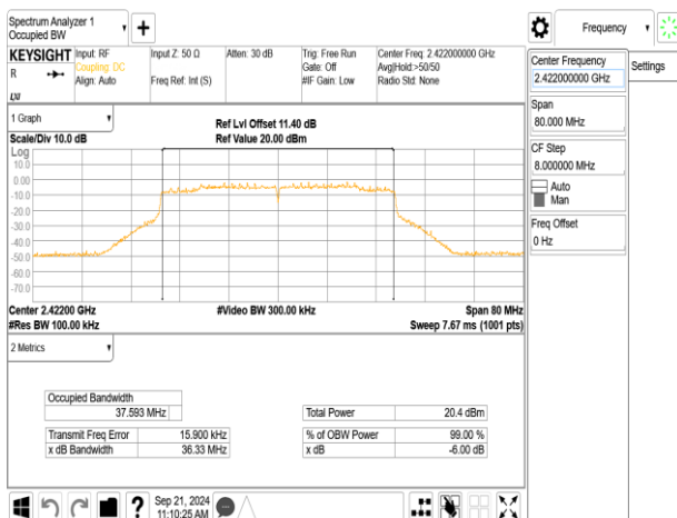
802.11be_40MHz_ChainA_2422MHz
