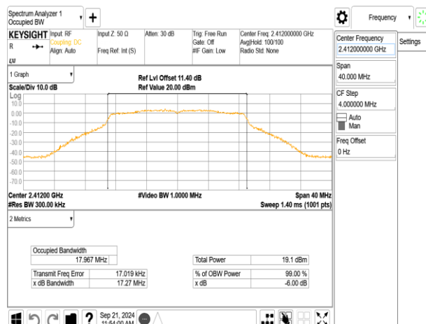
802.11n_20MHz_ChainB_2412MHz
