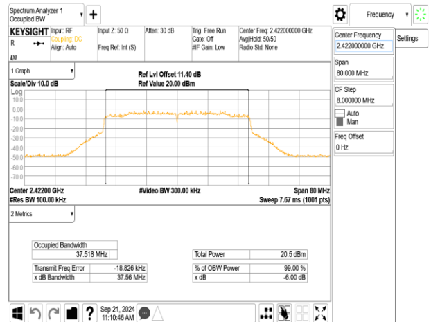
802.11be_40MHz_ChainB_2422MHz_RU242_61
