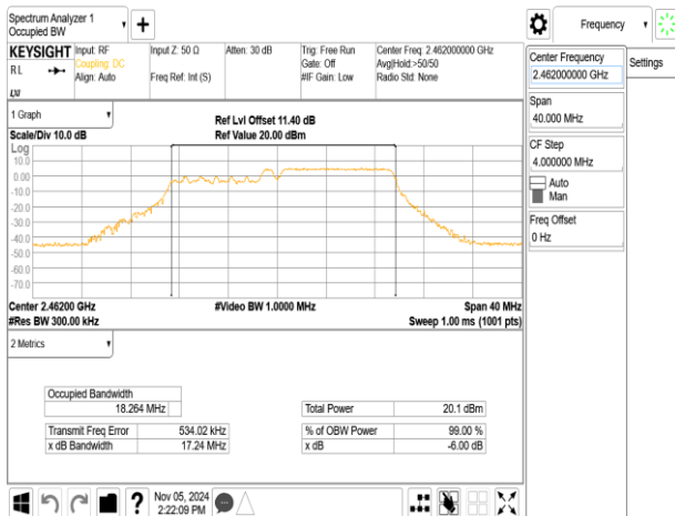
802.11be_20MHz_ChainA_2462MHz_52+26_MRU3
