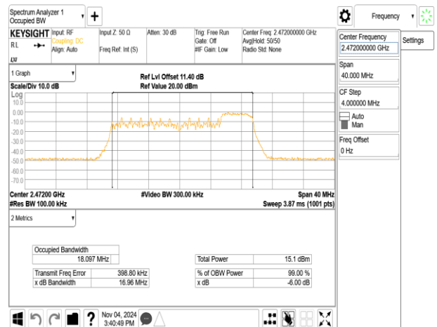
802.11ax_20MHz_ChainB_2472MHz_RU52_40
