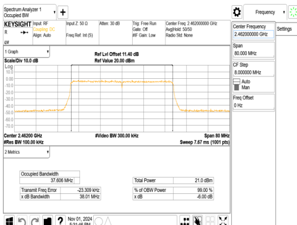
802.11ax_40MHz_ChainB_2462MHz
