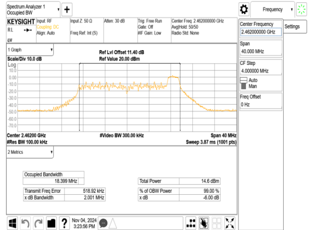
802.11ax_20MHz_ChainA_2462MHz_RU52_40
