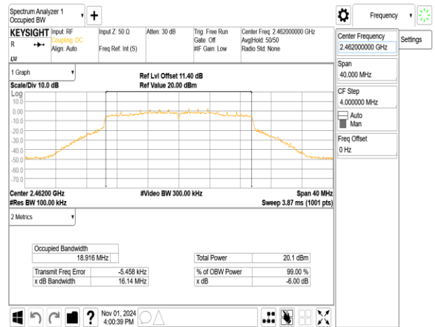
802.11ax_20MHz_ChainB_2462MHz_RU106_54
