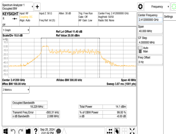
802.11be_20MHz_ChainA_2412MHz_RU26_0
