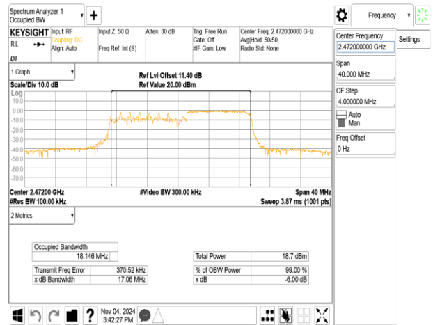
802.11ax_20MHz_ChainB_2472MHz_RU26_8
