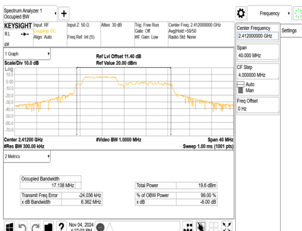
802.11be_20MHz_ChainB_2412MHz_52+26_MRUI
