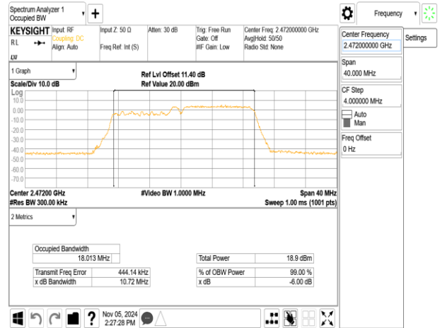
802.11be_20MHz_ChainB_2472MHz_52+26_MRU3
