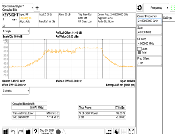
802.11be_20MHz_ChainA_2462MHz_RU106_54
