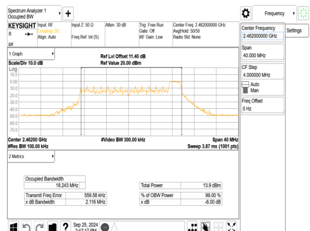
802.11be_20MHz_ChainB_2462MHz_RU26_8
