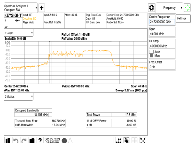
802.11be_20MHz_ChainB_2472MHz_RU106_54
