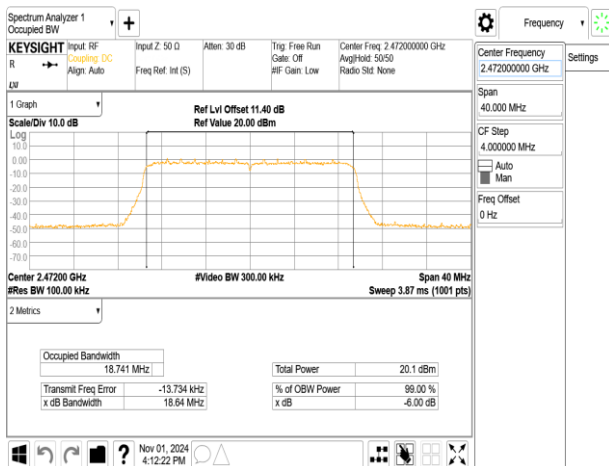
802.11ax_20MHz_ChainB_2472MHz
