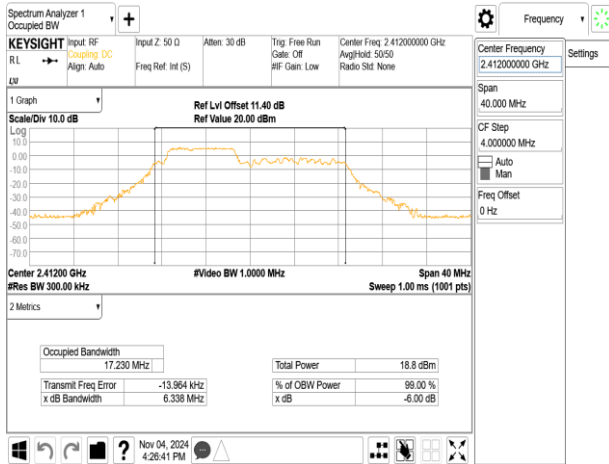
802.11be_20MHz_ChainA_2412MHz_RU106_53
