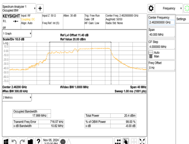
802.11be_20MHz_ChainB_2462MHz_106+26_MRUI2
