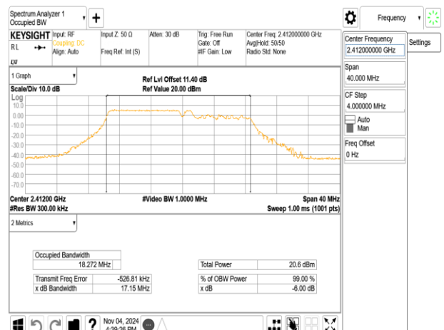
802.11be_20MHz_ChainA_2412MHz_106+26_MRU1
