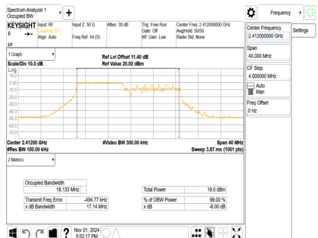
802.11ax_20MHz_ChainB_2412MHz_RU106_53
