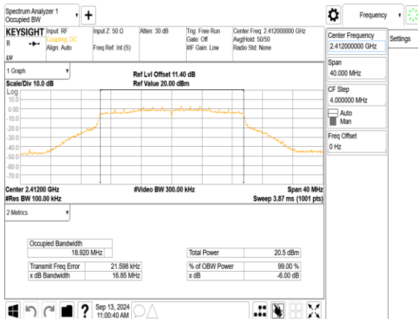
802.11be_20MHz_ChainB_2412MHz_106+26_MRUI
