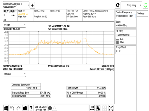
802.11be_20MHz_ChainA_2462MHz_RU52_40
