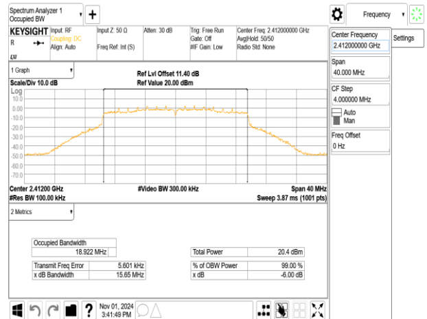
802.11ax_20MHz_ChainB_2412MHz_RU106_53
