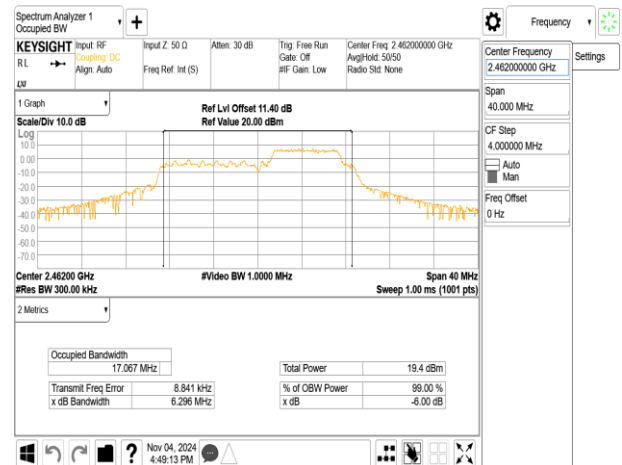
802.11be_20MHz_ChainB_2462MHz_RU106_54
