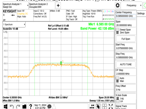
802.11be_320MHz_6585MHz(U-NII-7)_AWGN:6585MHz
