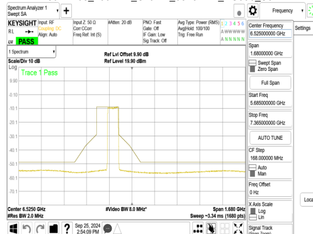
802.11be_160MHz_ChainB_6345MHz_RU996_S67
