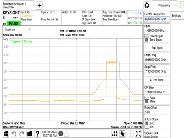
802.11be_160MHz_ChainA_6985MHz_RU996_67
