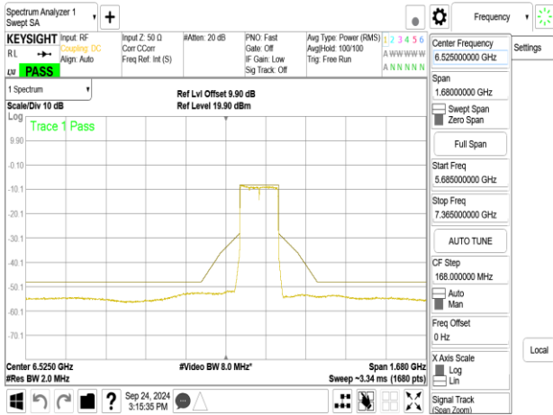
802.11be_160MHz_ChainB_6665MHz_996+484+242_MRU1
