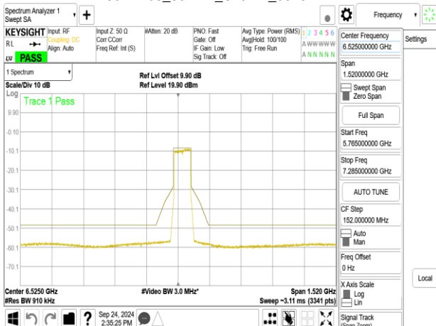
802.11be_80MHz_ChainA_6545MHz
