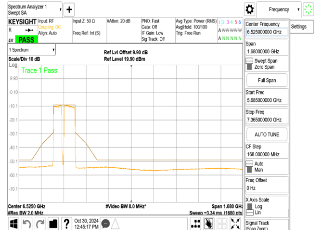
802.11be_160MHz_ChainA_6025MHz_996+484+242_MRU8
