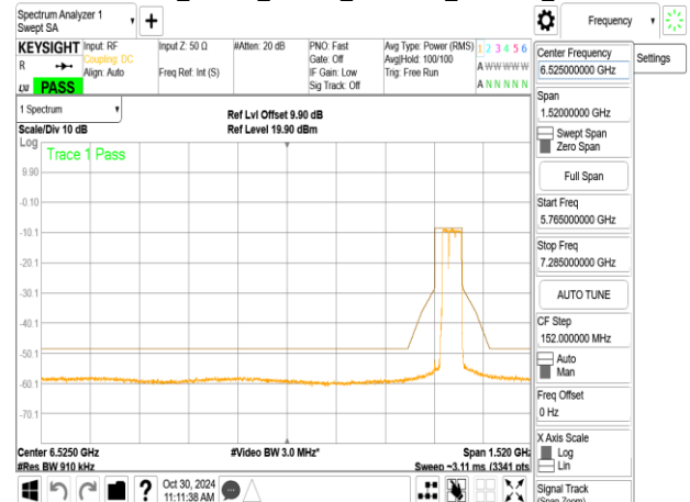
802.11be_80MHz_ChainB_7025MHz_484+242_MRU1
