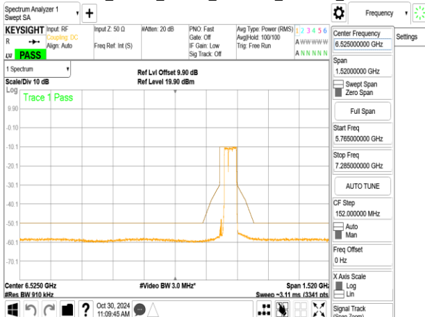
802.11be_80MHz_ChainB_6785MHz_484+242_MRU1
