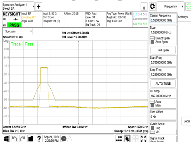
802.11be_80MHz_ChainA_6145MHz
