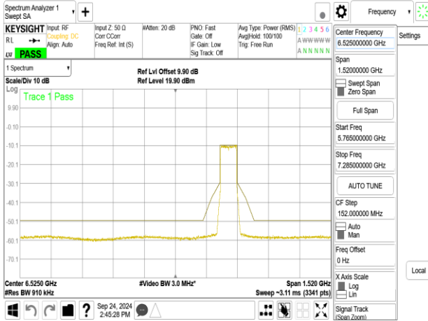
802.11be_80MHz_ChainB_6785MHz_484+242_MRU1
