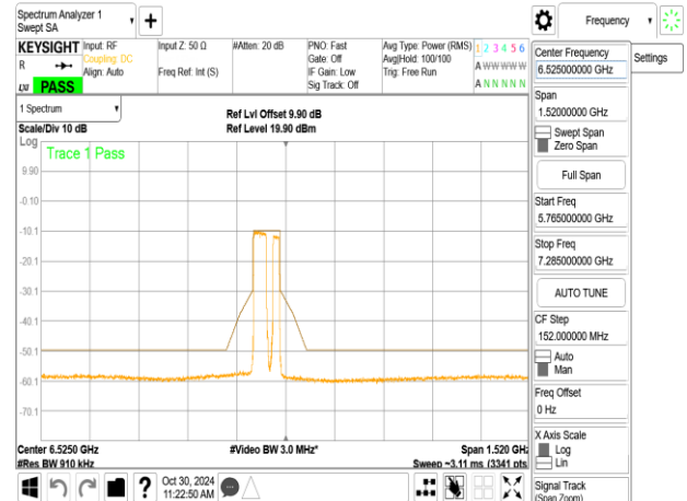
802.11be_80MHz_ChainA_6465MHz_484+242_MRU4
