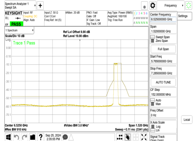
802.11be_80MHz_ChainB_7025MHz
