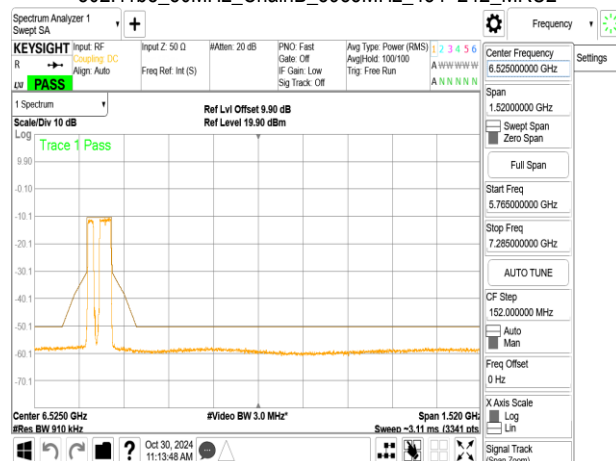
802.11be_80MHz_ChainB_5985MHz_484+242_MR4
