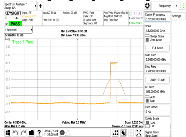
802.11be_80MHz_ChainA_6945MHz_RU484_65
