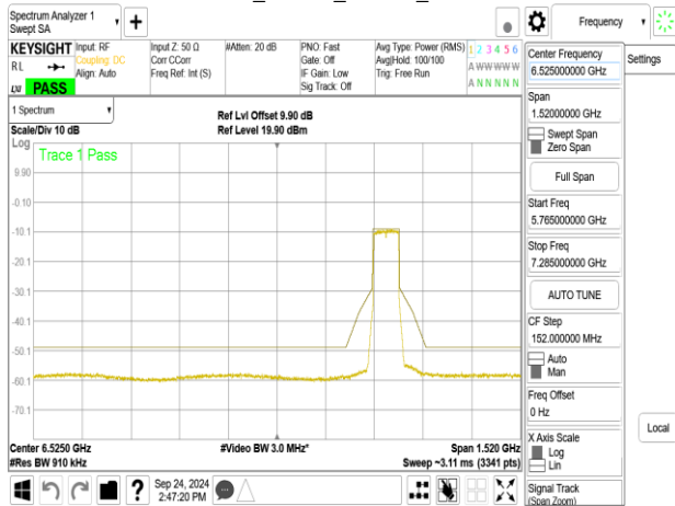
802.11be_80MHz_ChainA_6945MHz
