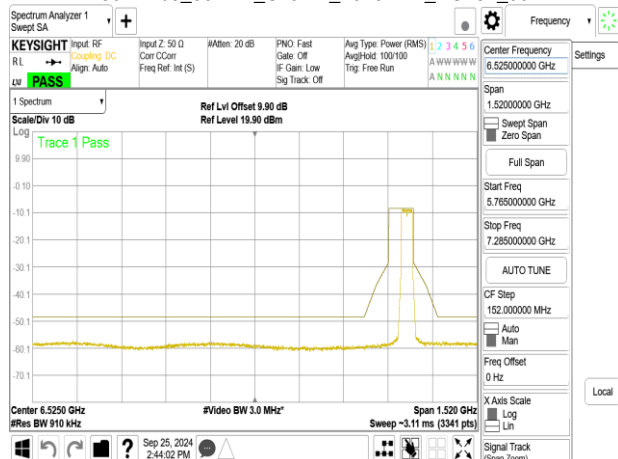
802.11be_80MHz_ChainA_7025MHz_RU484_66
