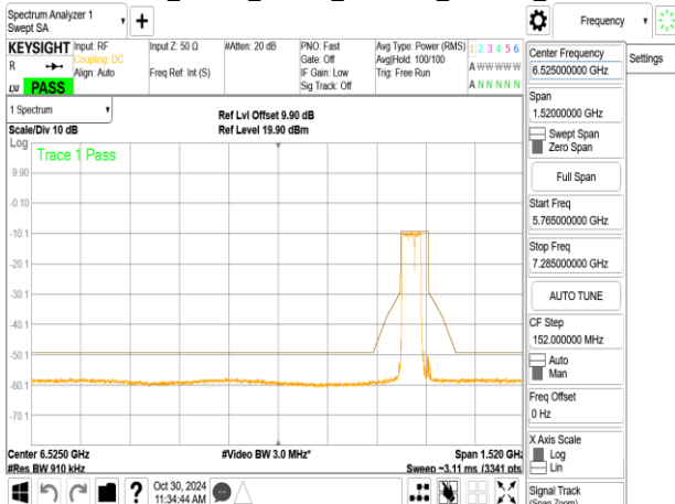
802.11be_80MHz_ChainB_6945MHz_484+242_MRU4
