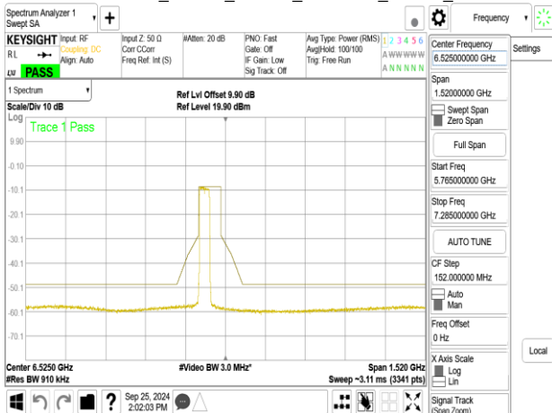
802.11be_80MHz_ChainA_6465MHz_RU484_66
