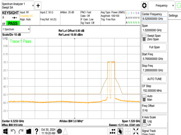
802.11be_80MHz_ChainB_6945MHz_484+242_MRU4
