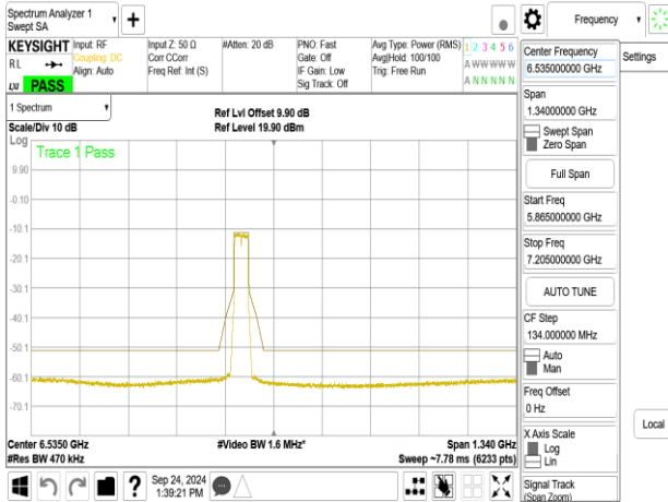
802.11be_40MHz_ChainB_6445MHz_RU242_61
