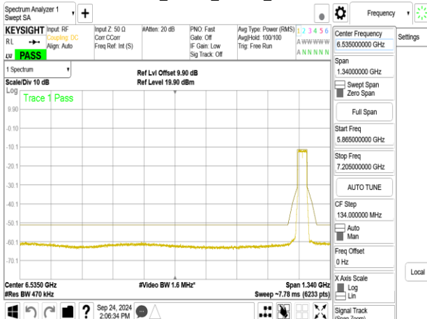
802.11be_40MHz_ChainB_7085MHz
