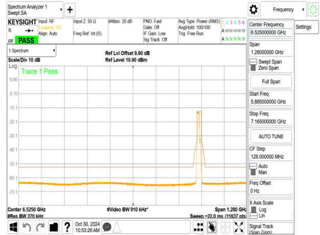
802.11be_20MHz_ChainB_6895MHz_52+26_MRUI
