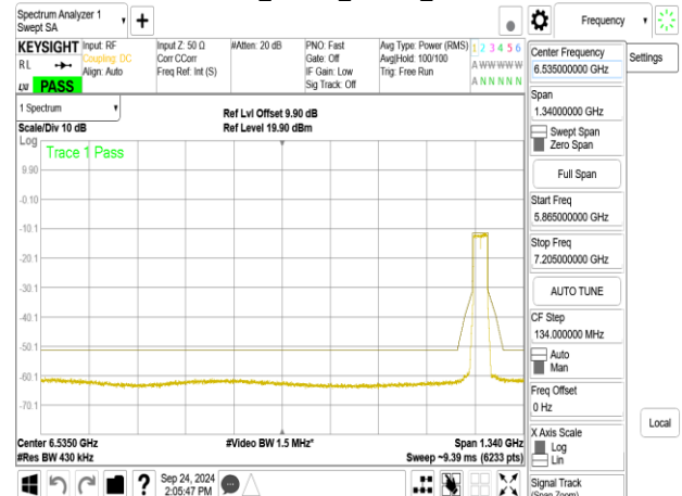
802.11be_40MHz_ChainA_7085MHz
