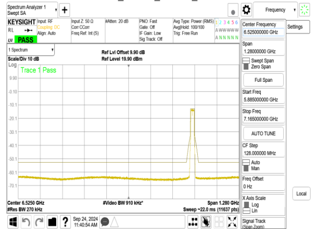
802.11be_20MHz_ChainB_6895MHz_106+26_MRUI
