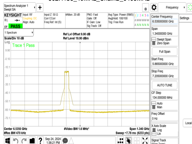
802.11be_40MHz_ChainB_6405MHz_RU242_62
