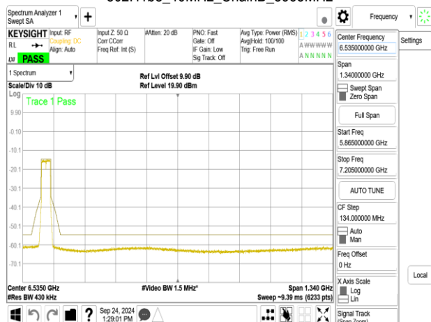
802.11be_40MHz_ChainB_5965MHz_RU242_61
