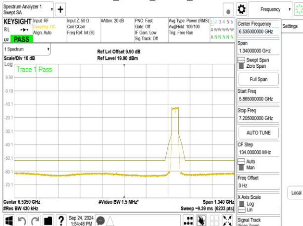
802.11be_40MHz_ChainB_6845MHz
