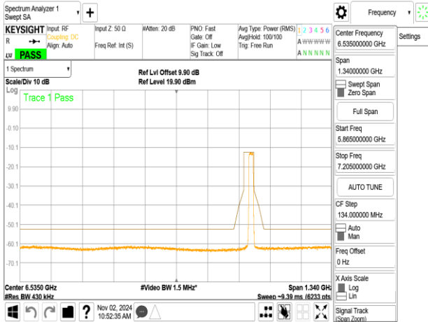
802.11be_40MHz_ChainA_6885MHz
