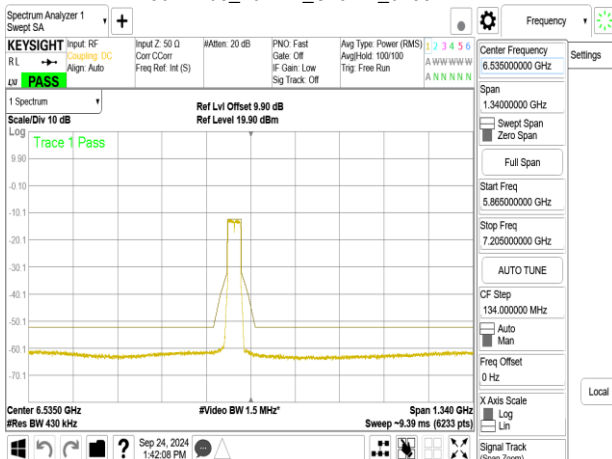
802.11be_40MHz_ChainB_6485MHz
