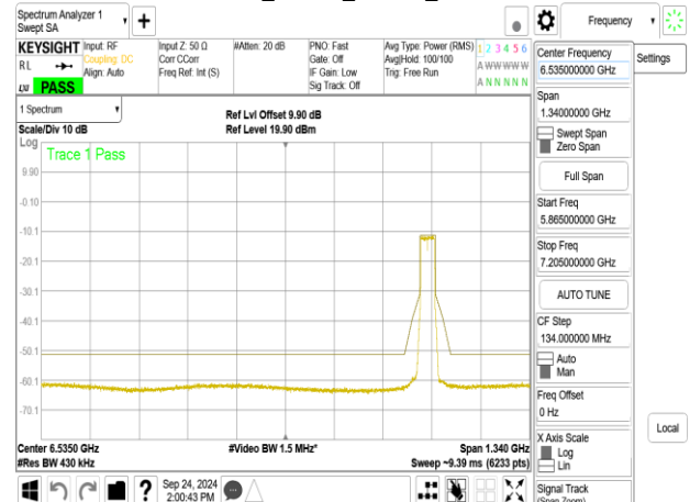
802.11be_40MHz_ChainB_6925MHz
