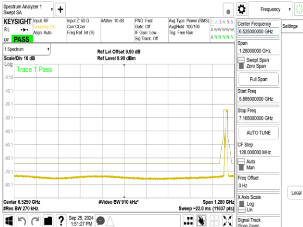
802.11be_20MHz_ChainB_7115MHz_RU26_8
