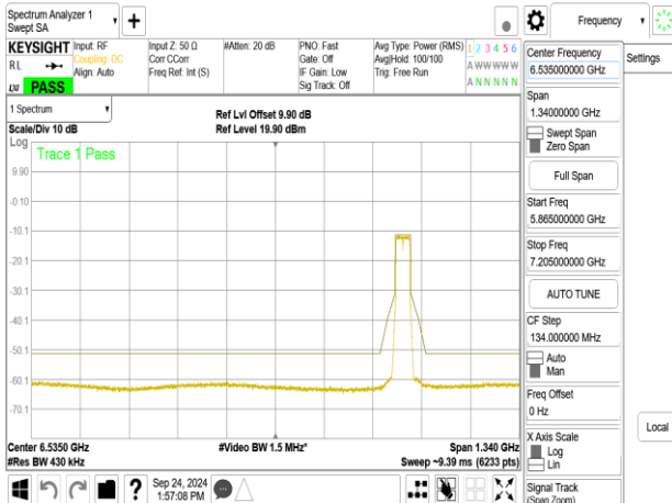
802.11be_40MHz_ChainA_6925MHz
