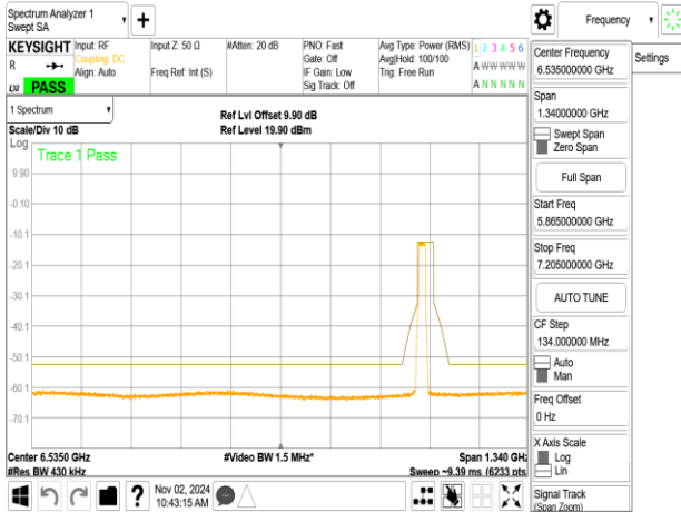
802.11be_40MHz_ChainB_7005MHz
