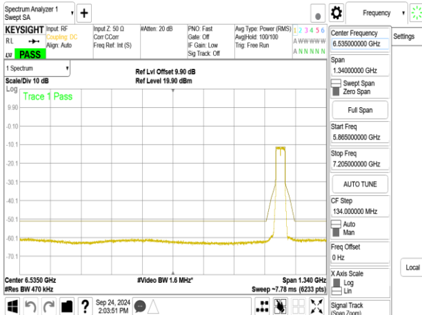
802.11be_40MHz_ChainB_7085MHz
