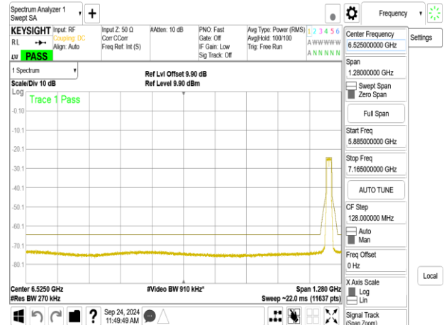
802.11be_20MHz_ChainB_7115MHz_106+26_MRU2
