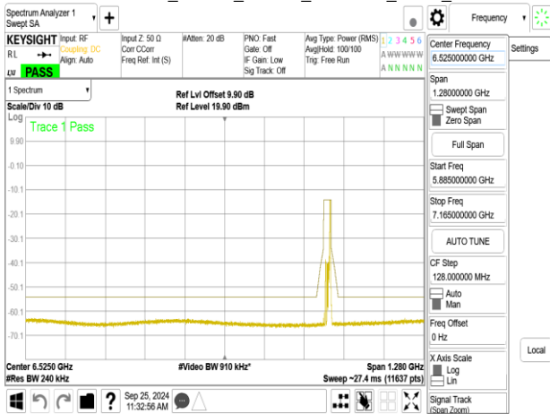
802.11be_20MHz_ChainB_6855MHz_RU52_40
