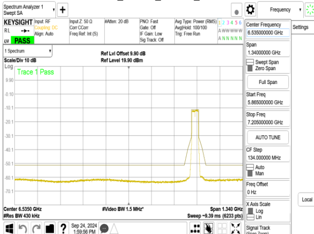
802.11be_40MHz_ChainA_6925MHz
