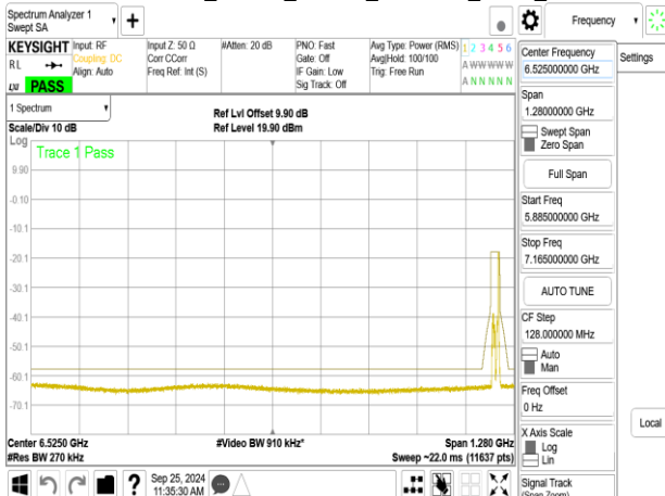
802.11be_20MHz_ChainB_7115MHz_RU26_8
