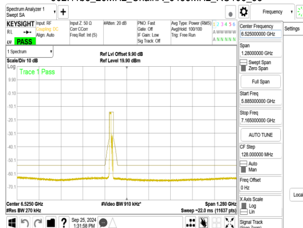
802.11be_20MHz_ChainA_6435MHz_RU26_0
