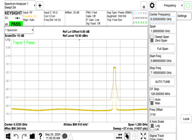
802.11be_20MHz_ChainA_6855MHz_106+26_MRU2
