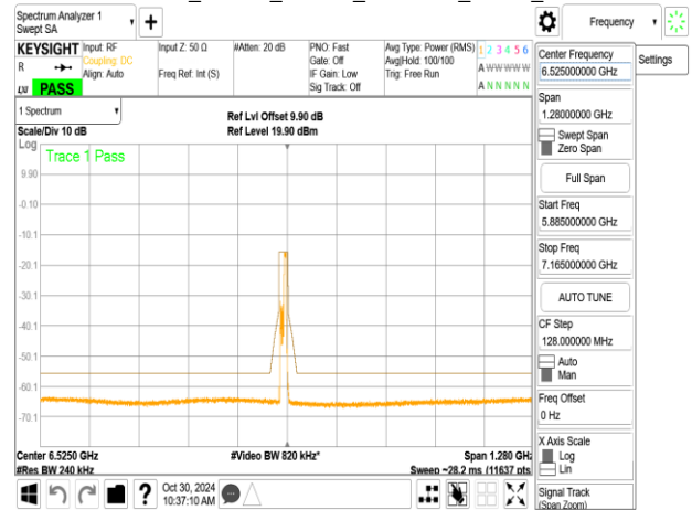
802.11be_20MHz_ChainB_6515MHz_RU106_54
