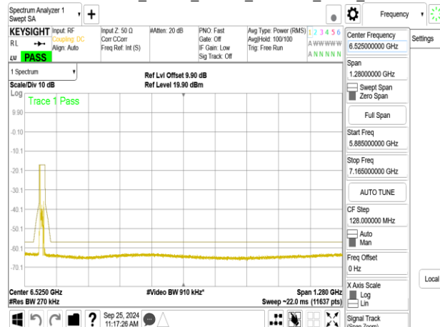
802.11be_20MHz_ChainB_5955MHz_RU52_37
