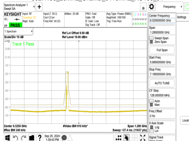
802.11be_20MHz_ChainB_6415MHz_RU26_8
