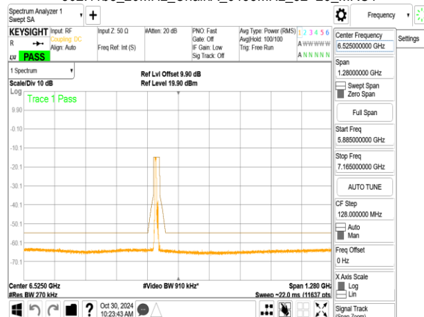
802.11be_20MHz_ChainA_6435MHz_RU106_53
