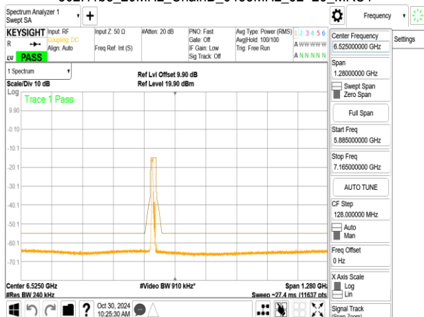
802.11be_20MHz_ChainB_6435MHz_52+26_MRUI
