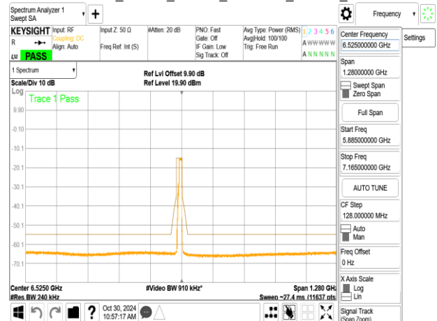
802.11be_20MHz_ChainA_6515MHz_52+26_MRU3
