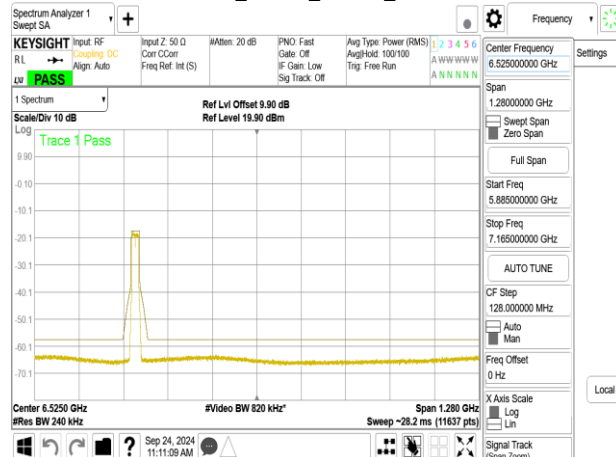
802.11be_20MHz_ChainB_6175MHz
