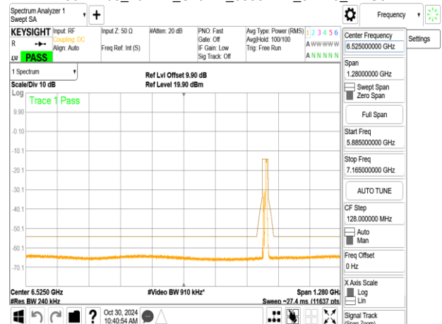
802.11be_20MHz_ChainA_6855MHz_52+26_MRU3
