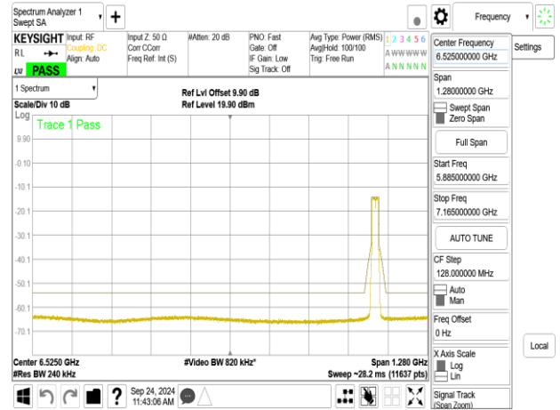
802.11be_20MHz_ChainA_7115MHz
