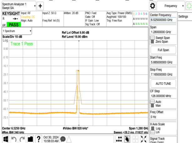
802.11be_20MHz_ChainB_6515MHz_106+26_MRUG
