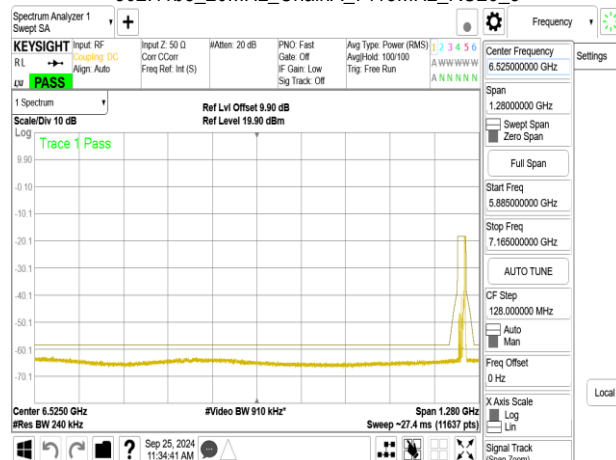
802.11be_20MHz_ChainA_7115MHz_RU52_40
