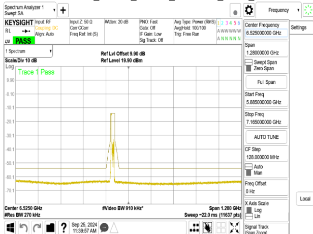
802.11be_20MHz_ChainA_6475MHz
