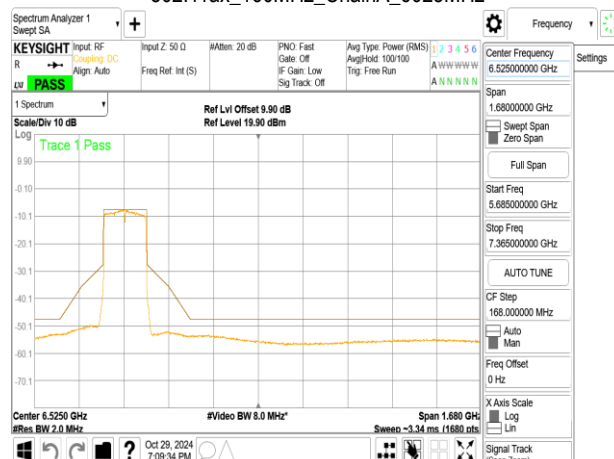
802.11ax_160MHz_ChainA_6025MHz_RU996_67
