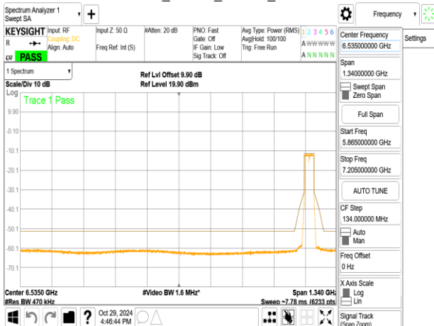
802.11ax_40MHz_ChainB_7085MHz_RU242_62
