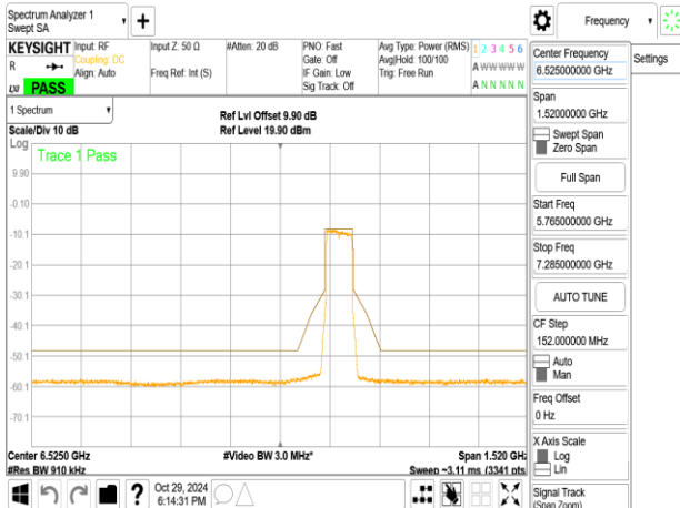
802.11ax_80MHz_ChainA_6785MHz
