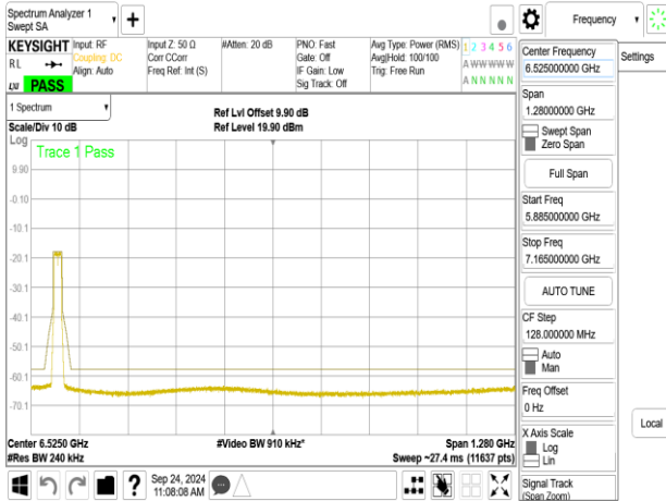
802.11be_20MHz_ChainA_5955MHz_106+26_MRUI
