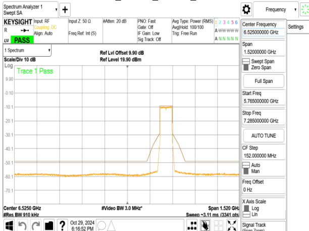
802.11ax_80MHz_ChainA_6785MHz
