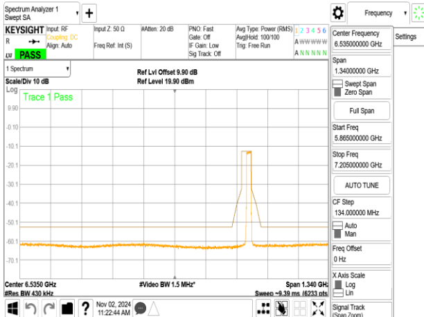
802.11ax_40MHz_ChainB_6885MHz
