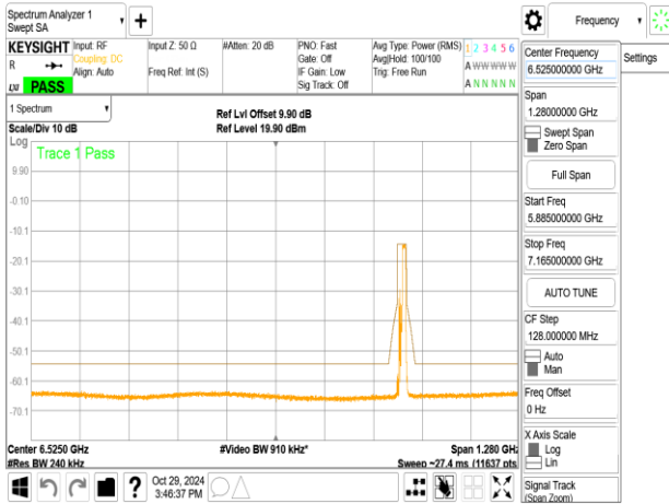
802.11ax_20MHz_ChainB_6855MHz_RU26_8
