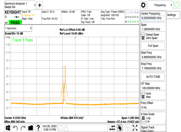
802.11ax_20MHz_ChainB_6435MHz
