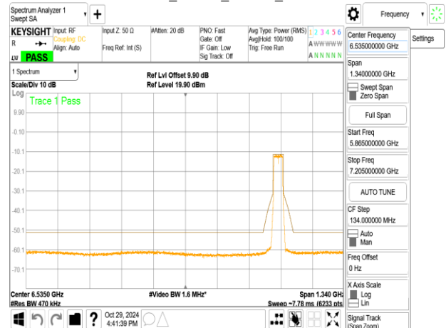
802.11ax_40MHz_ChainB_6925MHz_RU242_61
