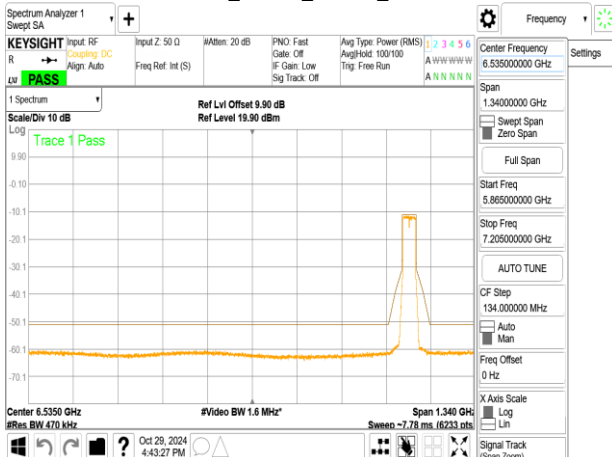
802.11ax_40MHz_ChainA_7005MHz
