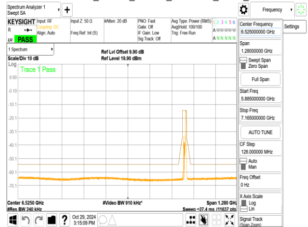
802.11ax_20MHz_ChainB_6875MHz
