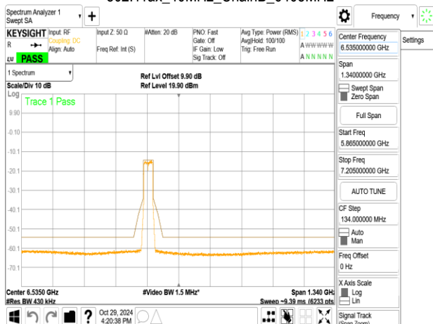
802.11ax_40MHz_ChainB_6405MHz
