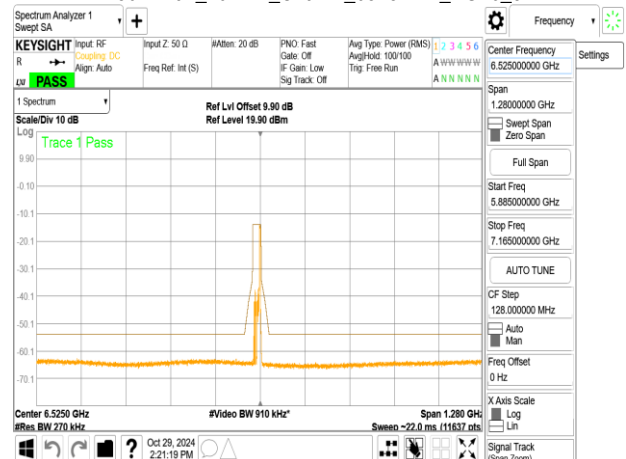
802.11ax_20MHz_ChainB_6515MHz_RU26_8
