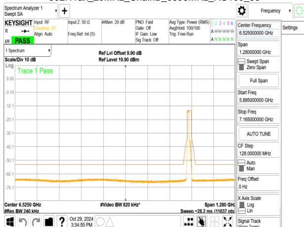
802.11ax_20MHz_ChainB_6895MHz_RU26_0
