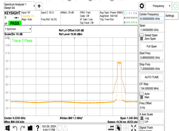
802.11ax_40MHz_ChainB_7005MHz
