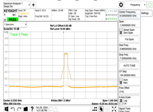
802.11ax_40MHz_ChainB_6565MHz_RU242_61
