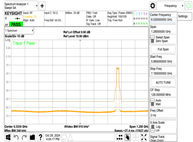
802.11ax_20MHz_ChainB_6895MHz
