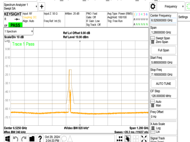
802.11ax_20MHz_ChainA_6435MHz_RU26_0
