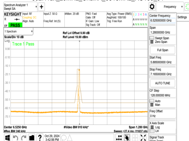
802.11ax_20MHz_ChainA_6515MHz_RU26_8
