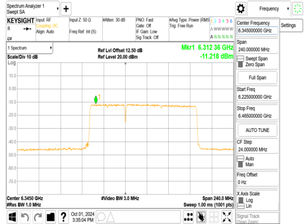
802.11be_160MHz_ChainB_6345MHz_996+484_MR3
