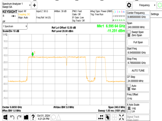
802.11be_160MHz_ChainB_6665MHz_996+484+242_MRU8
