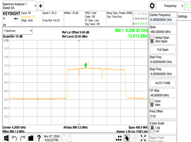
802.11be_320MHz_ChainA_6265MHz_3x996+484_MRU1
