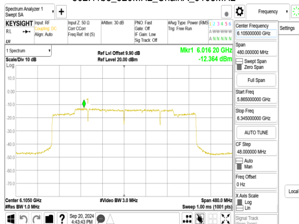
802.11be_320MHz_ChainA_6105MHz_2x996+484_MRU2
