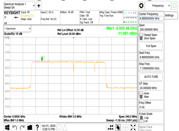
802.11be_160MHz_ChainB_6985MHz_996+484_MR1
