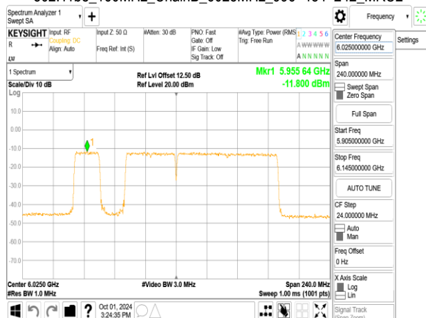
802.11be_160MHz_ChainB_6025MHz_996+484+242_MRU4
