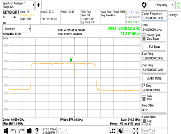
802.11be_160MHz_ChainB_6025MHz_996+484_MRU4
