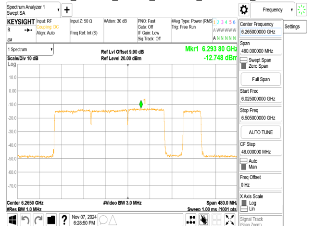
802.11be_320MHz_ChainA_6265MHz_3x996_MRU1
