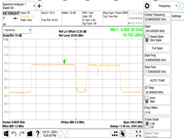
802.11be_160MHz_ChainA_6985MHz_996+484+242_MR07
