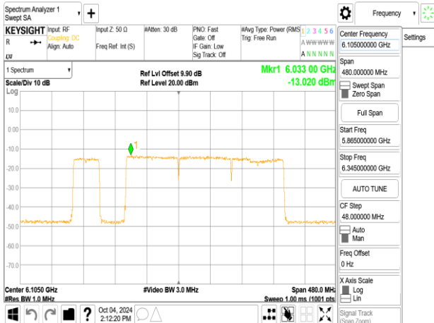
802.11be_320MHz_ChainA_6105MHz_3x996+484_MRU8
