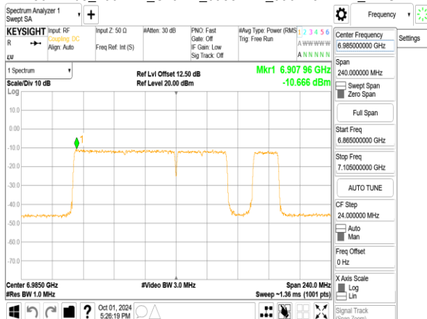
802.11be_160MHz_ChainB_6985MHz_996+484+242_MR7
