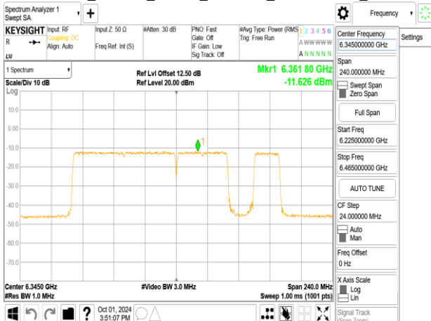
802.11be_160MHz_ChainB_6345MHz_996+484+242_MR7
