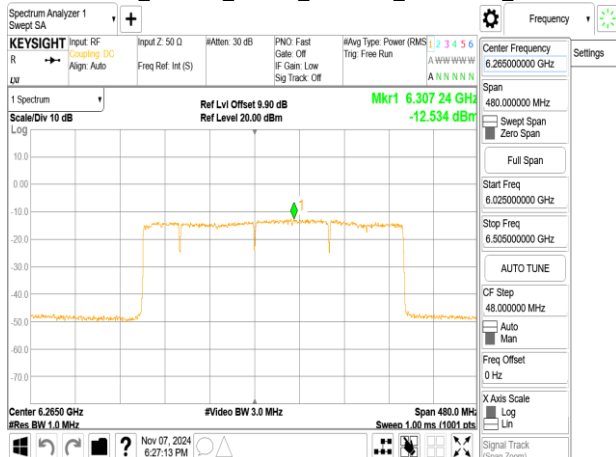
802.11be_320MHz_ChainA_6265MHz_3x996+484_MRU1
