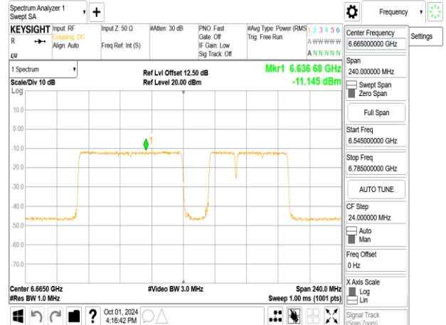
802.11be_160MHz_ChainB_6665MHz_996+484+242_MRU5
