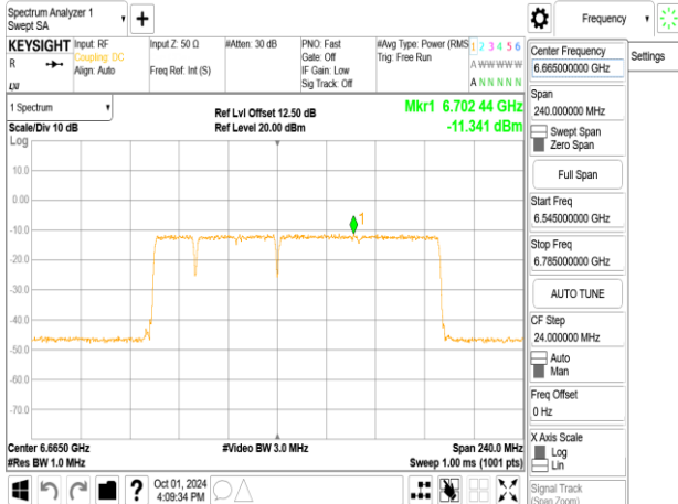
802.11be_160MHz_ChainB_6665MHz_996+484+242_MRU1
