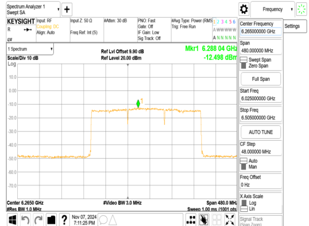
802.11be_320MHz_ChainA_6265MHz_3x996_MRU3
