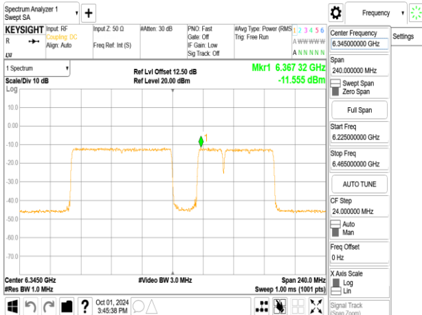
802.11be_160MHz_ChainB_6345MHz_996+484+242_MR7
