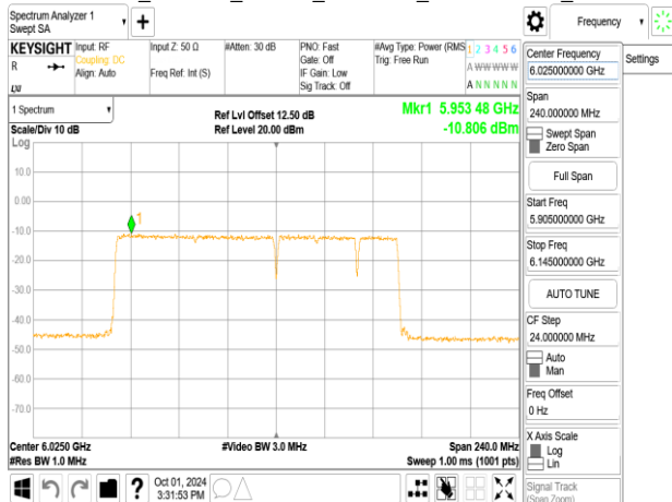
802.11be_160MHz_ChainB_6025MHz_996+484_MRU2
