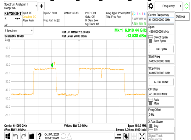
802.11be_320MHz_ChainA_6105MHz_3x996_MRU4
