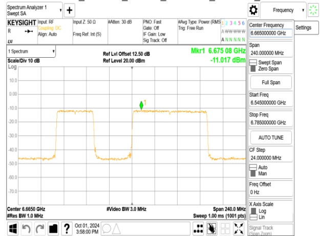
802.11be_160MHz_ChainB_6665MHz_996+484_MRU3
