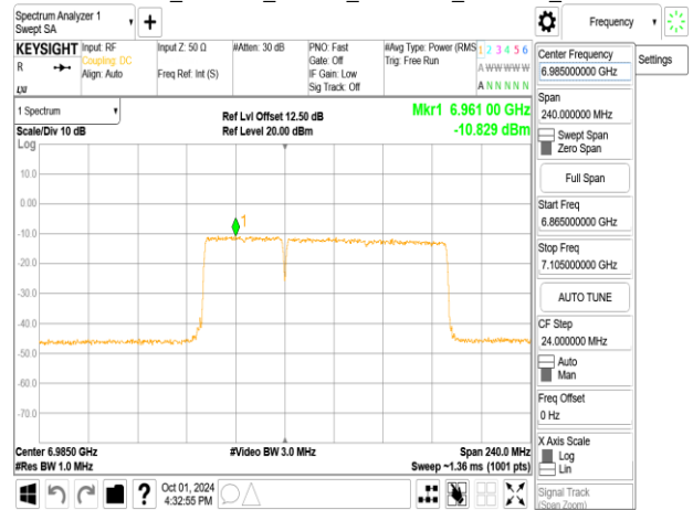
802.11be_160MHz_ChainA_6985MHz_996+484_MR02
