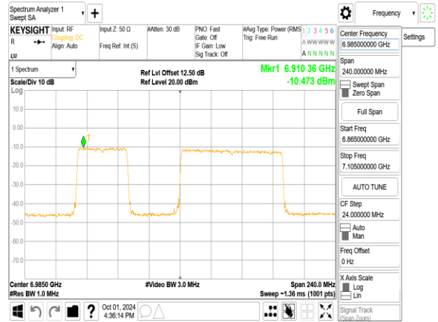
802.11be_160MHz_ChainA_6985MHz_996+484_MR03
