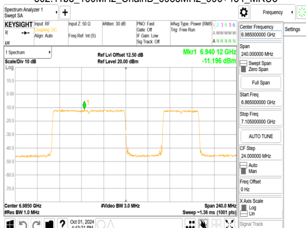
802.11be_160MHz_ChainB_6985MHz_996+484_MRU4
