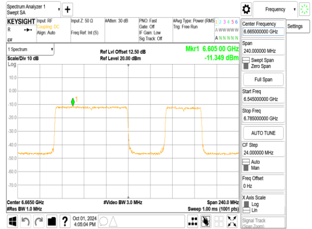
802.11be_160MHz_ChainB_6665MHz_996+484_MRU4
