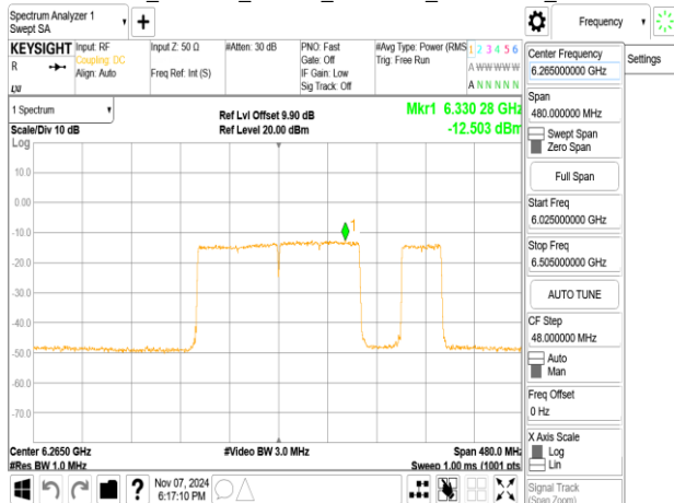
802.11be_320MHz_ChainA_6265MHz_2x996+484_MRU7
