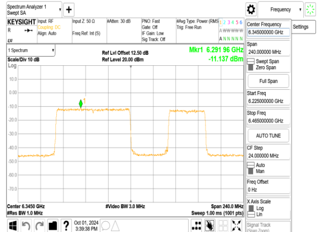
802.11be_160MHz_ChainB_6345MHz_RU996_S67
