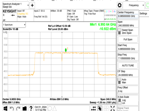
802.11be_160MHz_ChainB_6985MHz_996+484+242_MRUI
