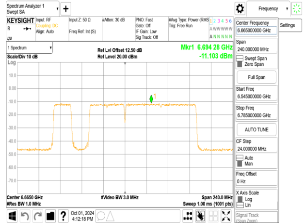
802.11be_160MHz_ChainB_6665MHz_996+484+242_MRU4
