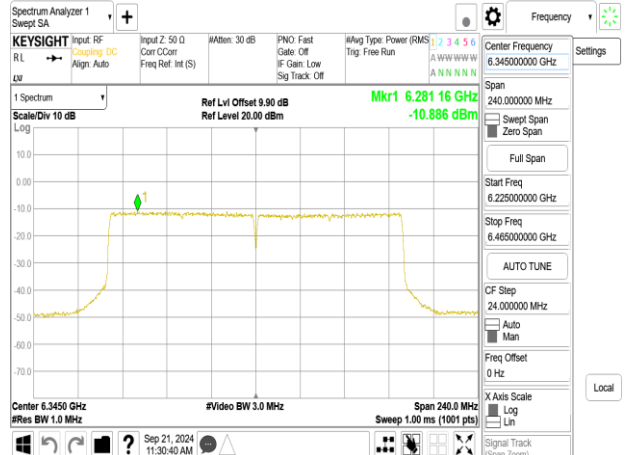
802.11be_160MHz_ChainB_6345MHz
