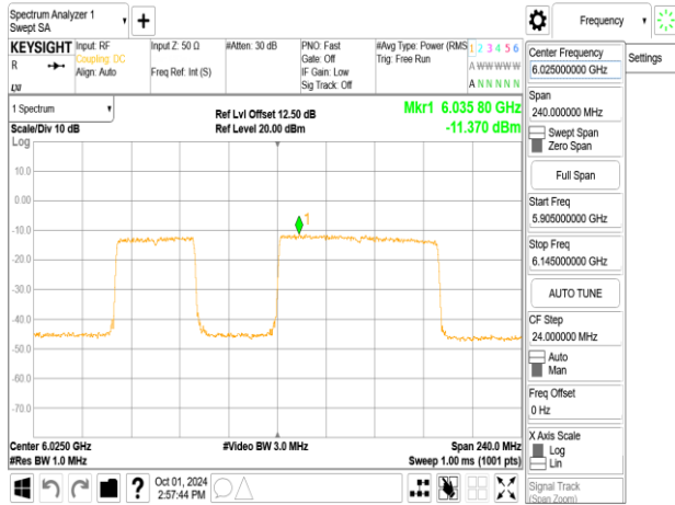
802.11be_160MHz_ChainB_6025MHz_996+484_MRU4
