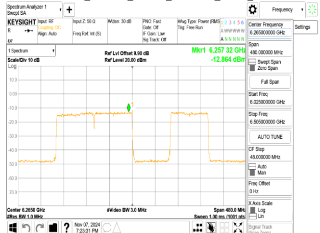
802.11be_320MHz_ChainA_6265MHz_3x996_MRU3
