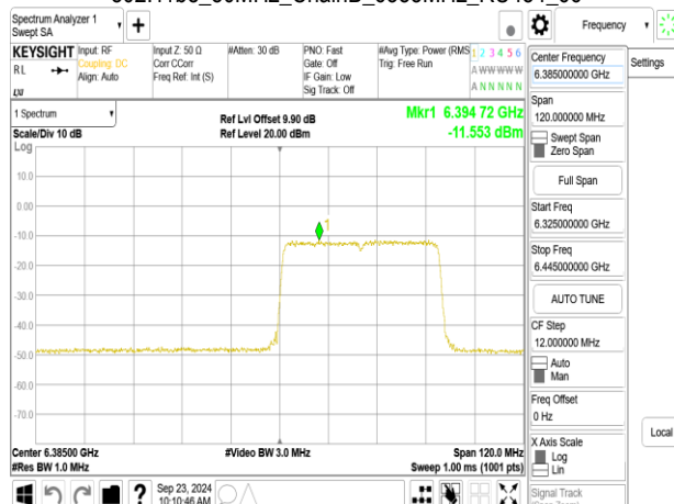
802.11be_80MHz_ChainB_6385MHz_RU484_66
