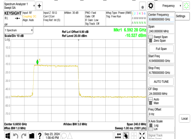
802.11be_160MHz_ChainA_6665MHz_RU996_67
