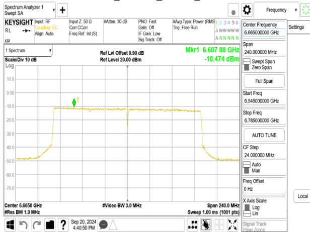
802.11be_160MHz_ChainA_6665MHz_996+484+242_MRU1
