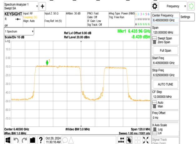
802.11be_80MHz_ChainB_6465MHz_484+242_MRU4
