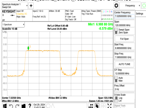
802.11be_80MHz_ChainA_7025MHz_RU484_66
