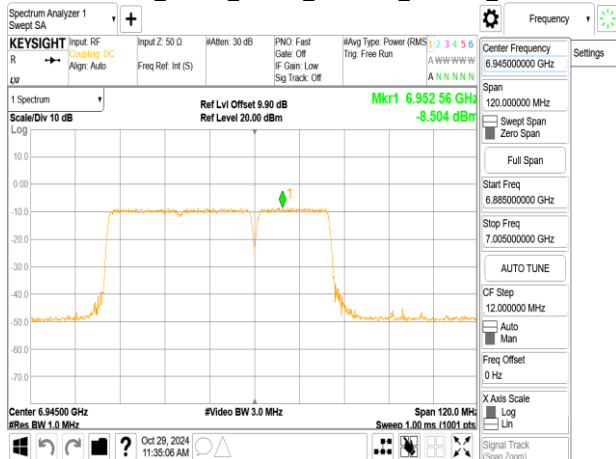
802.11be_80MHz_ChainB_6945MHz_484+242_MRU4
