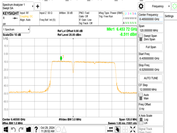
802.11be_80MHz_ChainB_6465MHz_484+242_MRU2
