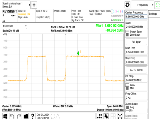
802.11be_160MHz_ChainA_6665MHz_996+484_MRU2
