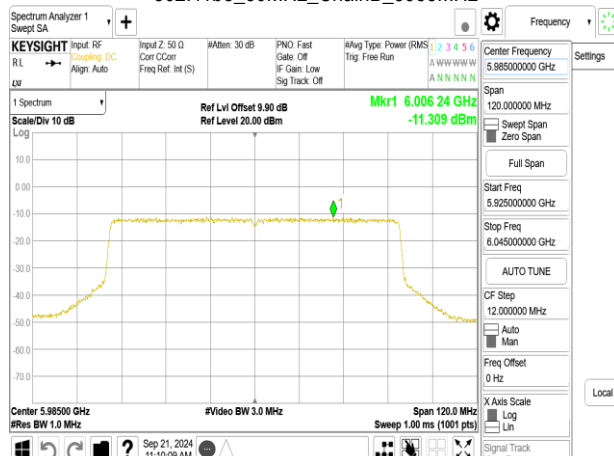
802.11be_80MHz_ChainB_5985MHz_484+242_MRU2
