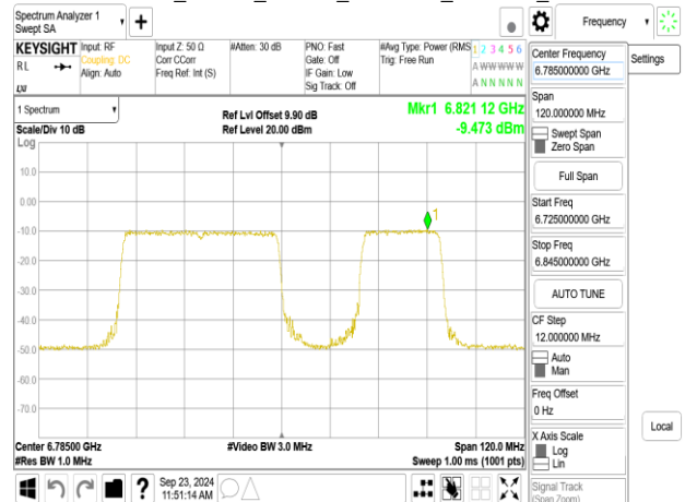
802.11be_80MHz_ChainB_6785MHz_RU484_66
