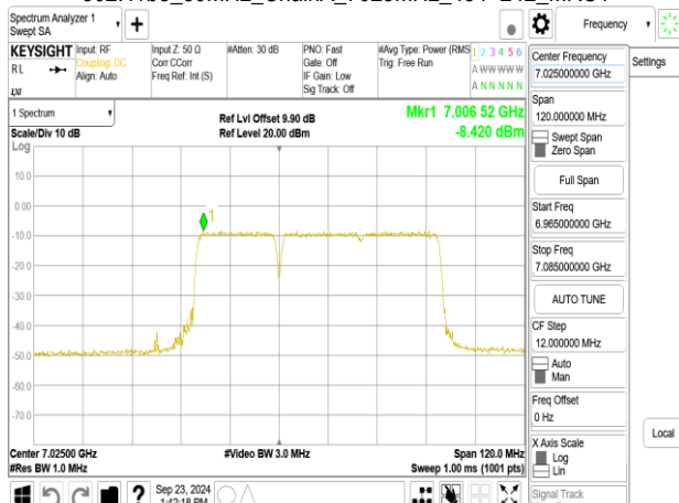
802.11be_80MHz_ChainA_7025MHz_484+242_MRU3
