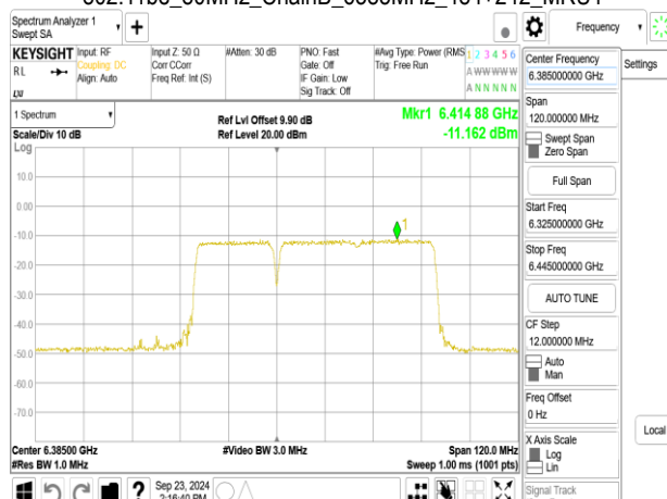
802.11be_80MHz_ChainB_6385MHz_484+242_MRU3
