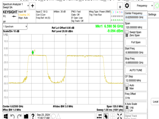
802.11be_80MHz_ChainB_6625MHz_484+242_MRU4
