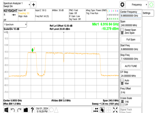
802.11be_160MHz_ChainA_6985MHz_996+484+242_MRU4
