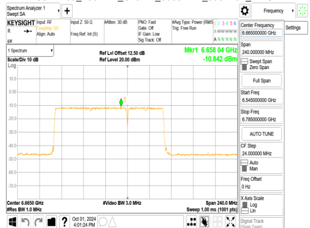
802.11be_160MHz_ChainA_6665MHz_RU996_67
