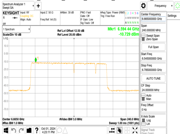
802.11be_160MHz_ChainA_6665MHz_996+484_MRU1
