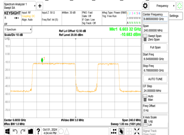
802.11be_160MHz_ChainA_6665MHz_996+484_MRU4
