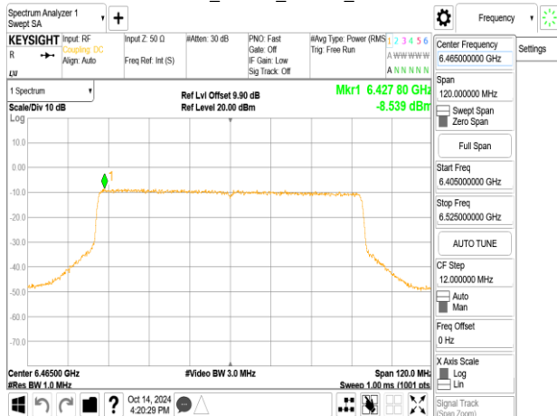
802.11be_80MHz_ChainB_6465MHz_484+242_MRU1
