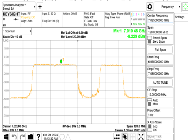
802.11be_80MHz_ChainB_7025MHz_RU484_66
