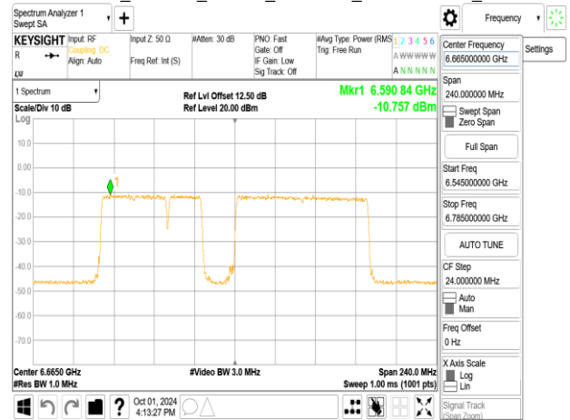
802.11be_160MHz_ChainA_6665MHz_996+484+242_MRU5
