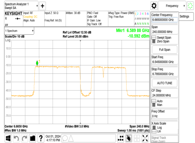
802.11be_160MHz_ChainA_6665MHz_996+484+242_MRU7
