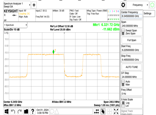
802.11be_160MHz_ChainA_6345MHz_RU996_S67
