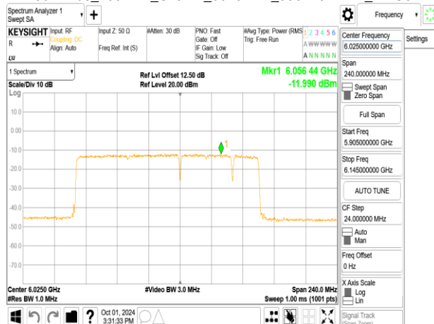
802.11be_160MHz_ChainA_6025MHz_996+484+242_MR08
