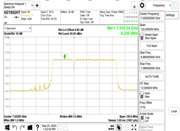
802.11be_80MHz_ChainB_7025MHz_484+242_MRU1
