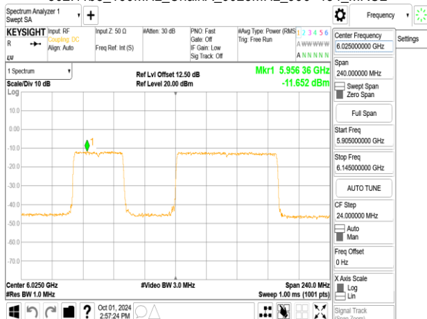
802.11be_160MHz_ChainA_6025MHz_996+484_MR04
