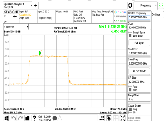
802.11be_80MHz_ChainB_6465MHz_RU484_65
