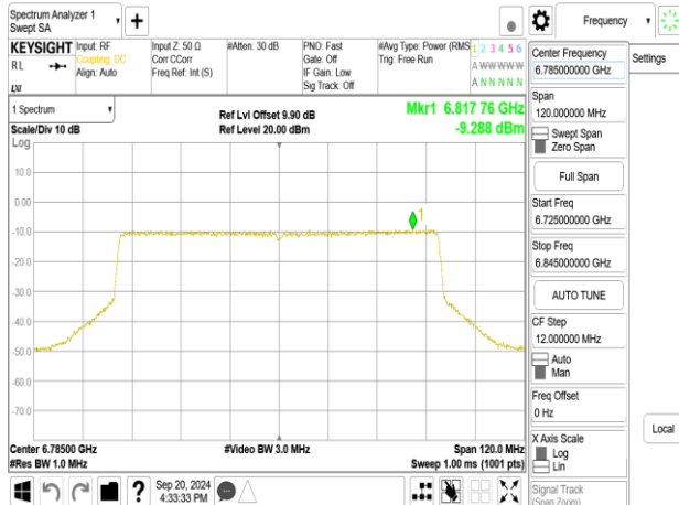
802.11be_80MHz_ChainB_6785MHz_484+242_MRU1
