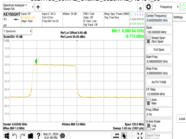
802.11be_80MHz_ChainB_6625MHz_RU484_65
