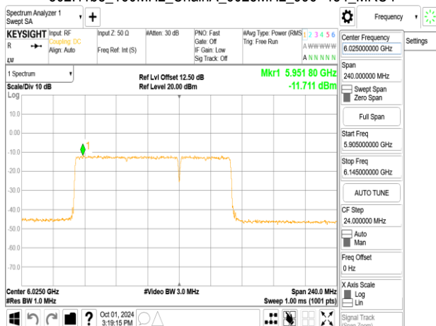
802.11be_160MHz_ChainA_6025MHz_RU996_67
