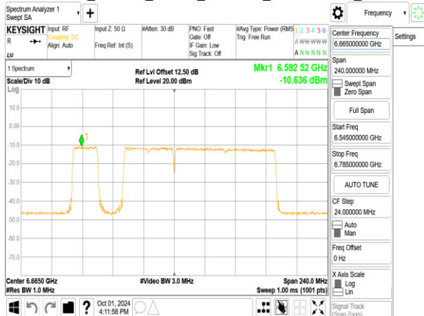
802.11be_160MHz_ChainA_6665MHz_996+484+242_MRU2
