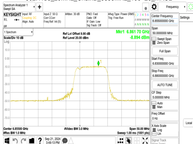
802.11be_20MHz_ChainB_6855MHz_52+26_MRU3
