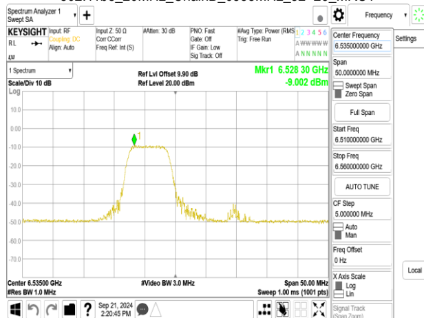
802.11be_20MHz_ChainB_6535MHz_RU106_53
