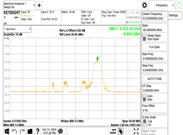
802.11be_20MHz_ChainB_6515MHz_RU26_8
