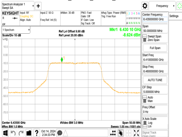
802.11be_20MHz_ChainB_6435MHz_106+26_MRU1
