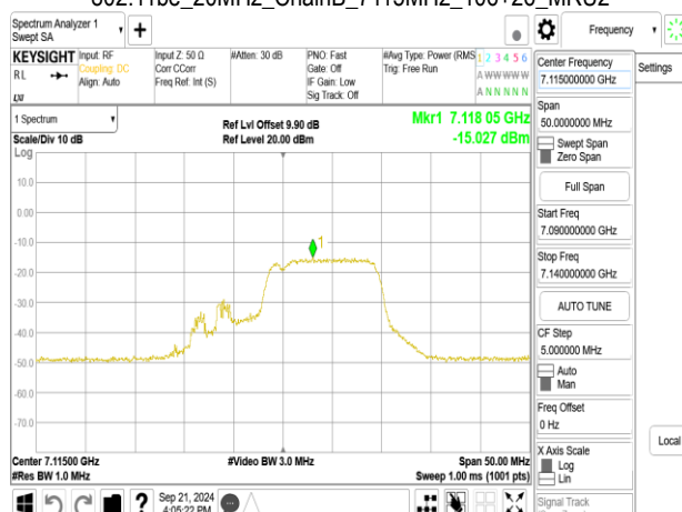
802.11be_20MHz_ChainB_7115MHz_106+26_MRU2
