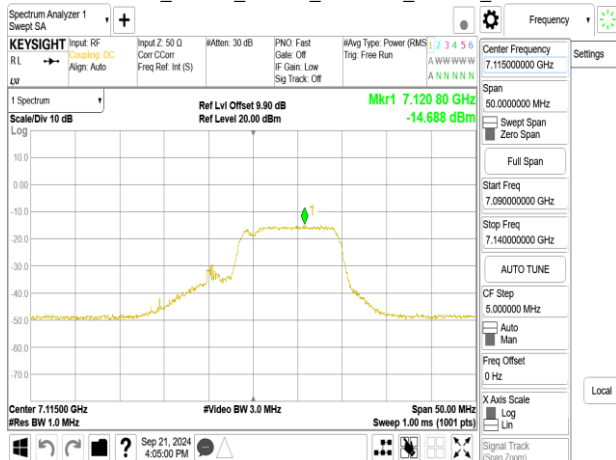
802.11be_20MHz_ChainA_7115MHz_52+26_MRU3
