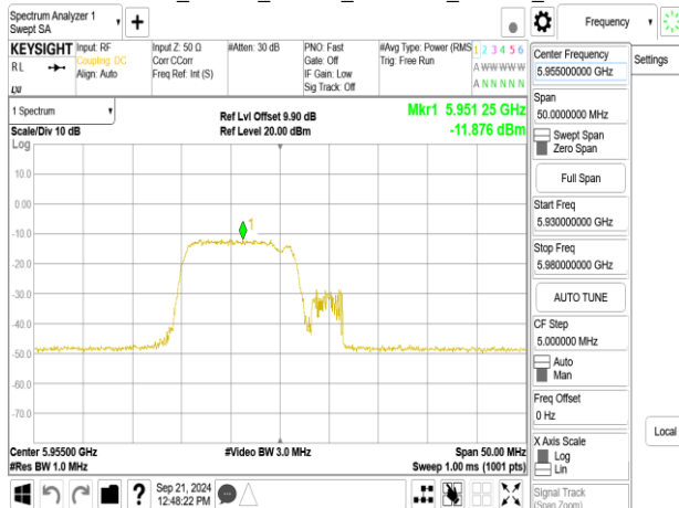
802.11be_20MHz_ChainB_5955MHz_52+26_MRUI
