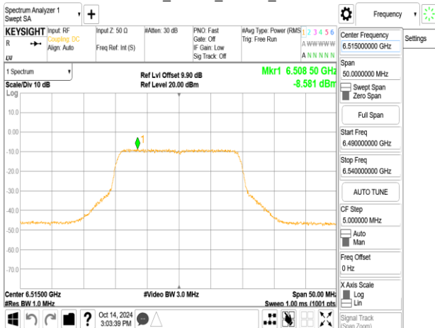
802.11be_20MHz_ChainB_6515MHz_106+26_MRUI2
