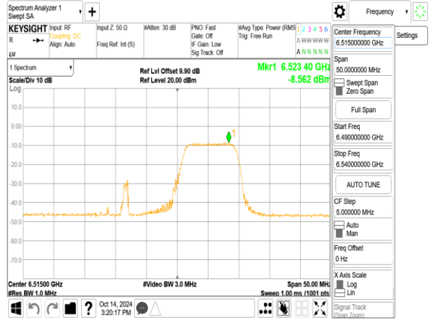
802.11be_20MHz_ChainB_6515MHz_RU26_8
