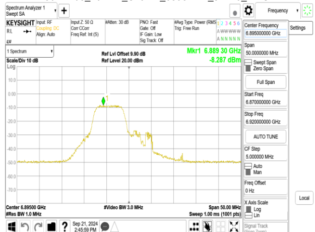
802.11be_20MHz_ChainB_6895MHz_52+26_MRUI
