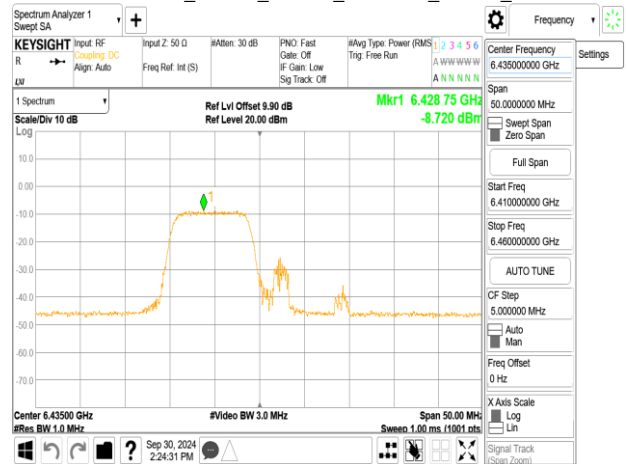
802.11be_20MHz_ChainB_6435MHz_RU26_0
