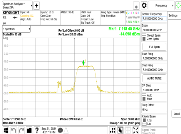
802.11be_20MHz_ChainA_7115MHz_RU106_54
