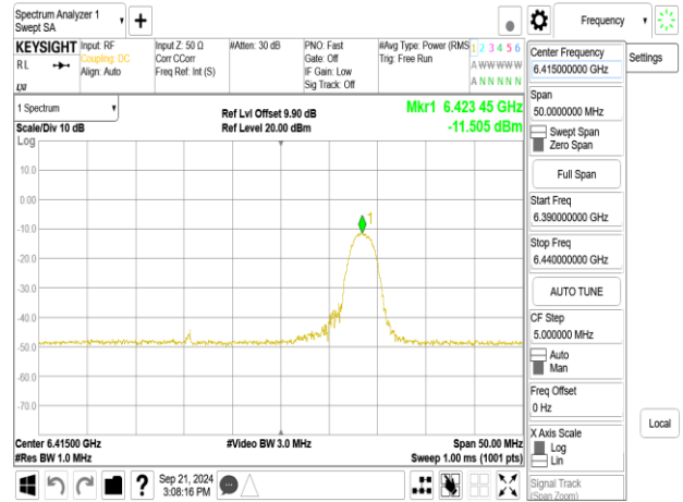
802.11be_20MHz_ChainB_6415MHz_RU52_40
