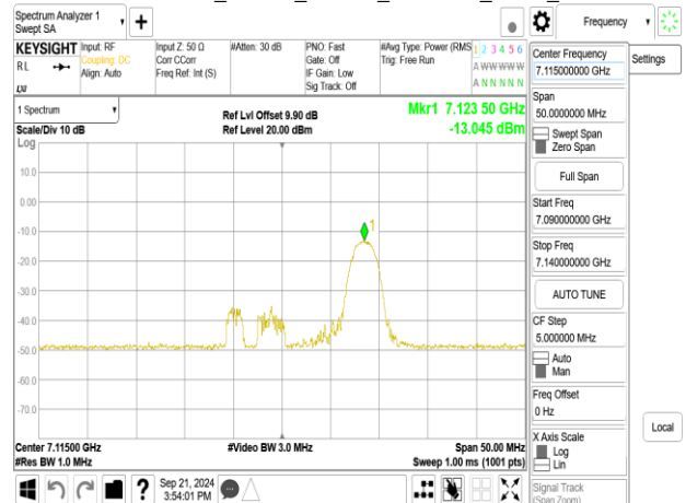
802.11be_20MHz_ChainA_7115MHz_RU52_40
