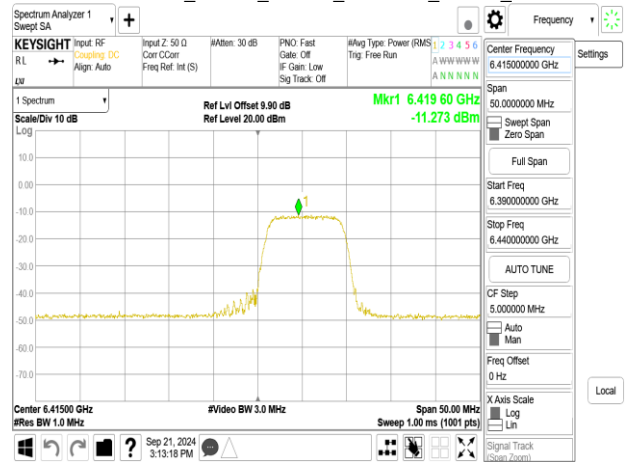
802.11be_20MHz_ChainB_6415MHz_RU26_8
