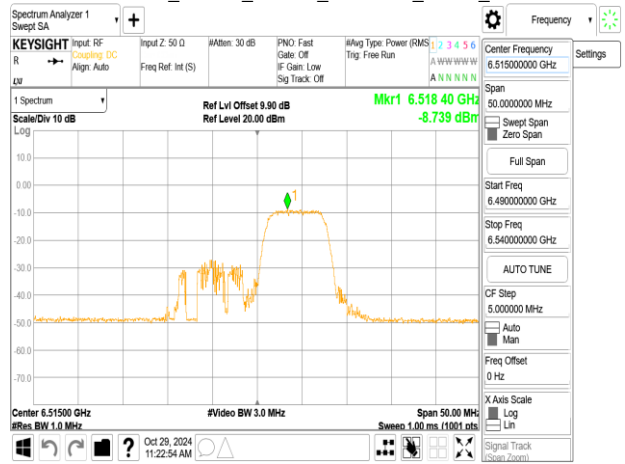
802.11be_20MHz_ChainB_6515MHz_RU106_54
