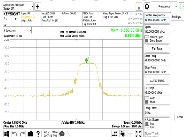
802.11be_20MHz_ChainB_6855MHz_RU106_54
