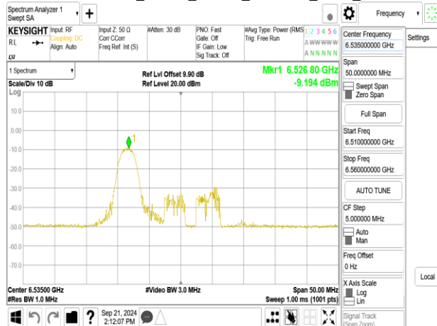
802.11be_20MHz_ChainB_6535MHz_RU26_0
