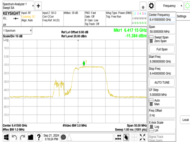
802.11be_20MHz_ChainB_6415MHz_52+26_MRU3
