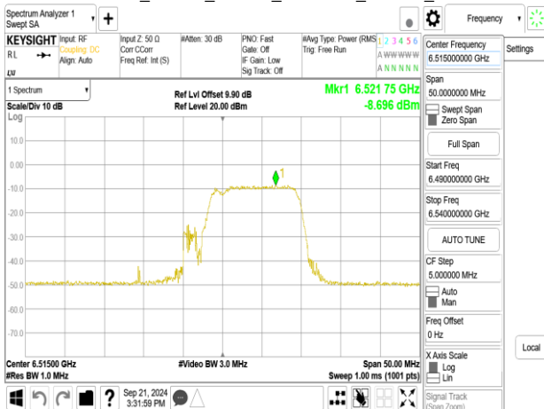
802.11be_20MHz_ChainB_6515MHz_106+26_MRUI2
