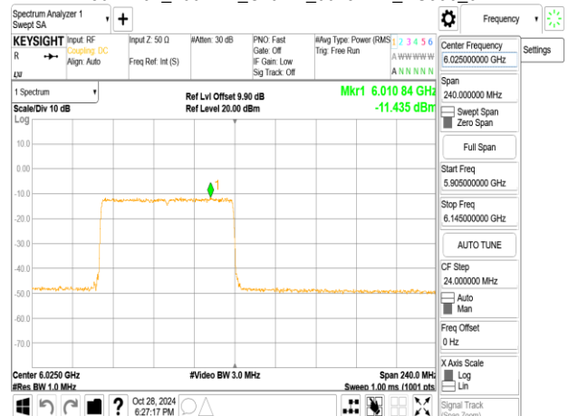
802.11ax_160MHz_ChainA_6025MHz_RU996_67
