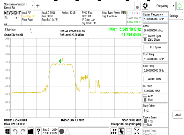
802.11be_20MHz_ChainA_5955MHz_RU26_0
