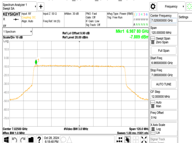
802.11ax_80MHz_ChainB_7025MHz
