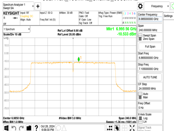
802.11ax_160MHz_ChainB_6985MHz_RU996_67
