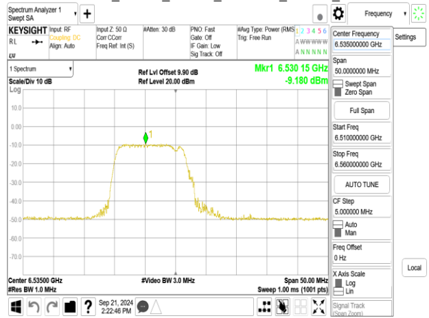
802.11be_20MHz_ChainA_6535MHz_52+26_MRUI
