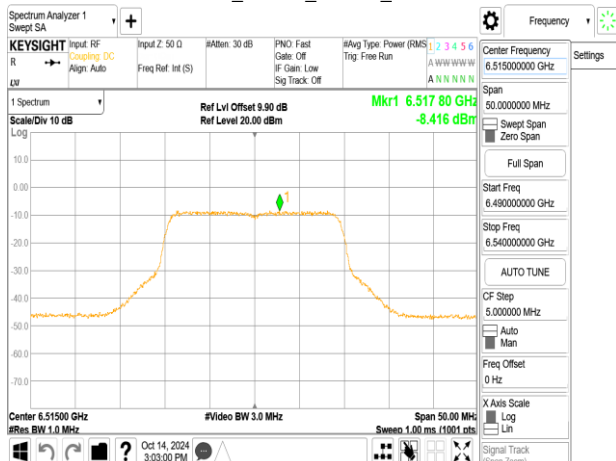
802.11be_20MHz_ChainA_6515MHz
