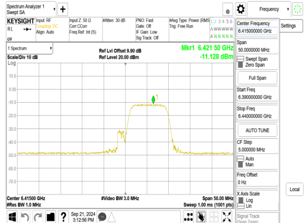
802.11be_20MHz_ChainA_6415MHz_RU26_8
