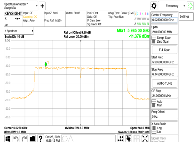
802.11ax_160MHz_ChainB_6025MHz
