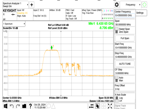
802.11be_20MHz_ChainA_6435MHz_RU106_53
