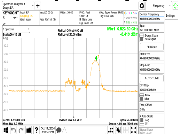
802.11be_20MHz_ChainA_6515MHz_RU52_40
