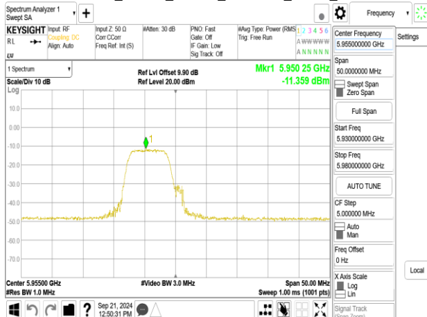
802.11be_20MHz_ChainA_5955MHz_52+26_MRU1
