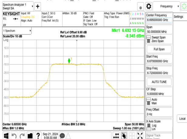
802.11be_20MHz_ChainA_6695MHz
