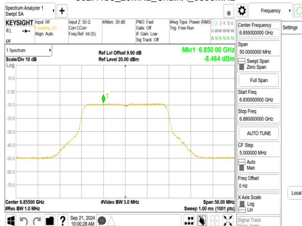
802.11be_20MHz_ChainA_6855MHz_106+26_MRU2
