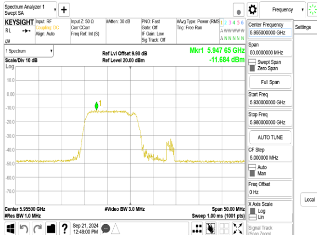
802.11be_20MHz_ChainA_5955MHz_52+26_MRU1
