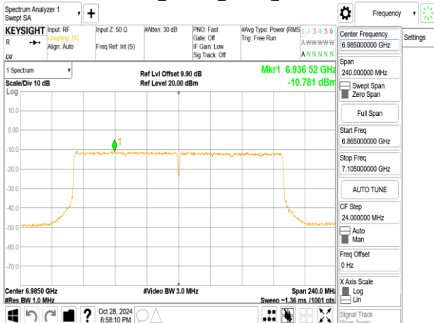
802.11ax_160MHz_ChainA_6985MHz
