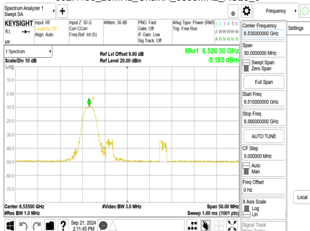
802.11be_20MHz_ChainA_6535MHz_RU52_37
