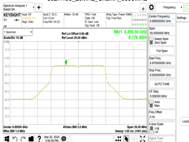
802.11be_20MHz_ChainA_6895MHz_106+26_MRU1
