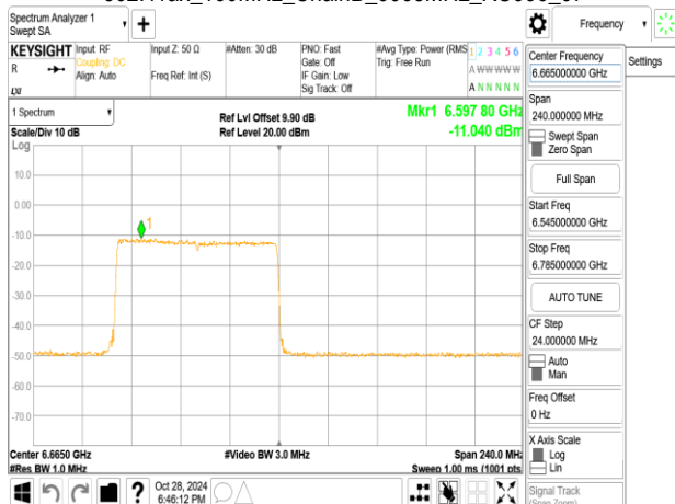
802.11ax_160MHz_ChainB_6665MHz_RU996_S67
