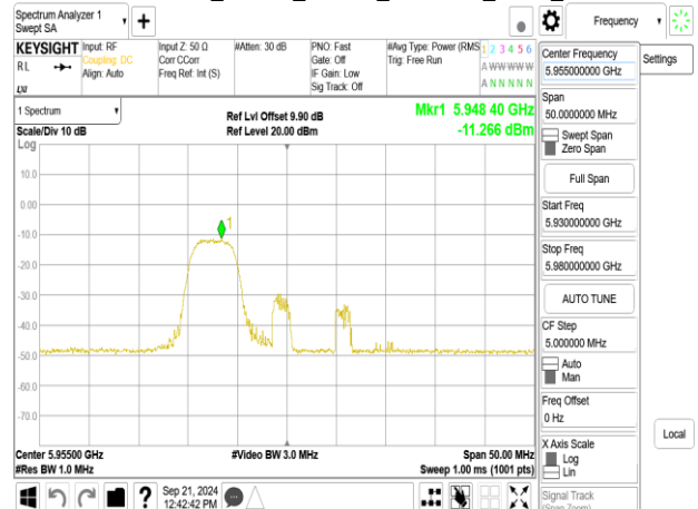
802.11be_20MHz_ChainA_5955MHz_RU52_37
