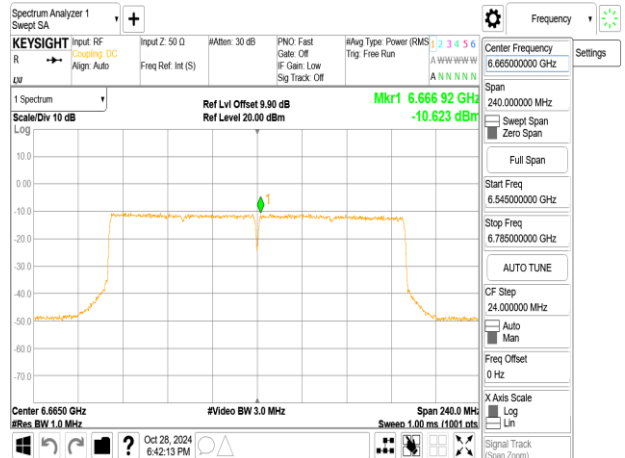
802.11ax_160MHz_ChainA_6665MHz_RU996_67
