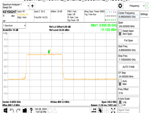
802.11ax_160MHz_ChainB_6985MHz_RU996_S67
