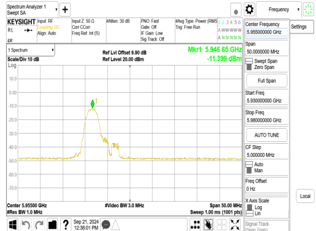
802.11be_20MHz_ChainA_5955MHz_RU52_37
