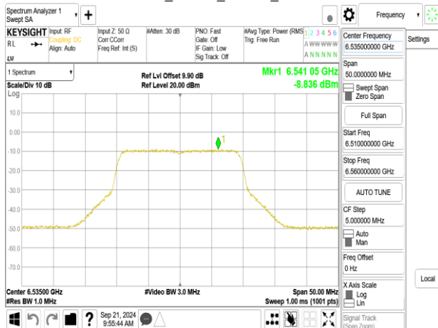
802.11be_20MHz_ChainA_6535MHz
