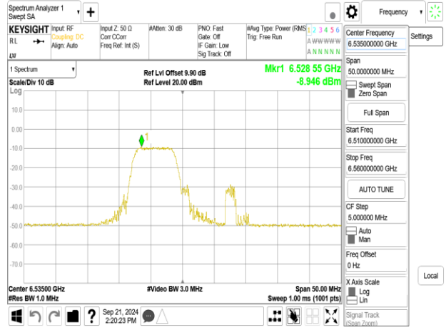
802.11be_20MHz_ChainA_6535MHz_RU106_53
