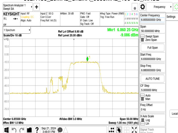
802.11be_20MHz_ChainA_6855MHz_52+26_MRU3
