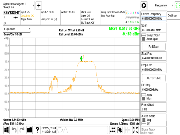
802.11be_20MHz_ChainA_6515MHz_RU106_54
