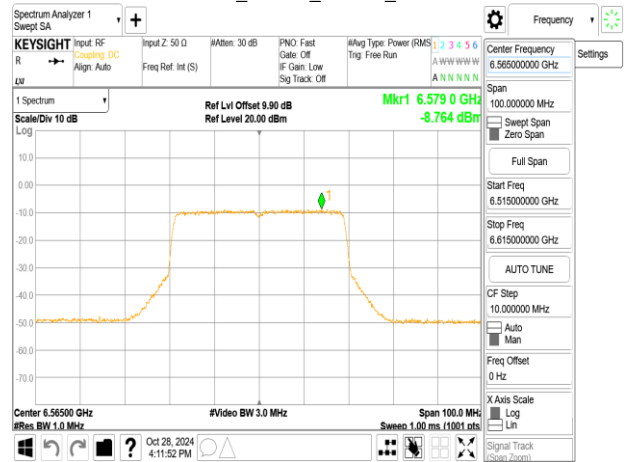
802.11ax_40MHz_ChainB_6565MHz_RU242_61
