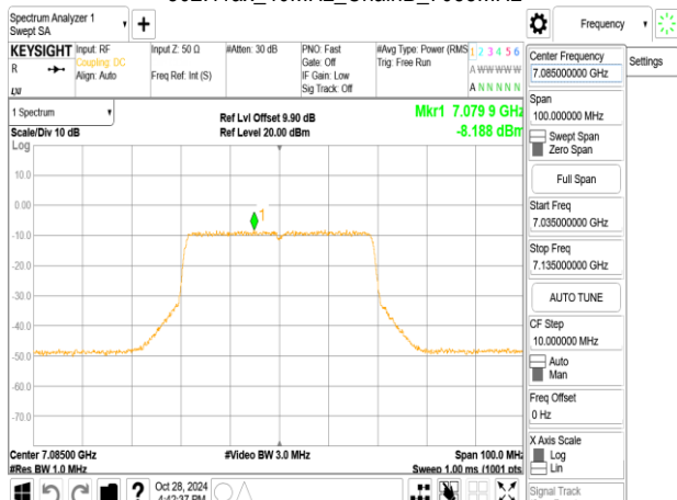
802.11ax_40MHz_ChainB_7085MHz_RU242_62
