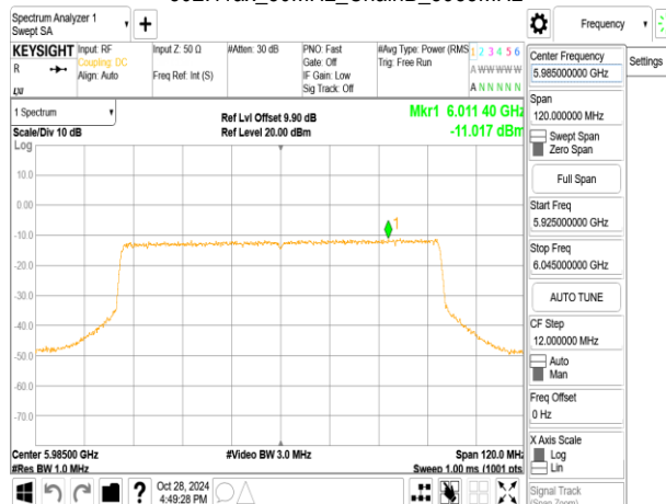
802.11ax_80MHz_ChainB_5985MHz_RU484_65
