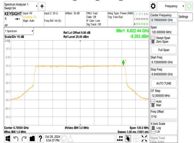
802.11ax_80MHz_ChainB_6785MHz_RU484_66
