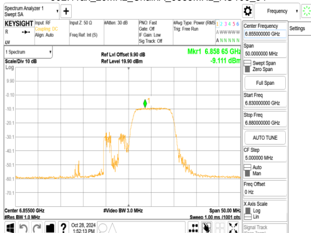
802.11ax_20MHz_ChainA_6855MHz_RU26_8
