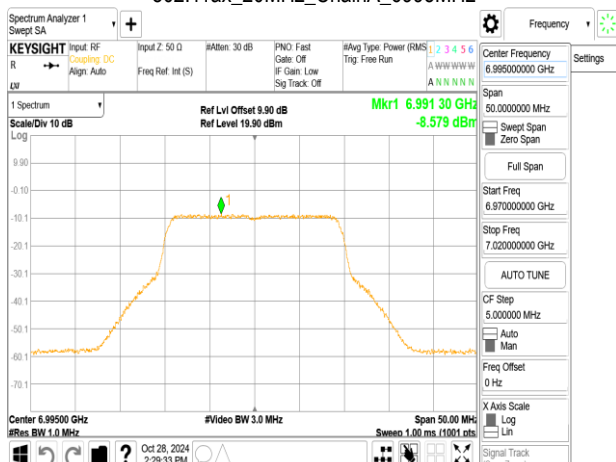
802.11ax_20MHz_ChainA_6995MHz
