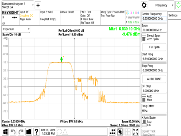
802.11ax_20MHz_ChainA_6535MHz_RU26_0
