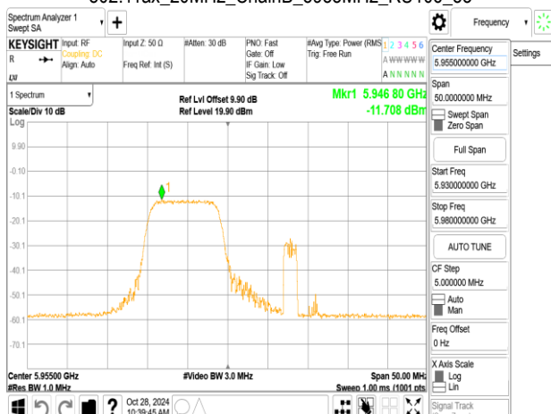
802.11ax_20MHz_ChainB_5955MHz_RU106_53
