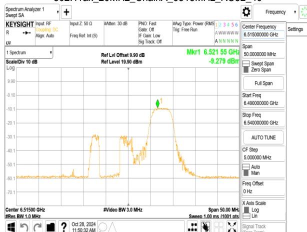
802.11ax_20MHz_ChainA_6515MHz_RU52_40
