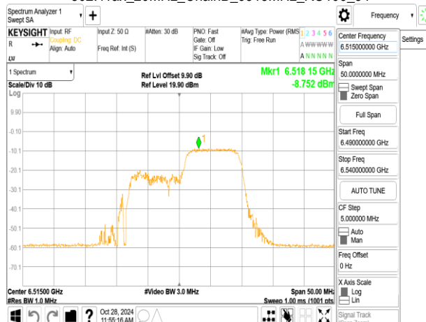
802.11ax_20MHz_ChainB_6515MHz_RU26_8
