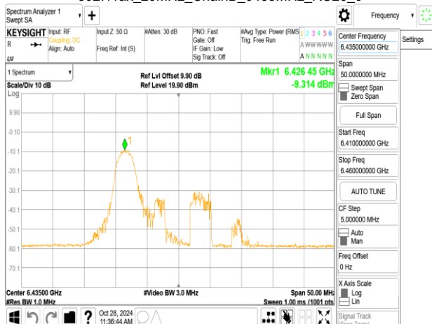
802.11ax_20MHz_ChainB_6435MHz_RU52_37
