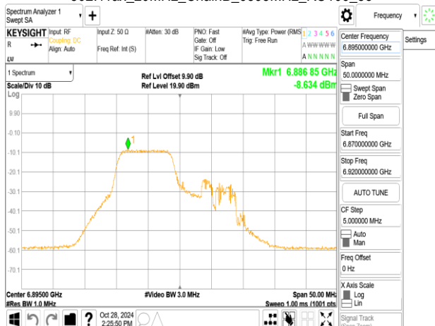
802.11ax_20MHz_ChainB_6895MHz_RU26_0
