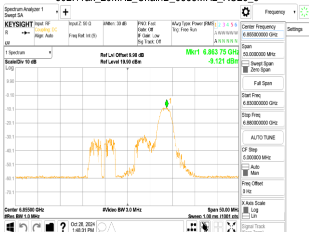
802.11ax_20MHz_ChainB_6855MHz_RU26_8
