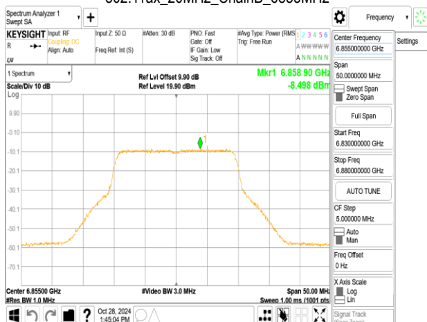
802.11ax_20MHz_ChainB_6855MHz_RU106_54
