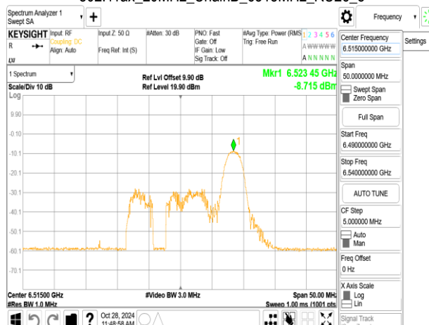
802.11ax_20MHz_ChainB_6515MHz_RU26_8
