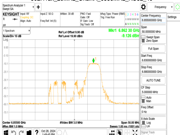
802.11ax_20MHz_ChainA_6855MHz_RU52_40
