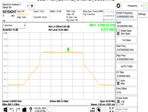
802.11ax_20MHz_ChainB_6895MHz
