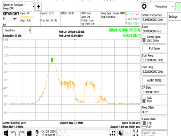
802.11ax_20MHz_ChainA_6895MHz_RU52_37
