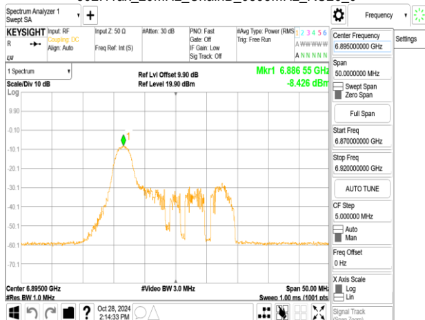
802.11ax_20MHz_ChainB_6895MHz_RU52_37
